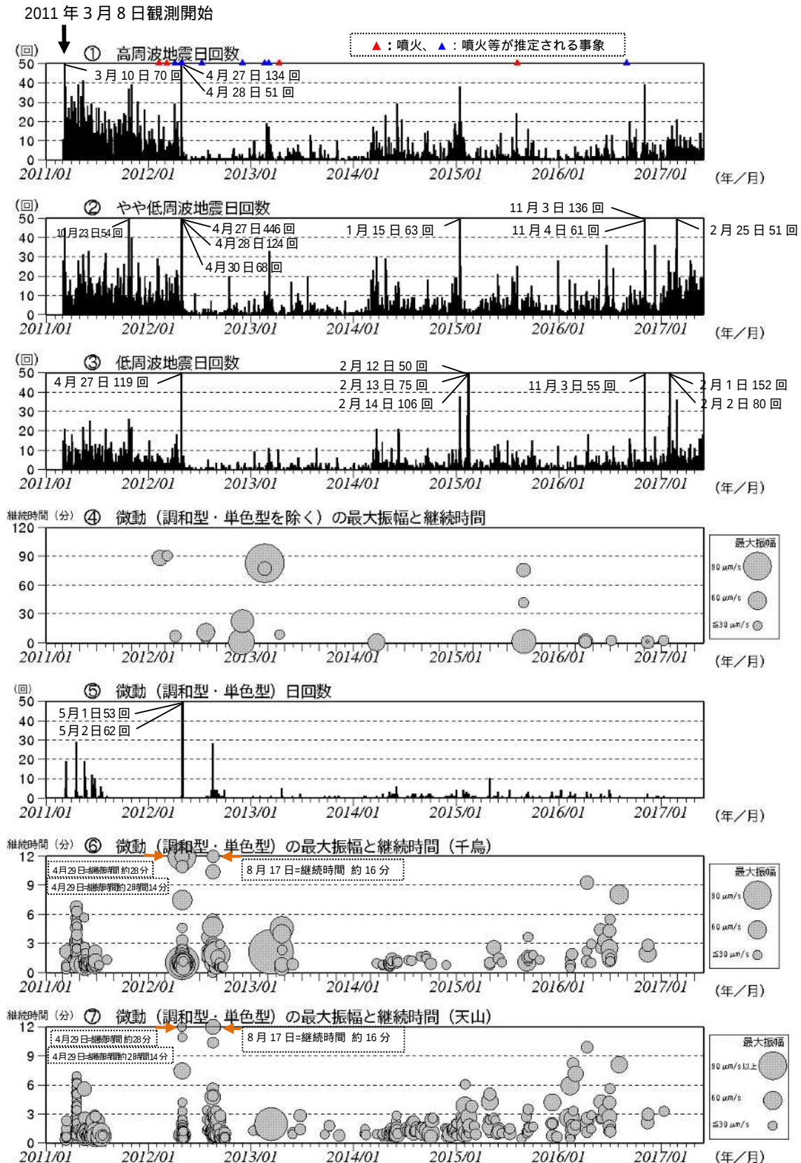
図4 硫黄島 火山活動経過図（2011年3月8日～2017年5月31日）
