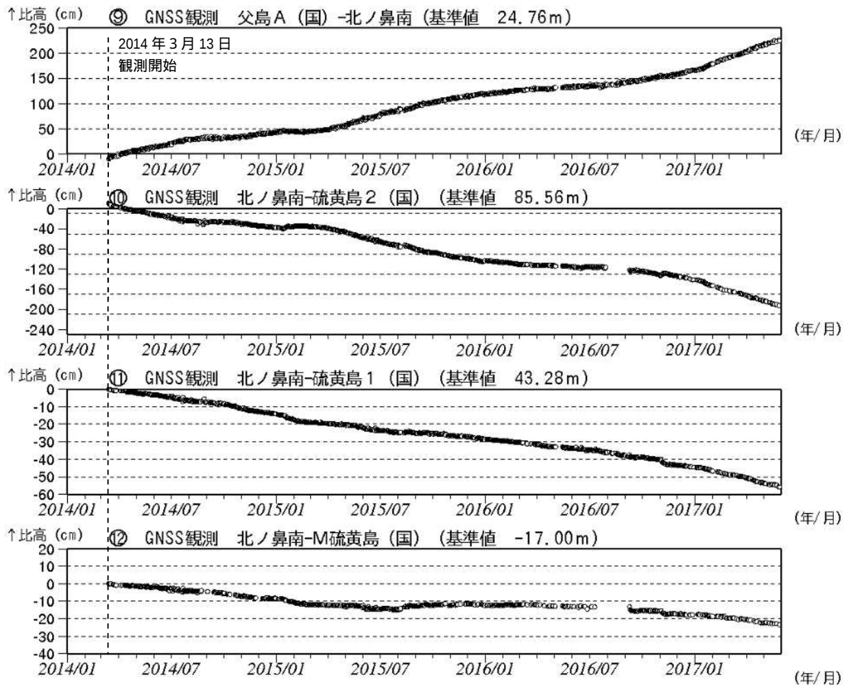
図6 硫黄島 GNSS 観測結果（2014 年 3 月 13 日～2017 年 5 月 31 日）（国）：国土地理院
