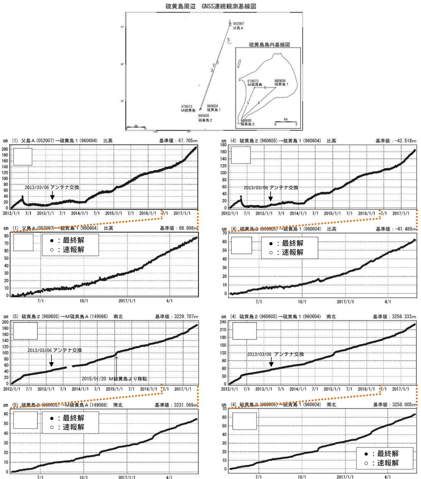
図 5 硫黄島 国土地理院による地殻変動観測結果 3)
