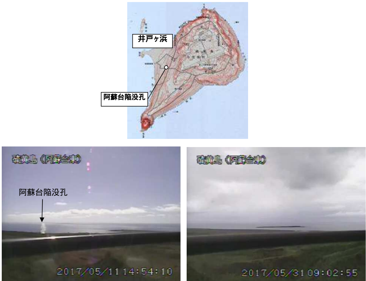
図2 硫黄島 海岸付近の噴気の状態、阿蘇台東監視カメラによる
