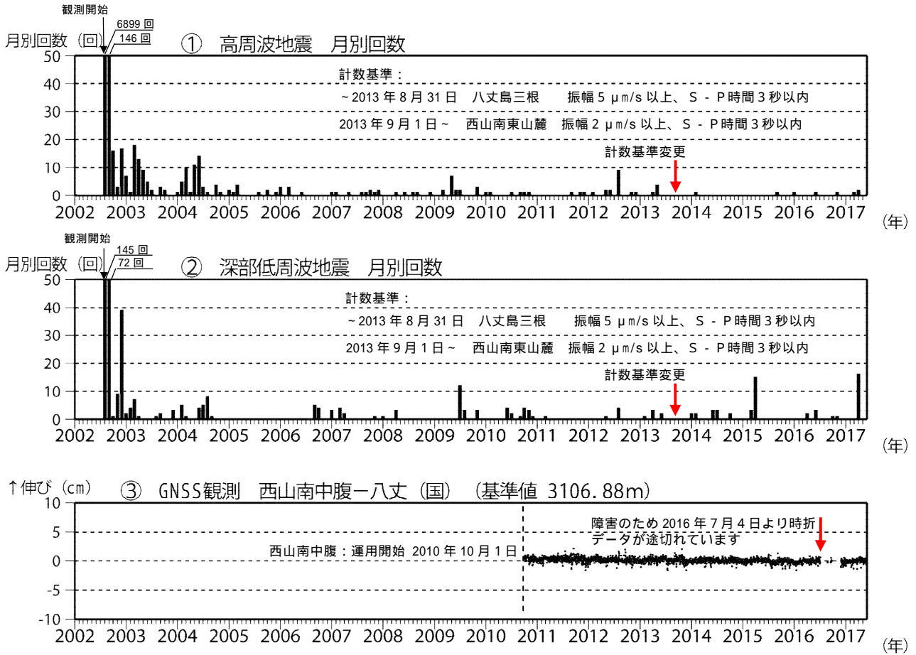
図2 八丈島 火山活動経過図(2002年8月13日~2017年5月31日)
