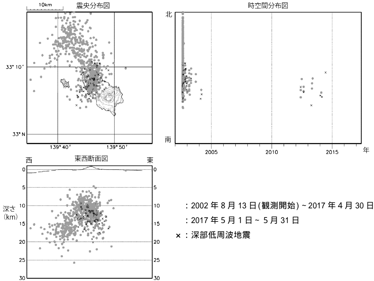
図3 八丈島 震源分布図(2002年8月13日~2017年5月31日) ・今期間、八丈島付近に震源が求まる高周波地震及び深部低周波地震はありませんでした。
