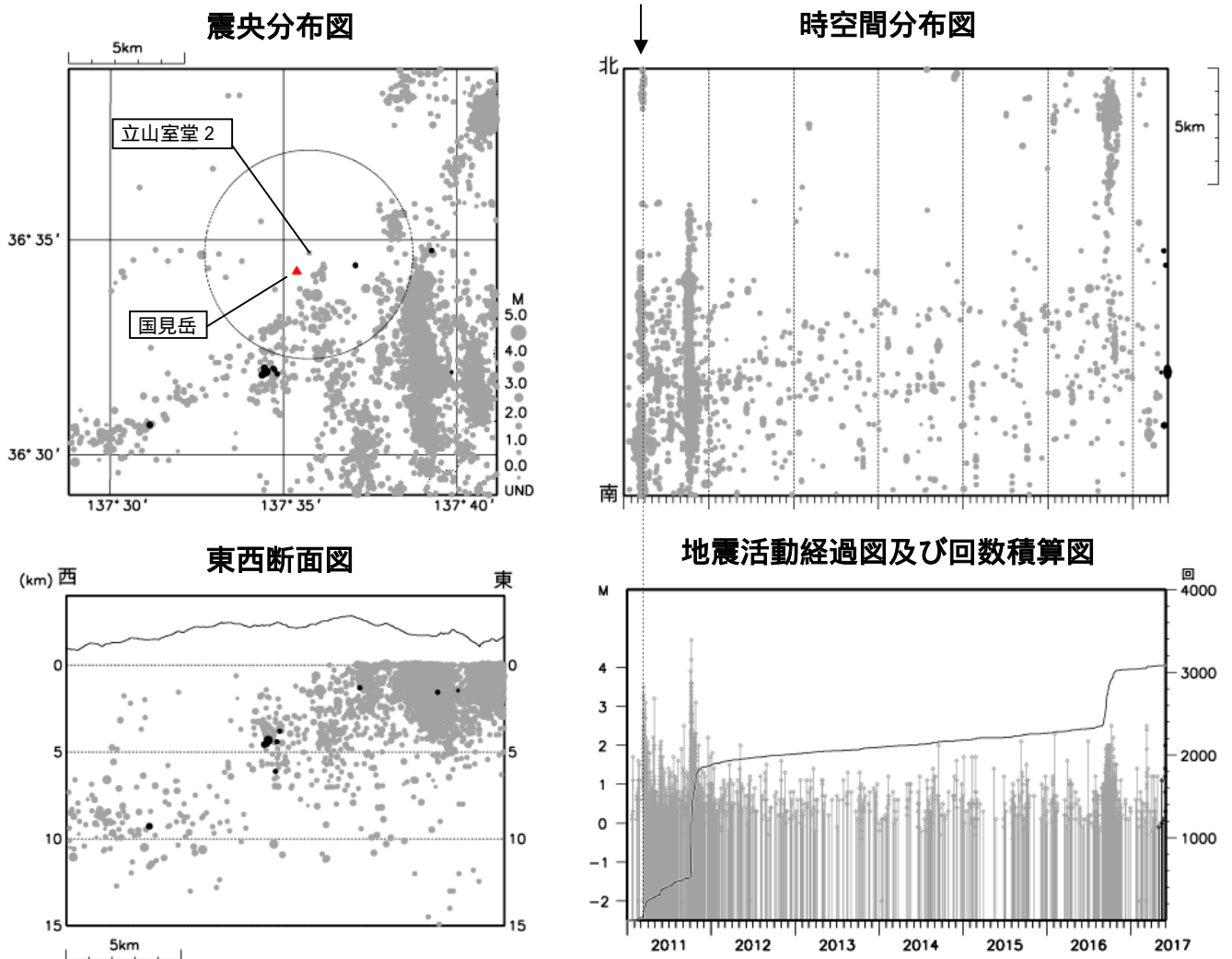
図 2 弥陀ヶ原 広域地震観測網による山体・周辺の地震活動（2011 年 1 月 1 日～2017 年 5 月 31 日） : 2011 年 1 月 1 日～2017 年 4 月 30 日 : 2017 年 5 月 1 日～5 月 31 日
