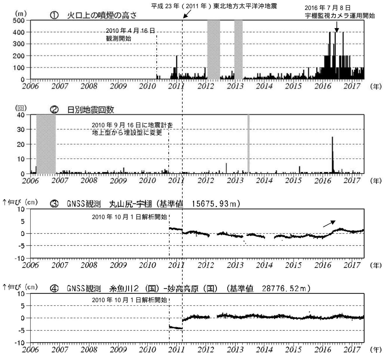
図3 新潟焼山 火山活動経過図(2006年1月1日~2017年5月31日)
