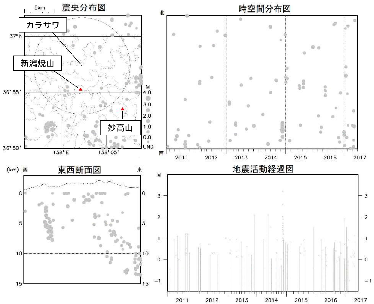
図8 新潟焼山 広域地震観測網による山体周辺の地震活動(2011年1月1日~2017年5月31日) : 2011年1月1日~2017年4月30日 : 2017年5月1日~5月31日
