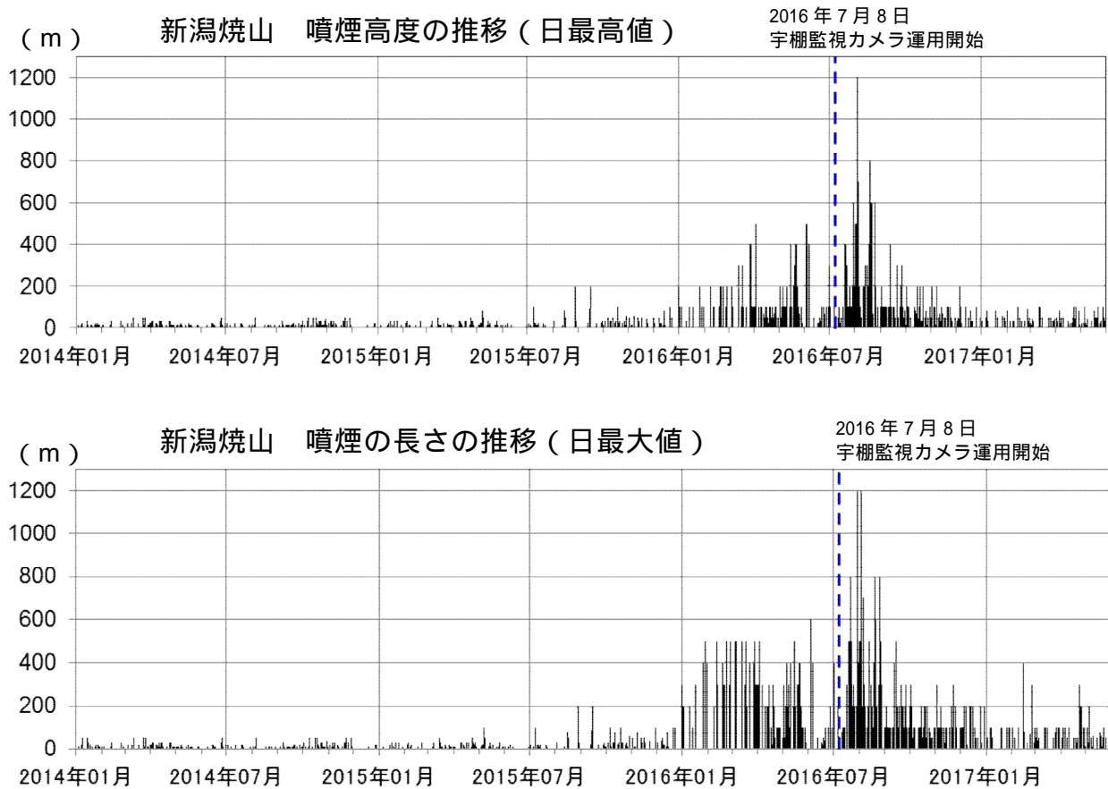
図4 新潟焼山 噴煙高度と噴煙の長さの推移 （それぞれ日最高値及び日最大値、2014年1月1日～2017年5月31日）
