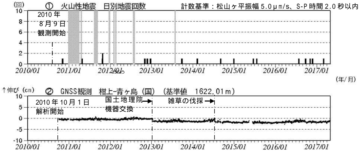
図2 青ヶ島 火山活動経過図（2010年8月9日～2017年4月30日）（年/月） 青ヶ島周辺の日別地震回数 グラフの灰色部分は機器障害による欠測。 GNSS連続観測による基線長変化（国）：国土地理院 は図3のGNSS基線に対応。グラフの空白部分は欠測。 ・2014年7月15日に実施した雑草の伐採の影響により、ステップ状の変化がみられます。
