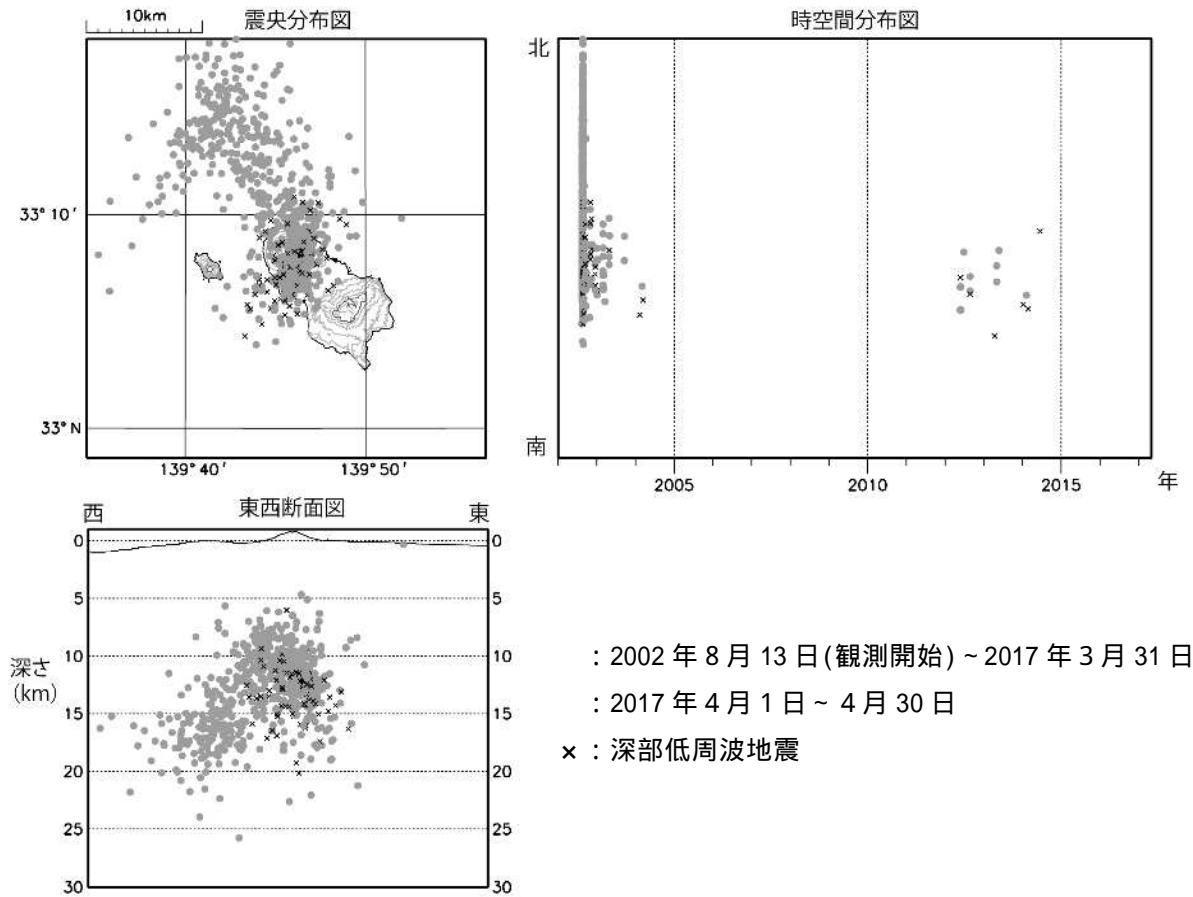
図3 八丈島 震源分布図(2002年8月13日~2017年4月30日) ・今期間、八丈島付近に震源が求まる高周波地震及び深部低周波地震はありませんでした。
