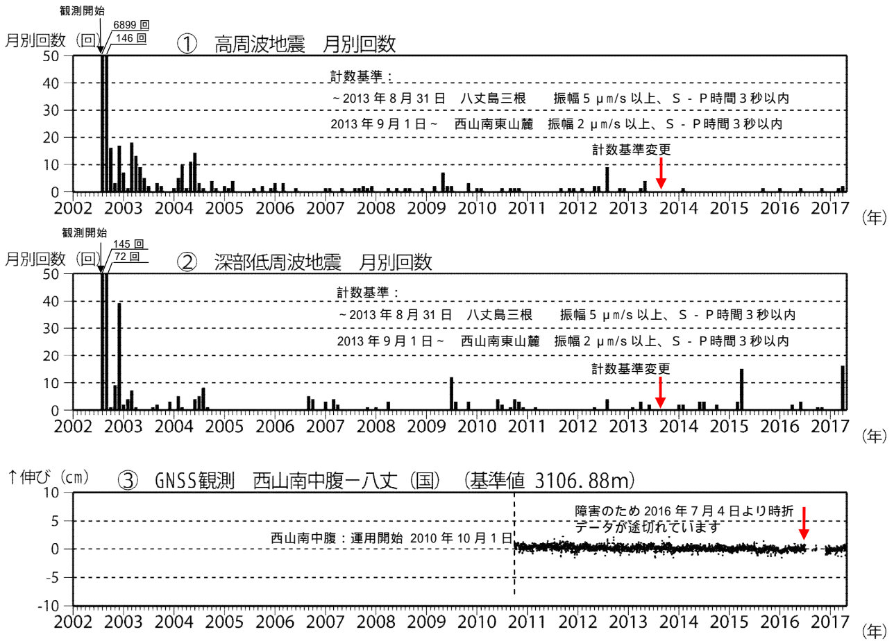
図2 八丈島 火山活動経過図(2002年8月13日~2017年4月30日)
