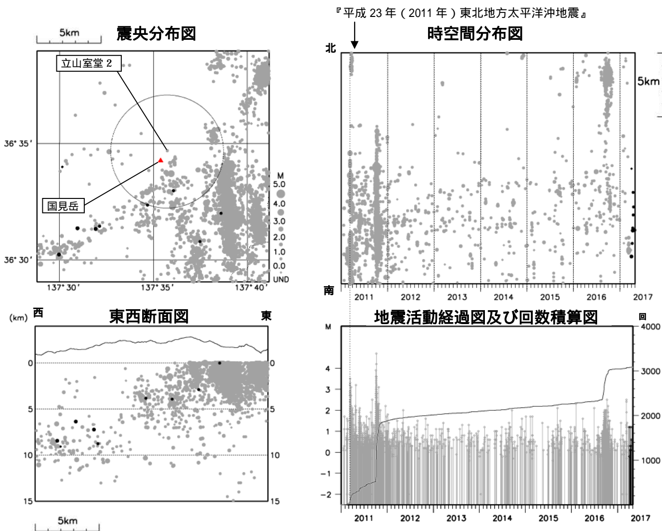
図 2 弥陀ヶ原 広域地震観測網による山体・周辺の地震活動 (2011 年 1 月 1 日 ~ 2017 年 4 月 30 日) : 2011 年 1 月 1 日 ~ 2017 年 3 月 31 日 : 2017 年 4 月 1 日 ~ 4 月 30 日
