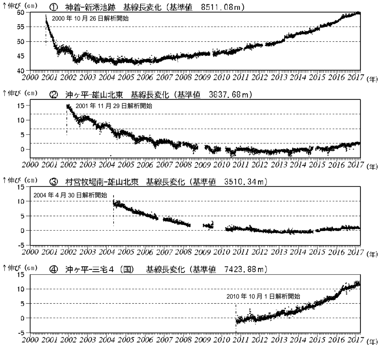
図9 三宅島 GNSS 連続観測結果 (2000年10月26日~2017年3月31日)
