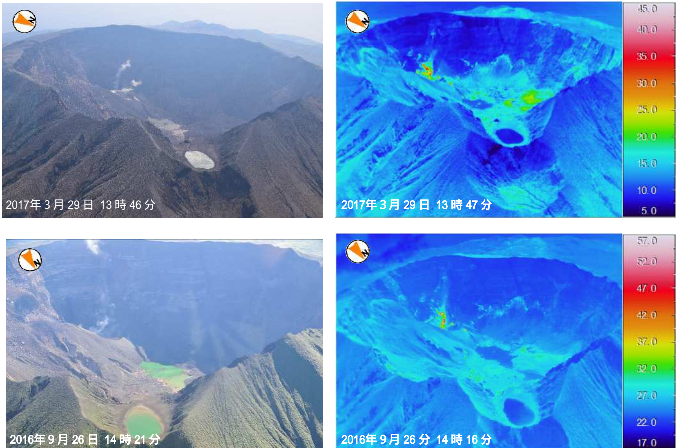
図5 三宅島 山頂火口の様子と赤外熱映像装置によるその地表面温度分布（陸上自衛隊の協力による） 上段：天気：晴れ 気温：12.4 （高度約 1200mより撮影） 下段：天気：曇り 気温：19.1 （高度約 1200mより撮影）
