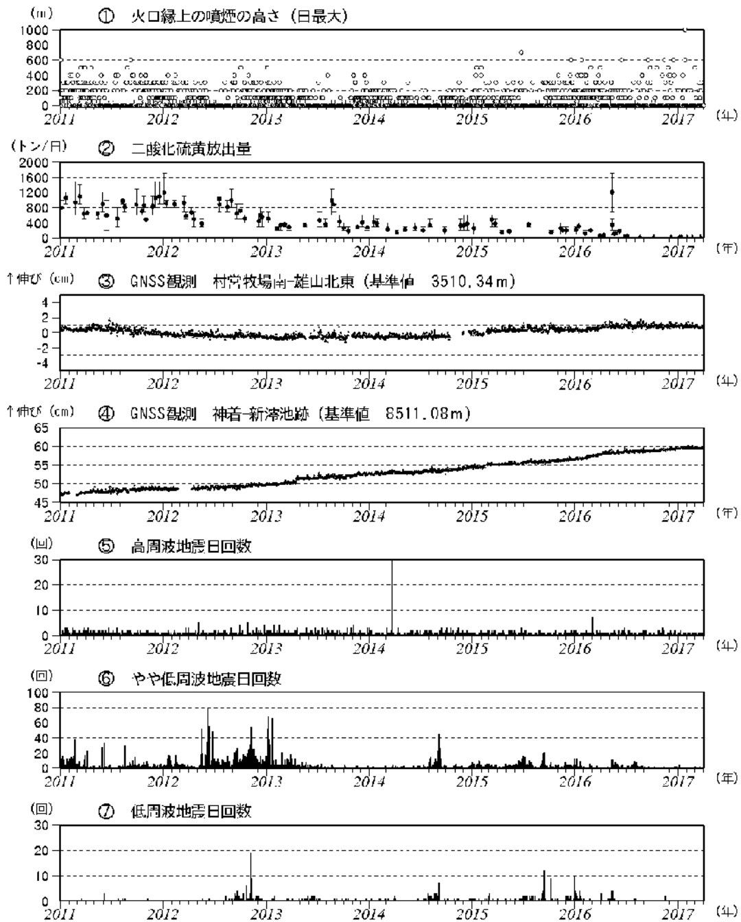
図 8 三宅島 火山活動短期経過図（2011 年 1 月 1 日～2017 年 3 月 31 日）
