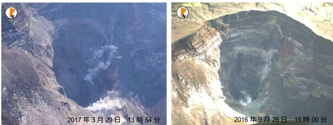
図6 三宅島 主火孔内の状況（左：2017年3月29日、右：2016年9月26日、いずれも陸上自衛隊の協力による） ・前回の観測（2016年9月26日）と比べて、主火孔内の地形等に特段の変化は認められません。
