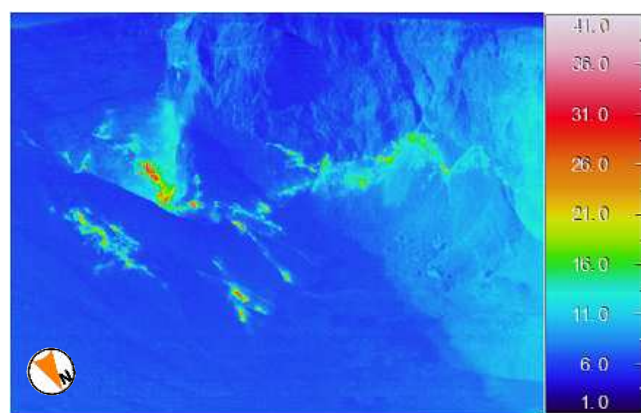
図 4 三宅島 赤外熱映像装置による山頂火口内の地表面温度分布
