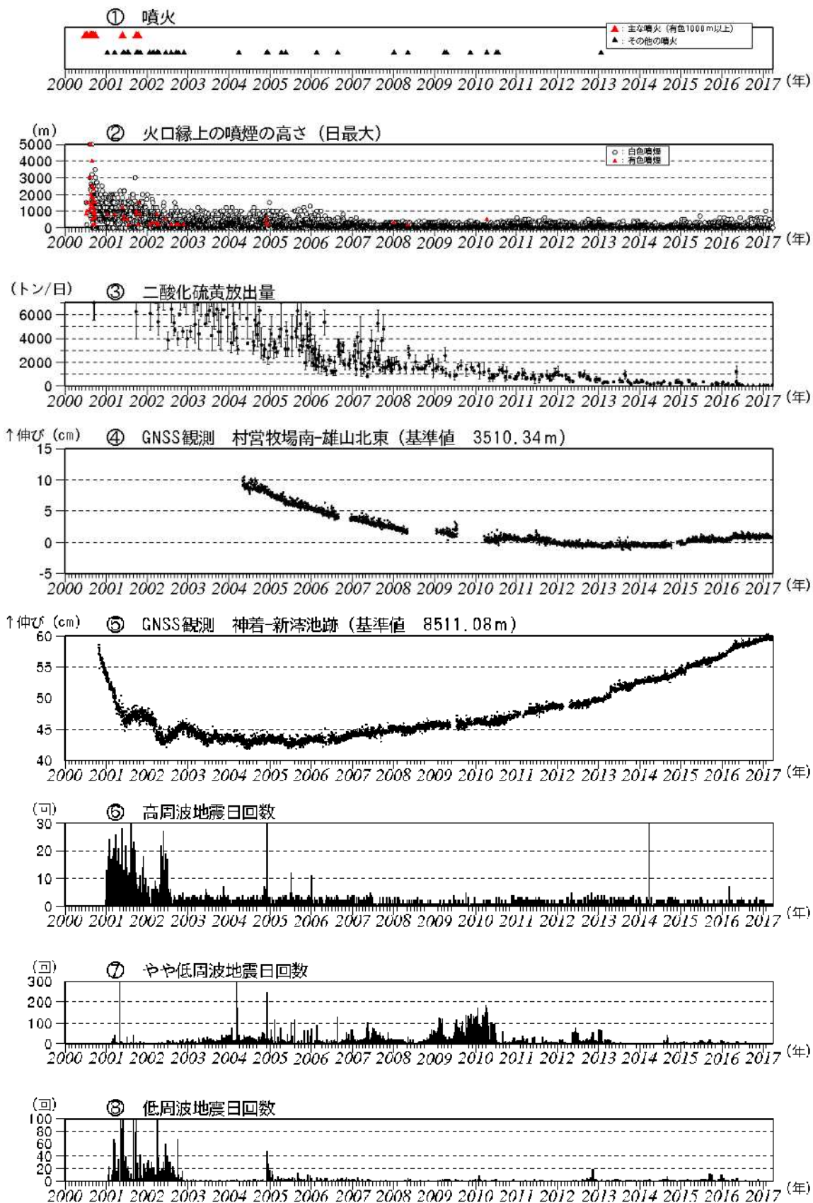
図7 三宅島 火山活動長期経過図 (2000年1月1日~2017年3月31日)
