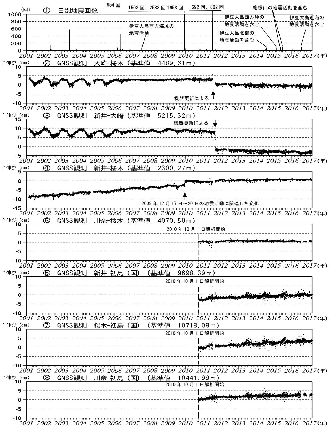
図3 伊豆東部火山群 火山活動経過図（2001年1月1日～2017年2月28日）
