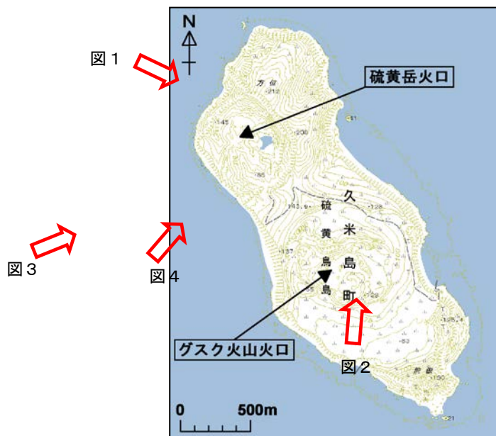
図 5 硫黄島 火口位置図と各図の撮影方向
