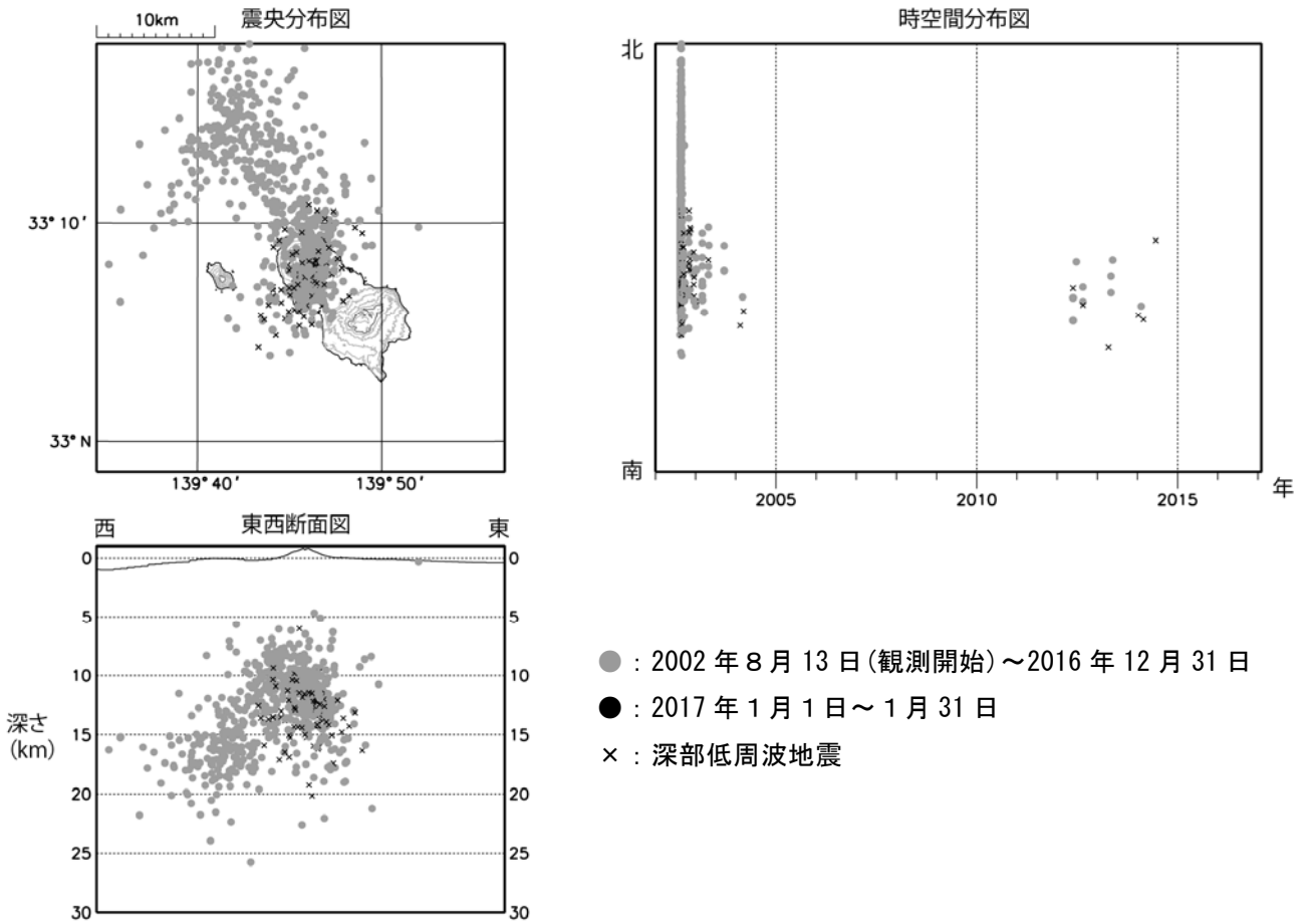
図 3 八丈島 震源分布図 (2002 年 8 月 13 日~2017 年 1 月 31 日) ・今期間、八丈島付近に震源が求まる高周波地震及び深部低周波地震はありませんでした。
