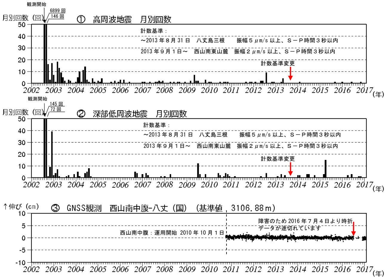
図2 八丈島 火山活動経過図 (2002年8月13日~2017年1月31日)
