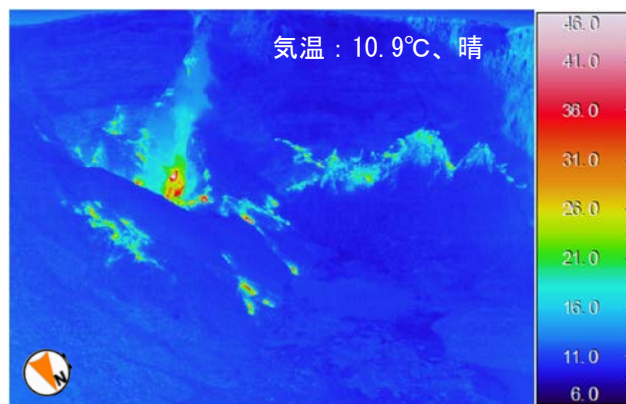
図 3 三宅島 赤外熱映像装置による山頂火口内の地表面温度分布 (1月22日)
