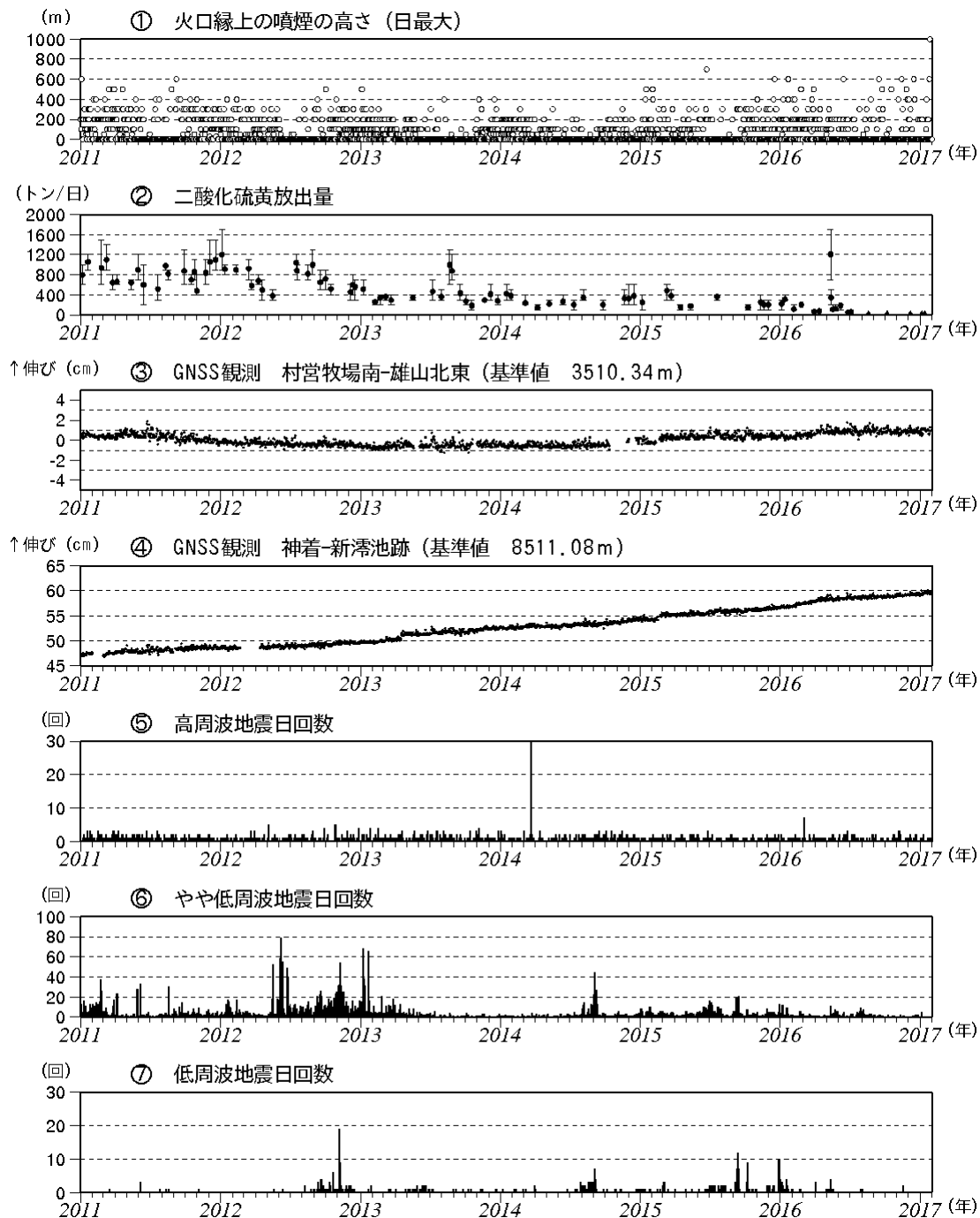
図5 三宅島 火山活動短期経過図（2011年1月1日～2017年1月31日）
