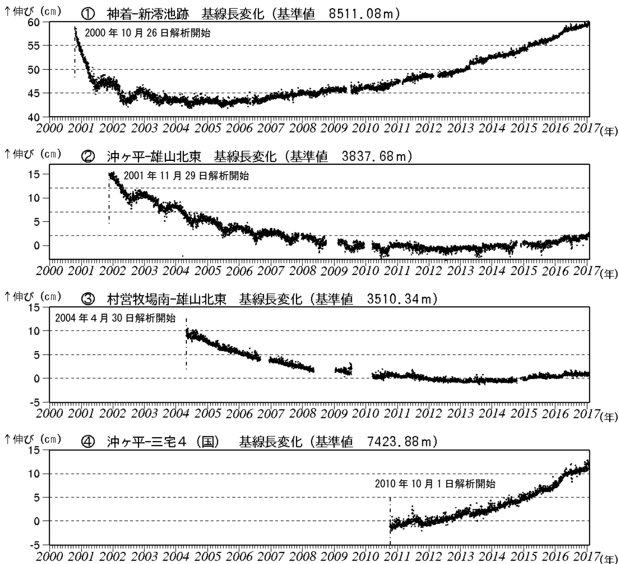
図6 三宅島 GNSS 連続観測結果 (2000年10月26日~2017年1月31日) (国): 国土地理院
