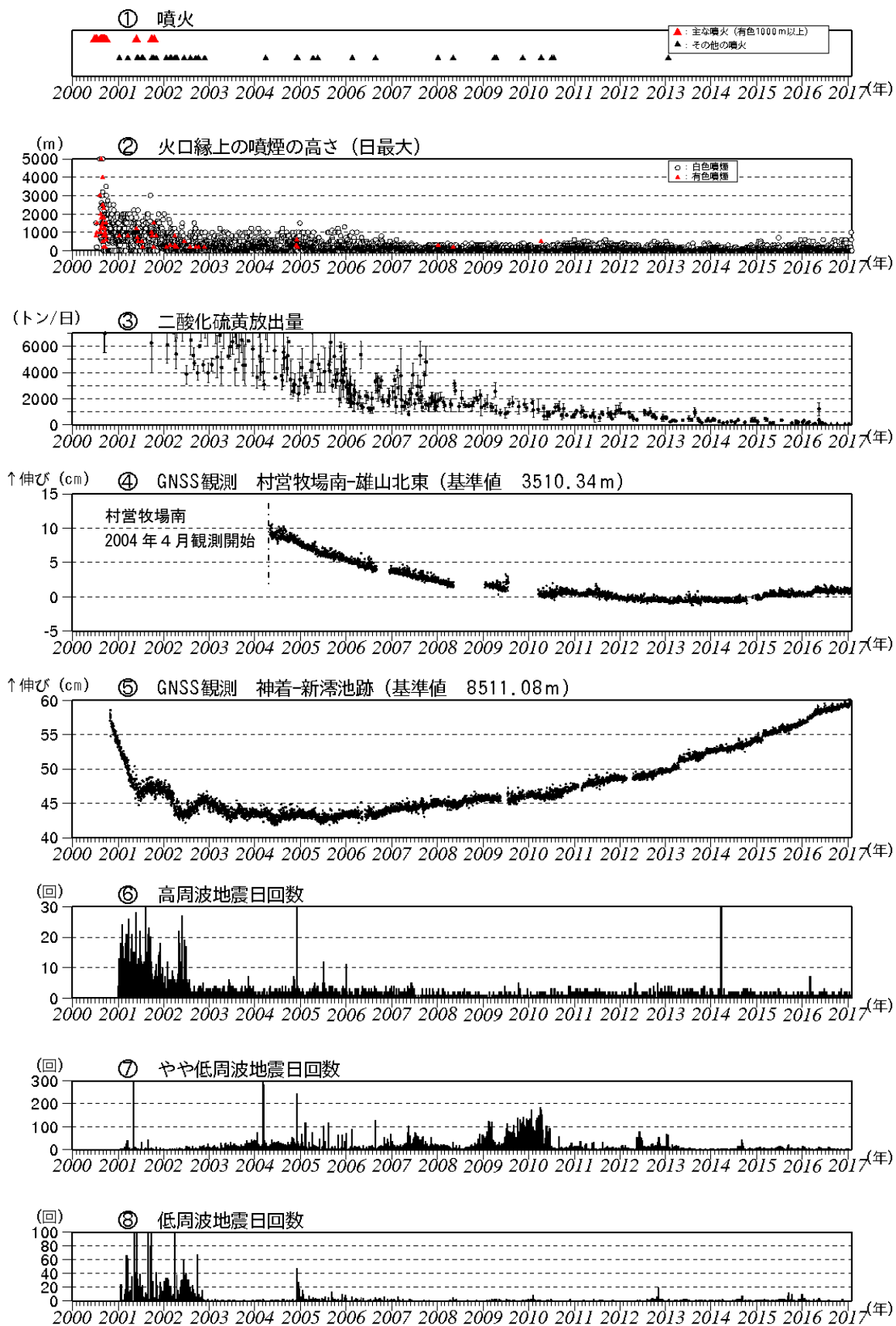
図4 三宅島 火山活動長期経過図 (2000年1月1日~2017年1月31日)
