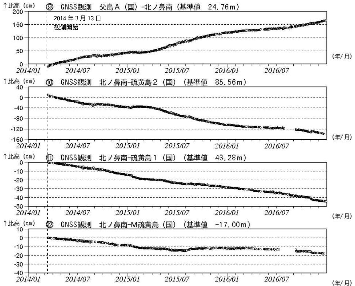
図7 硫黄島 GNSS 観測結果（2014年3月13日～2016年12月31日）（国）：国土地理院
