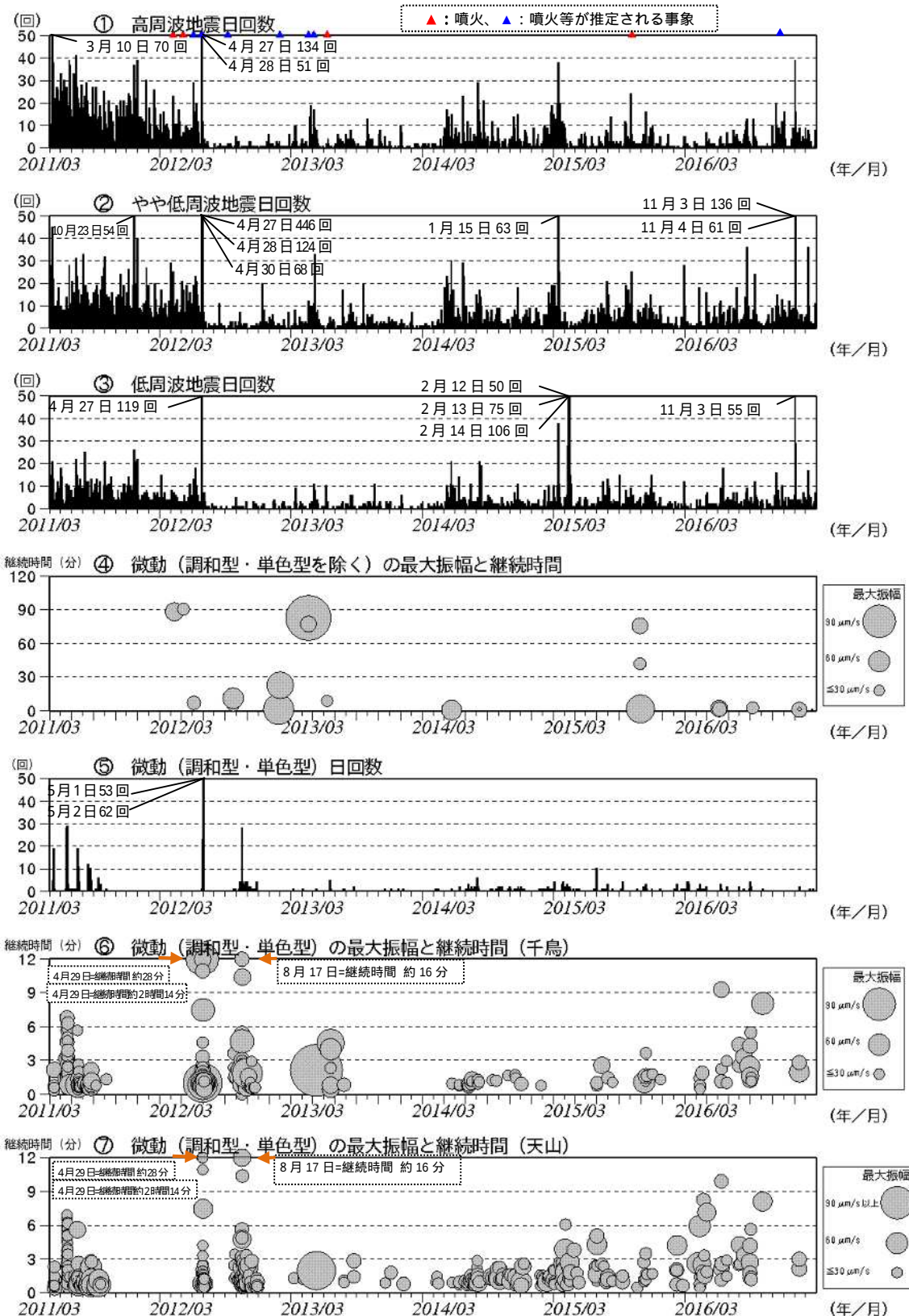
図5 硫黄島 火山活動経過図（2011年3月8日～2016年12月31日）
