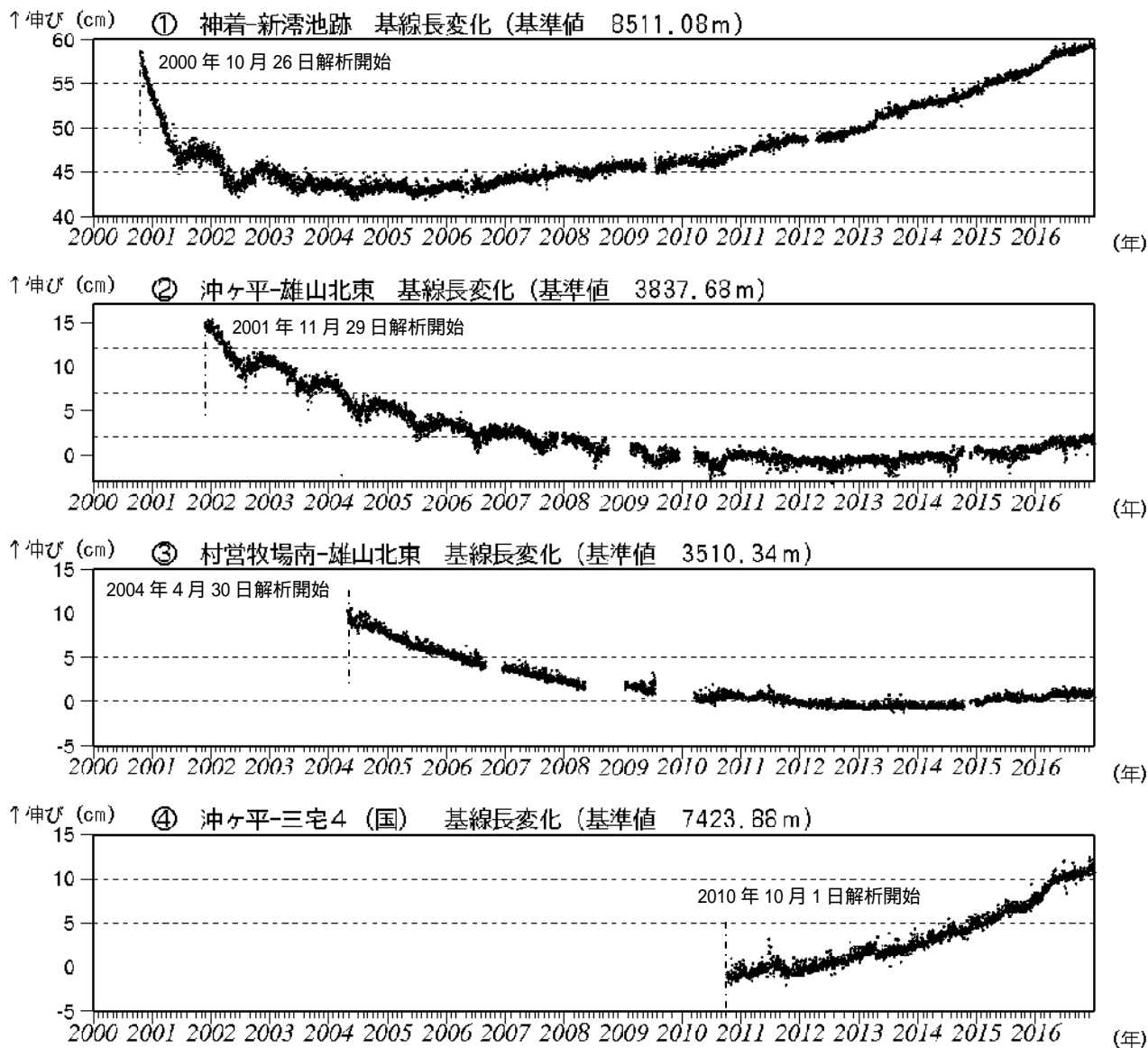
図6 三宅島 GNSS 連続観測結果 (2000年10月26日~2016年12月31日) (国): 国土地理院
