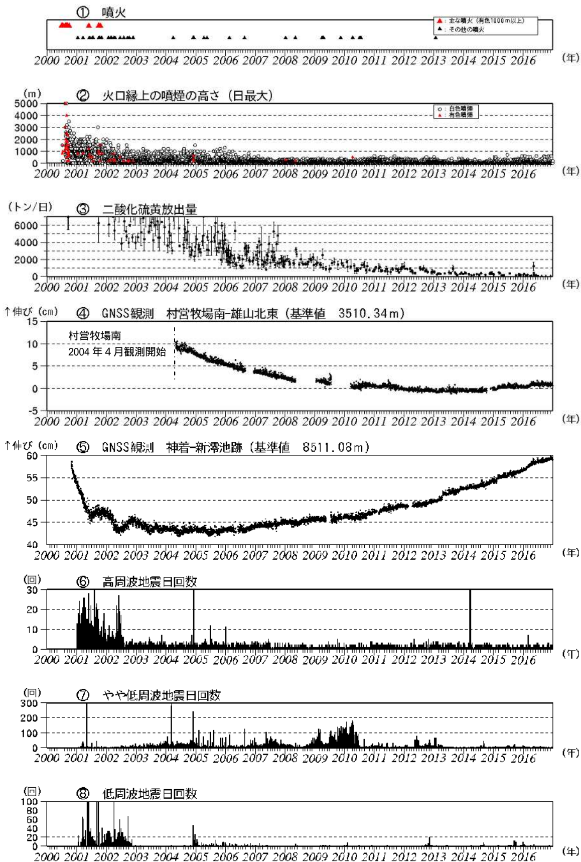
図4 三宅島 火山活動長期経過図(2000年1月1日~2016年12月31日) 図4の説明は次ページに掲載しています。
