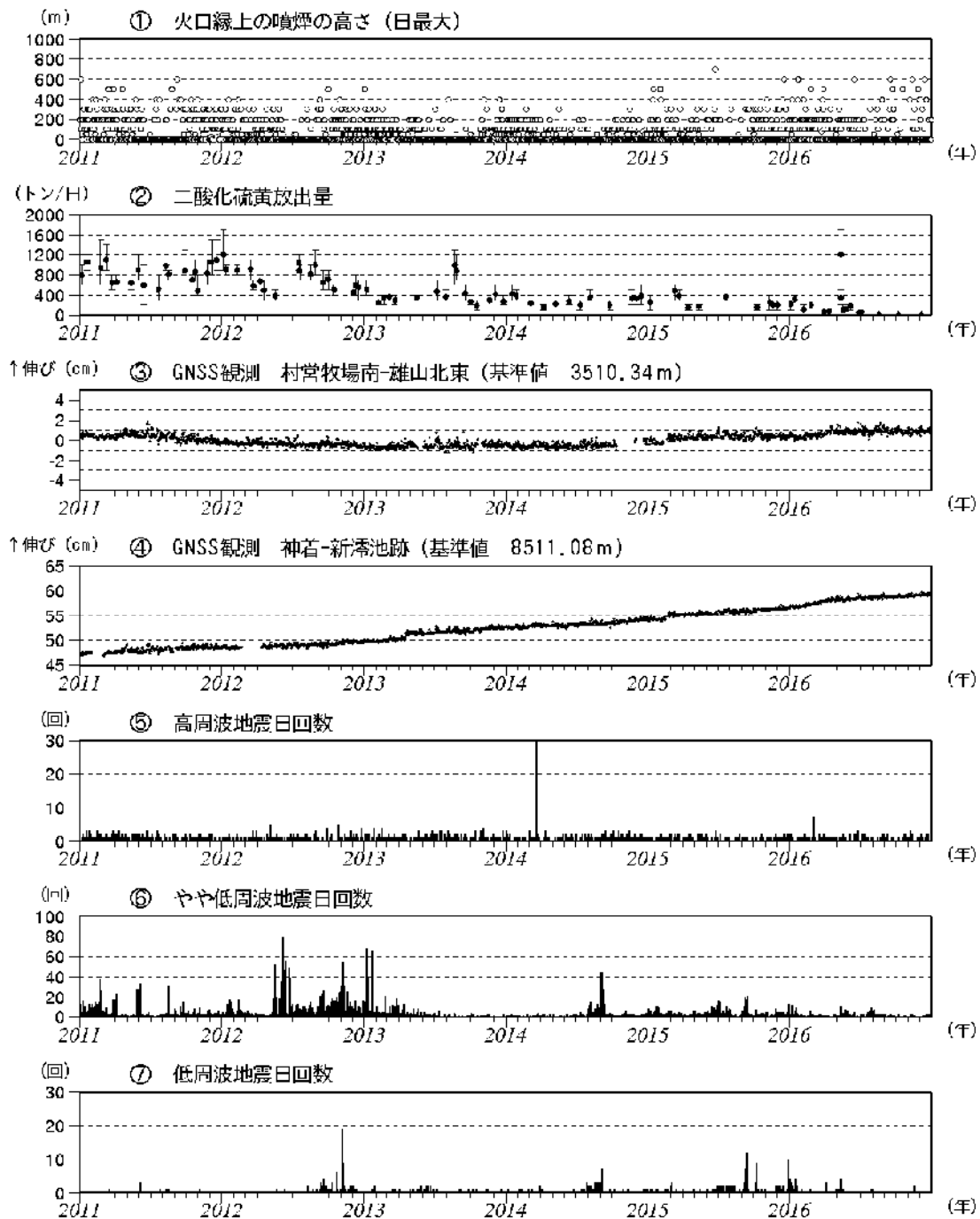
図5 三宅島 火山活動短期経過図(2011年1月1日~2016年12月31日)
