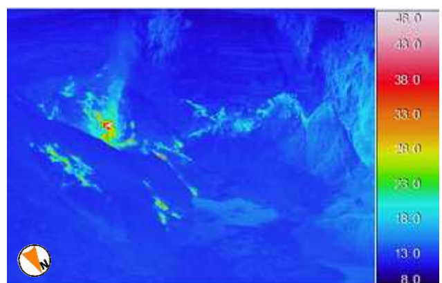
図3 三宅島 赤外熱映像装置による山頂火口内の地表面温度分布(12月9日) ・前回(11月16日)と比べて、火口内の地形、噴気及び高温領域の分布に特段の変化は認められません。
