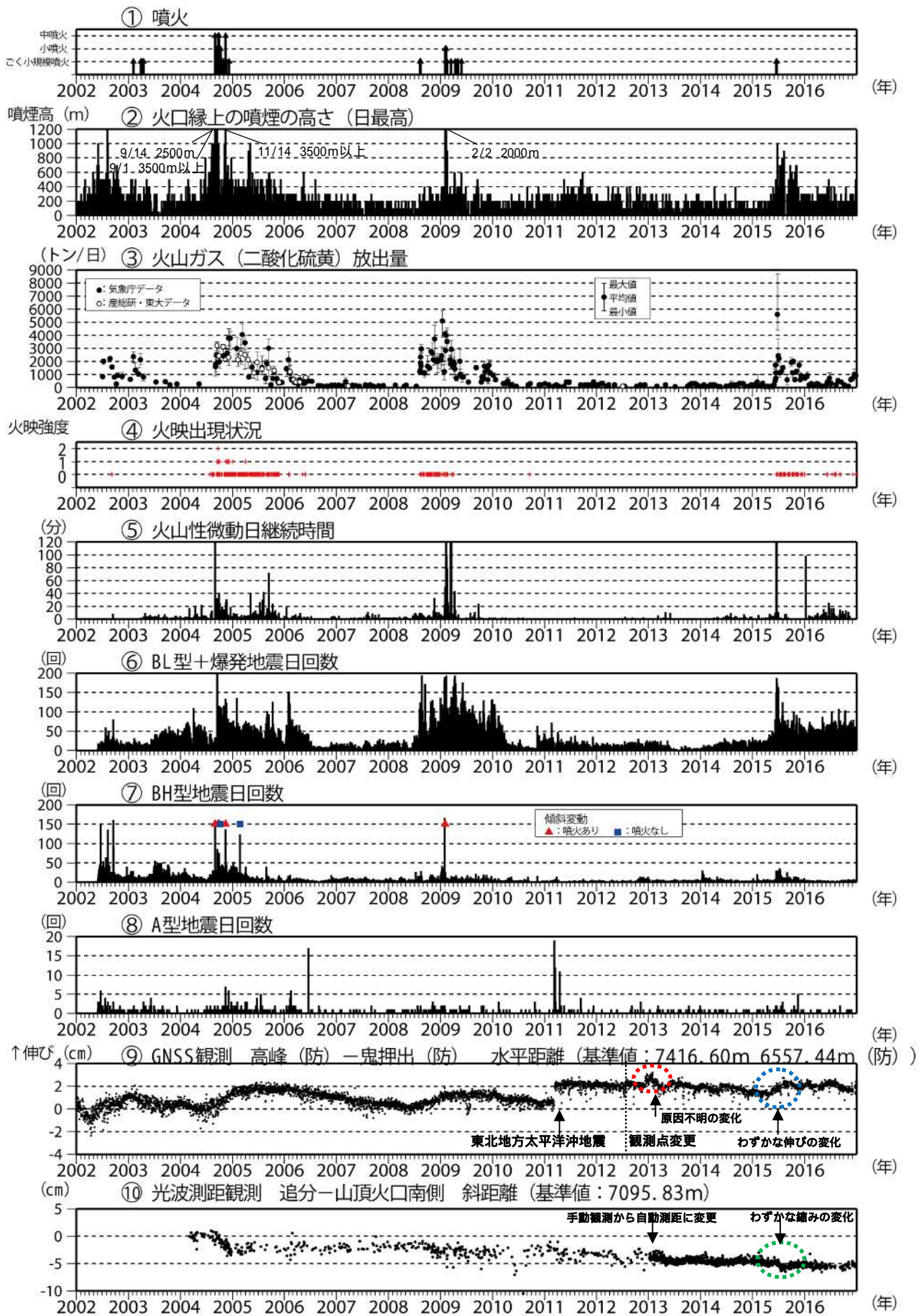
図3 浅間山 火山活動経過図(2002年1月1日~2016年12月31日)
