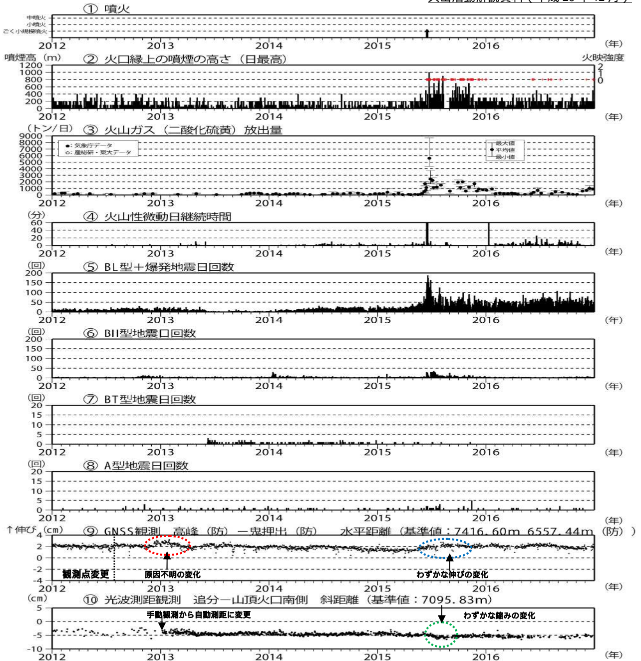
図4 浅間山 最近の火山活動経過図(2012年1月1日~2016年12月31日)
