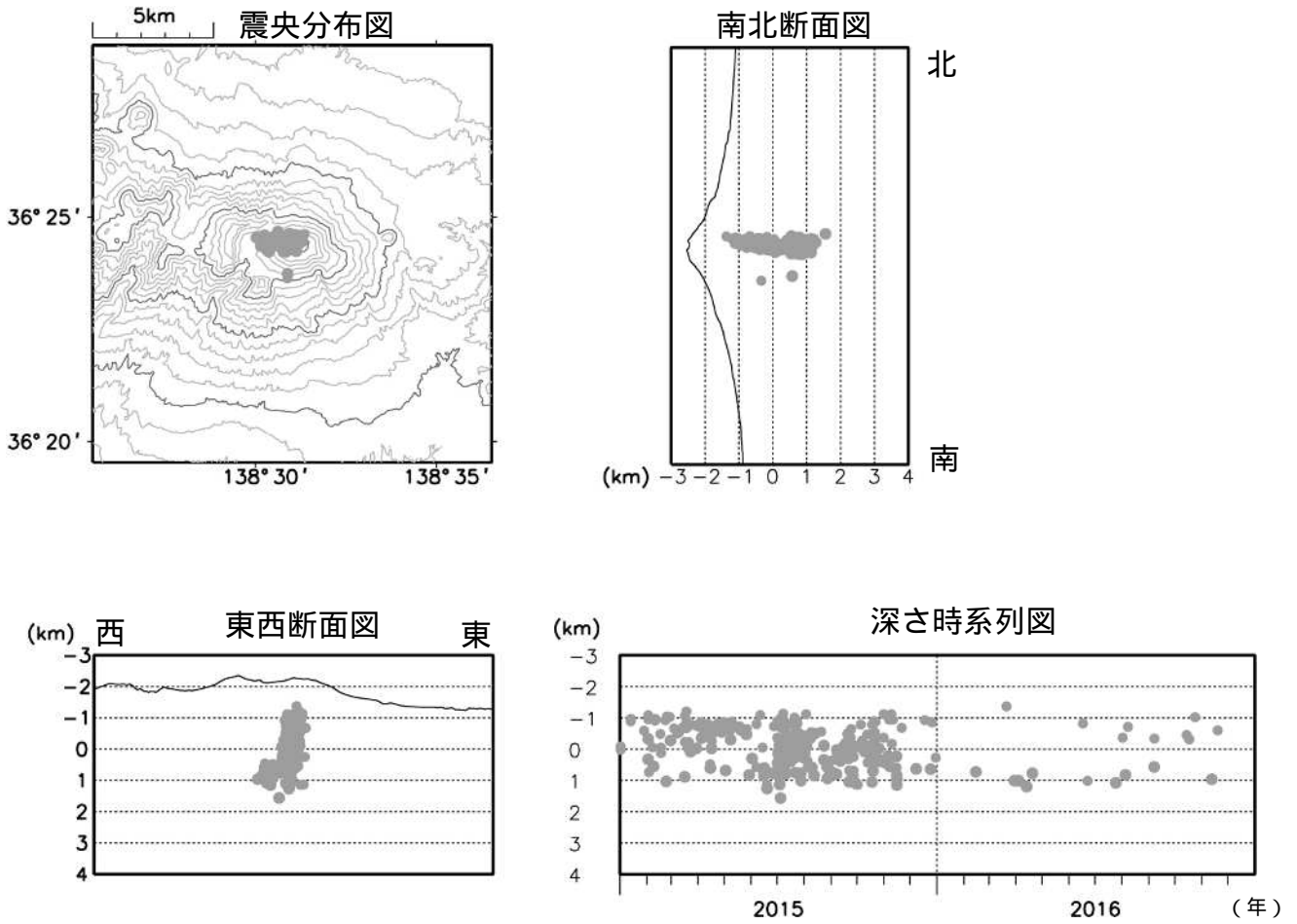
図5 浅間山 震源分布図（2015年1月1日～2016年12月31日）
