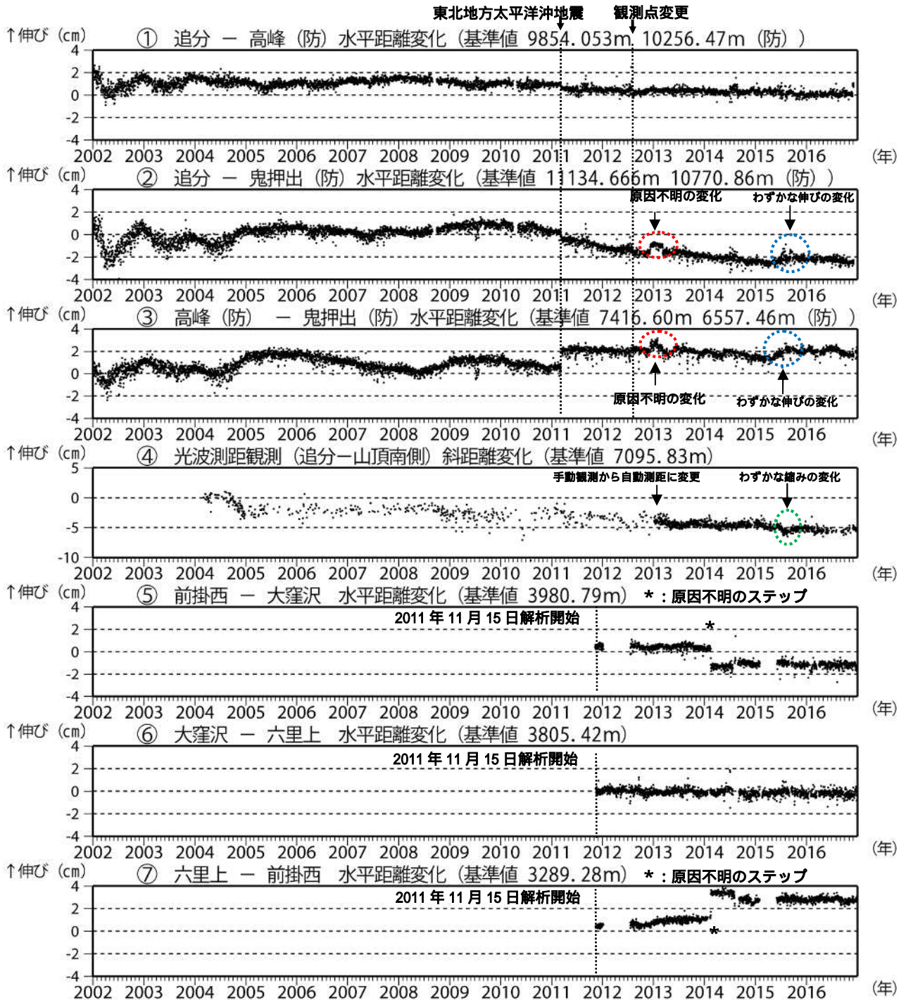
図6 浅間山 GNSS 連続観測及び光波測距観測の結果(2002年1月1日~2016年12月31日)
