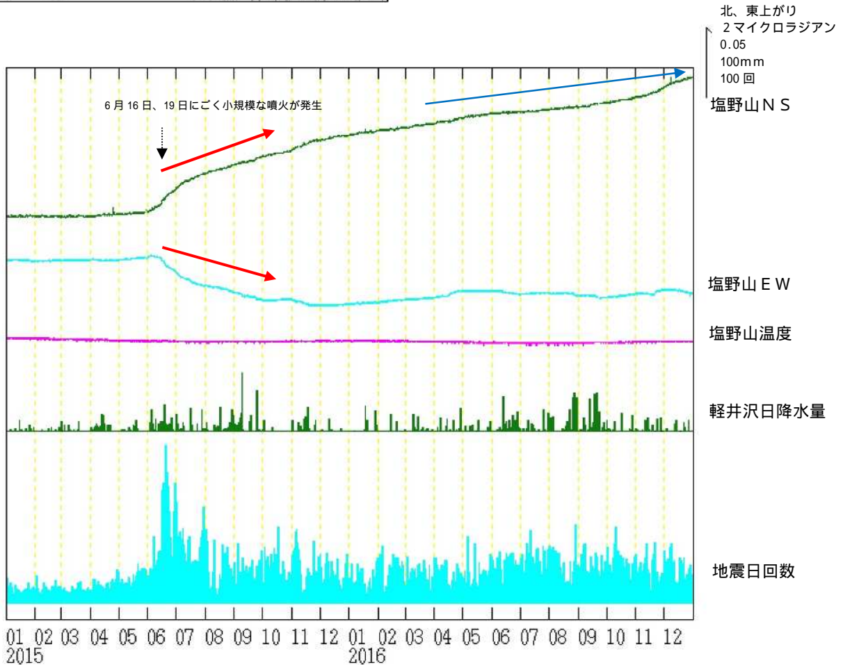
図8 浅間山 塩野山観測点における傾斜データ(2015年1月1日~2016年12月31日)
