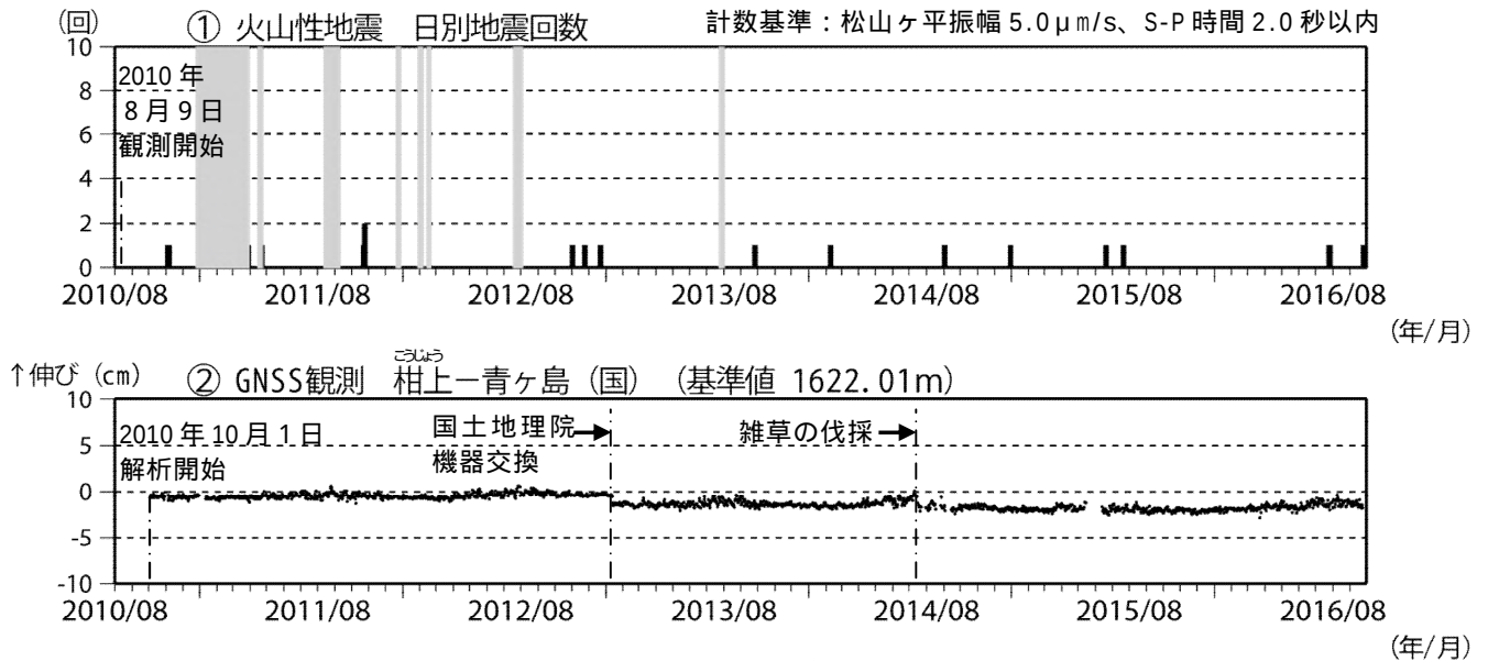
図 2 青ヶ島 火山活動経過図（2010 年 8 月 9 日～2016 年 9 月 30 日）
