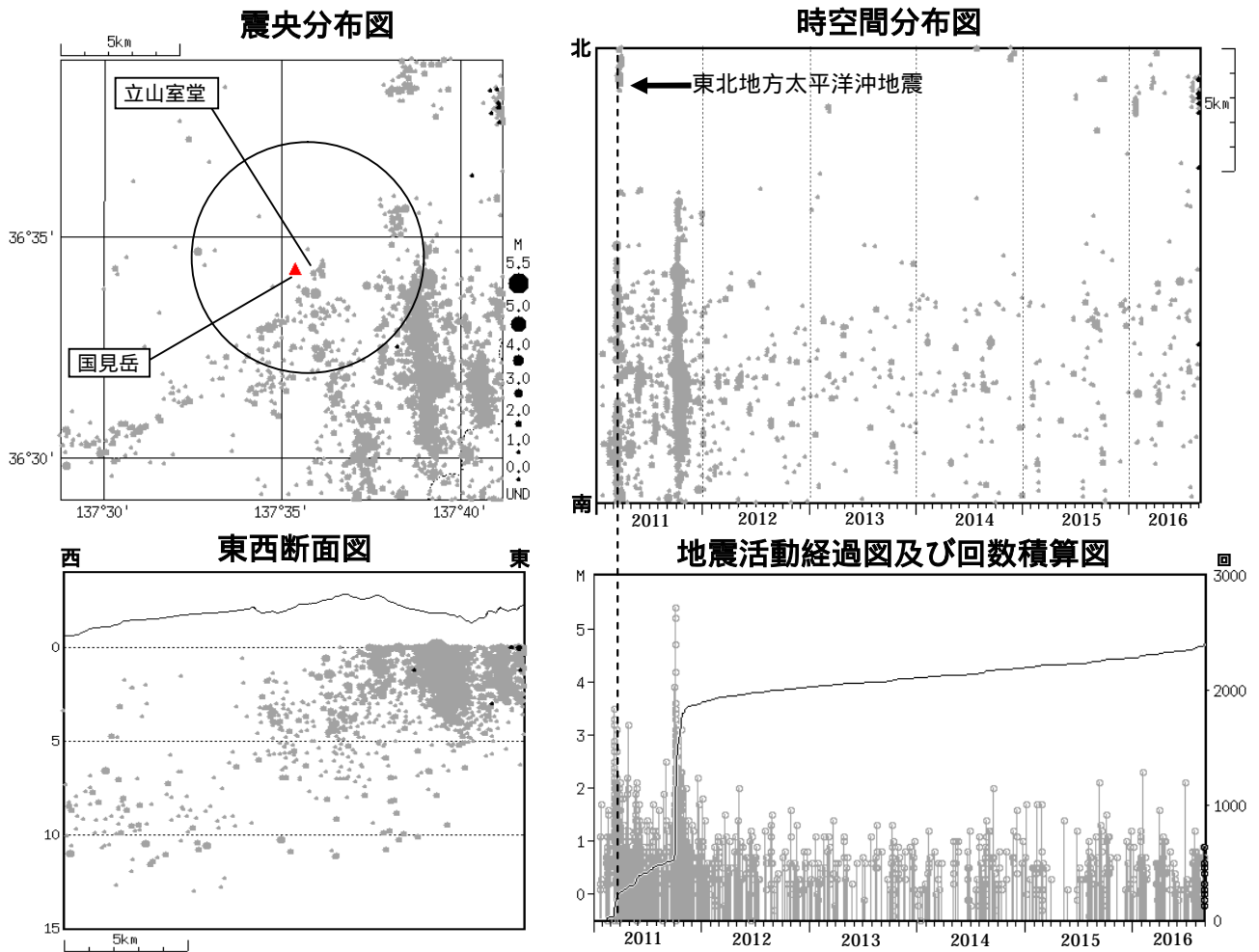
図2 弥陀ヶ原 広域地震観測網による山体・周辺の地震活動（2011年1月1日～2016年8月31日） : 2011年1月1日～2016年7月31日 : 2016年8月1日～8月31日 ・ 震央分布図内の円は、立山室堂に設置した地震計（立山室堂2）で地震回数を計数しているS-P時間1秒以内となるおおよその範囲を示します。 ・ これは広域地震観測網により震源決定したもので、深さは全て海面以下として決定しています。 ・ M（マグニチュード）は地震の規模を表します。 ・ 図中の震源要素は一部暫定値が含まれており、後日変更することがあります。 ・ 弥陀ヶ原近傍の地震活動は、低調に経過しています。
