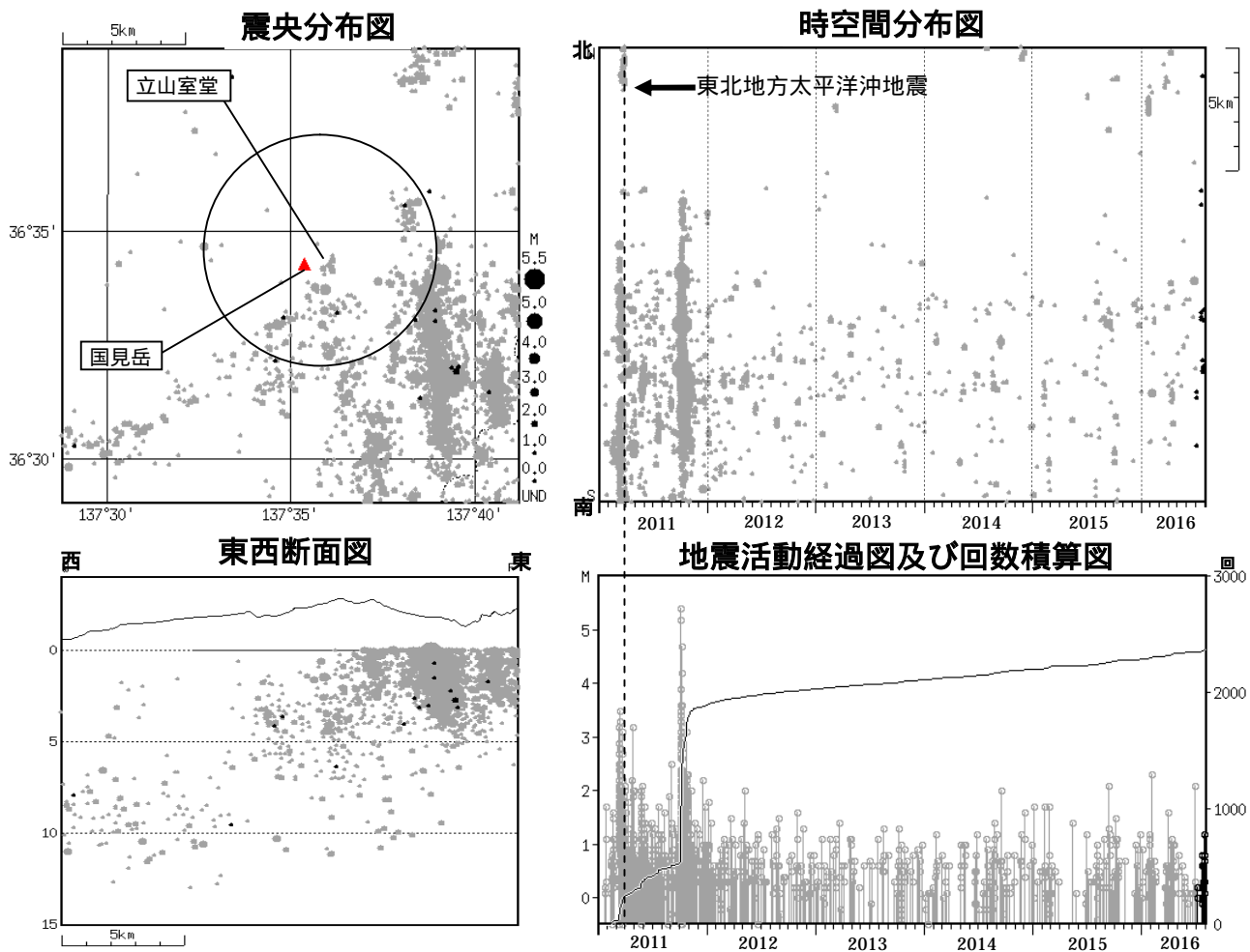
図2 弥陀ヶ原 広域地震観測網による山体・周辺の地震活動(2011年1月1日~2016年7月31日) : 2011年1月1日~2016年6月30日 : 2016年7月1日~7月31日 ・ 震央分布図内の円は、立山室堂に設置した地震計(立山室堂2)で地震回数を計数しているS-P時間1秒以内となるおおよその範囲を示します。 ・ M(マグニチュード)は地震の規模を表します。 ・ 図中の震源要素は一部暫定値が含まれており、後日変更することがあります。 ・ 弥陀ヶ原近傍の地震活動は、低調に経過しています。
