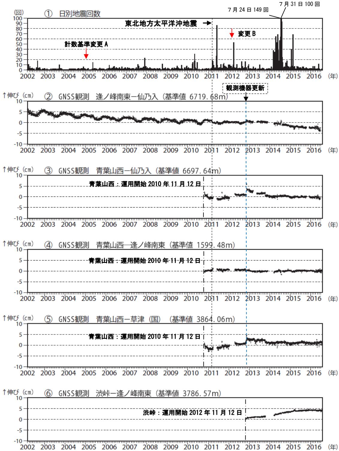
図5 草津白根山 火山活動経過図（2002年4月1日～2016年7月31日）
