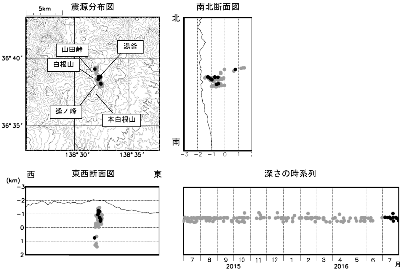
図3 草津白根山 震源分布図（2015年7月1日～2016年7月31日）
