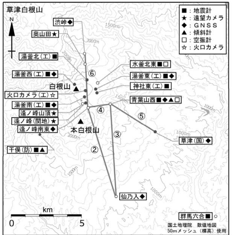
図1 草津白根山 観測点配置図
