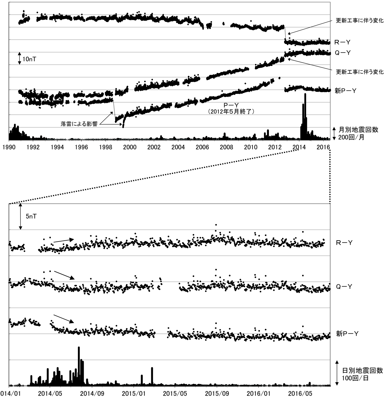
図6 草津白根山 全磁力連続観測による全磁力値の変化及び地震回数 上段：1990年～2016年7月27日、下段：2014年1月～2016年7月27日
