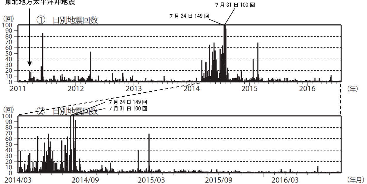
図4 草津白根山 日別地震回数（2011年1月1日～2016年7月31日）
