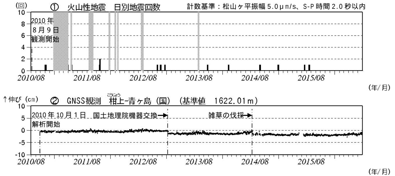
図 2 青ヶ島 火山活動経過図 (2010 年 8 月 9 日 ~ 2016 年 6 月 30 日) 青ヶ島周辺の日別地震回数 グラフの灰色部分は機器障害による欠測。 GNSS 連続観測による基線長変化 (国): 国土地理院 は図 3 の GNSS 基線 に対応。グラフの空白部分は欠測。 ・2014 年 7 月 15 日に実施した雑草の伐採の影響により、ステップ状の変化がみられます。
