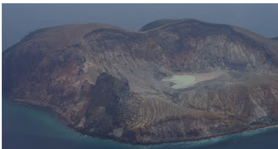
図3 硫黄島 硫黄島の南西方向へ拡大する変色水域(1日) (第十一管区海上保安本部提供) ・硫黄島の西側海岸線に沿って青白色の変色水が分布していました。
