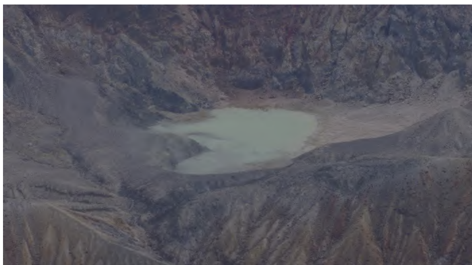
図2 硫黄島 硫黄岳火口の噴気の状況(1日) (第十一管区海上保安本部提供) ・硫黄岳火口内に弱い白色噴気が認められました。
