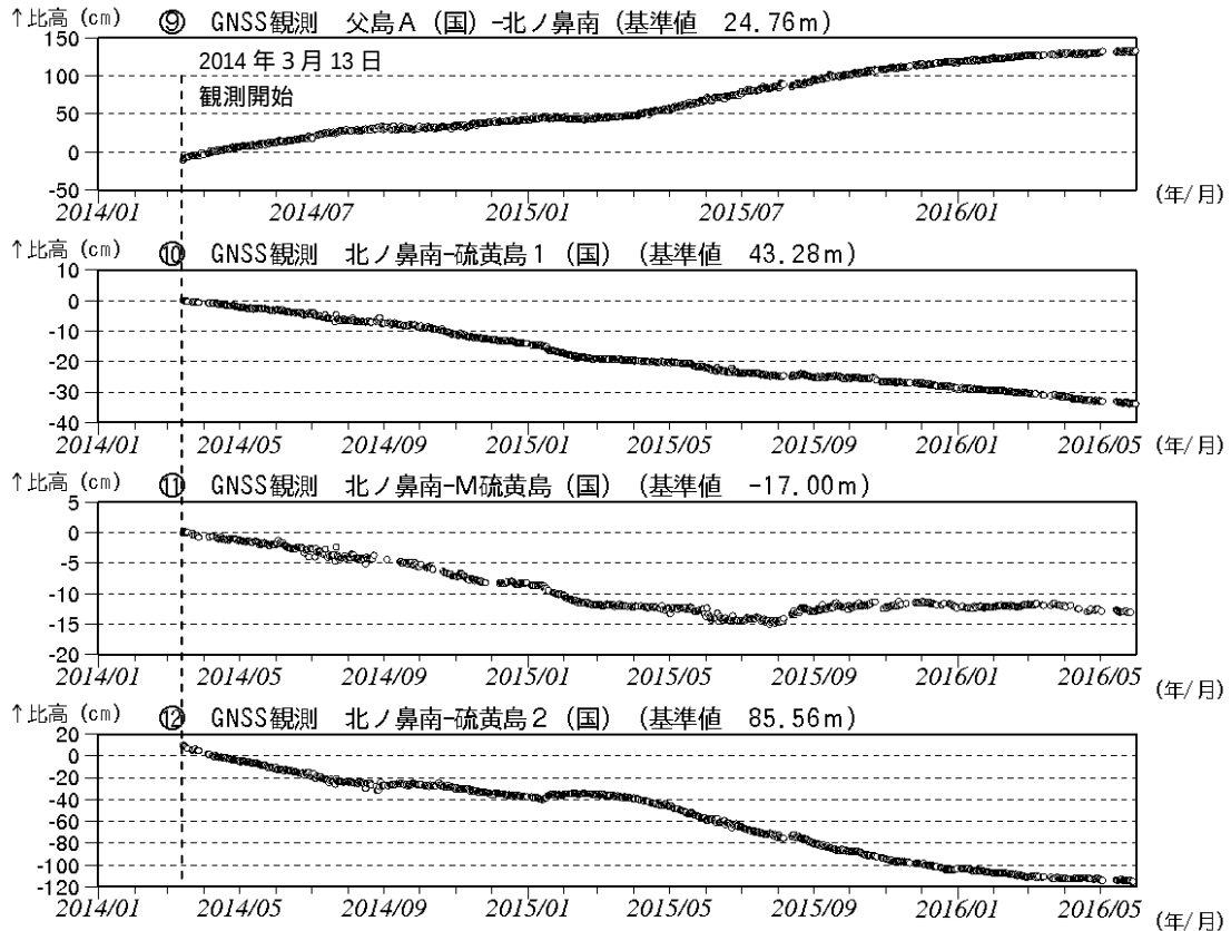
図7 硫黄島 GNSS 1) 観測結果（2014年3月13日～2016年5月31日）（国）：国土地理院
