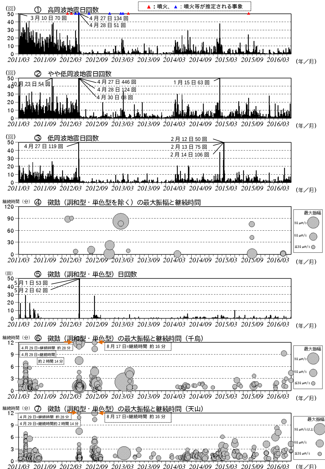
図5 硫黄島 火山活動経過図（2011年3月8日～2016年5月31日）
