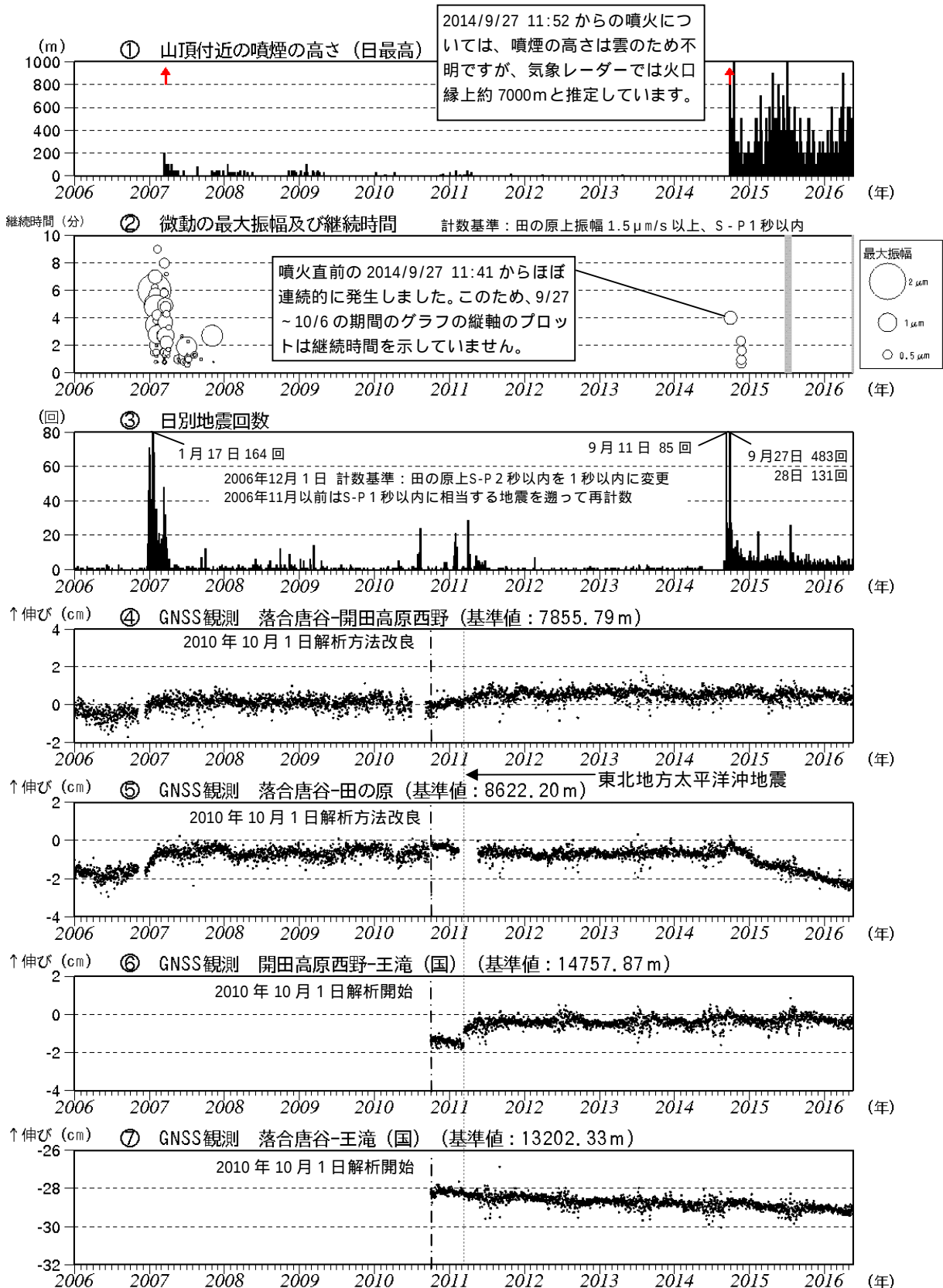
図 5 御嶽山 長期間の火山活動経過図（2006 年 1 月 1 日～2016 年 5 月 31 日）
