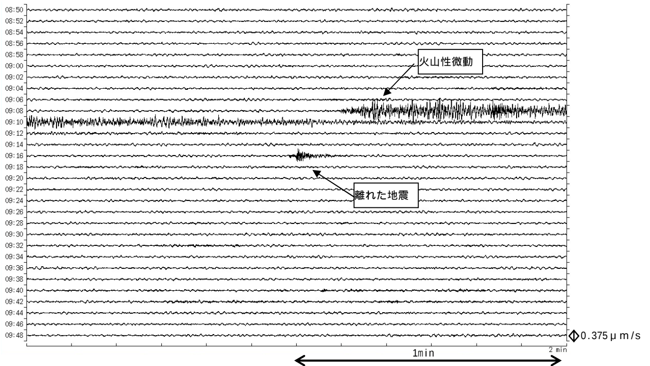
図3 御嶽山 火山性微動の状況（5月19日、田の原観測点上下成分）
