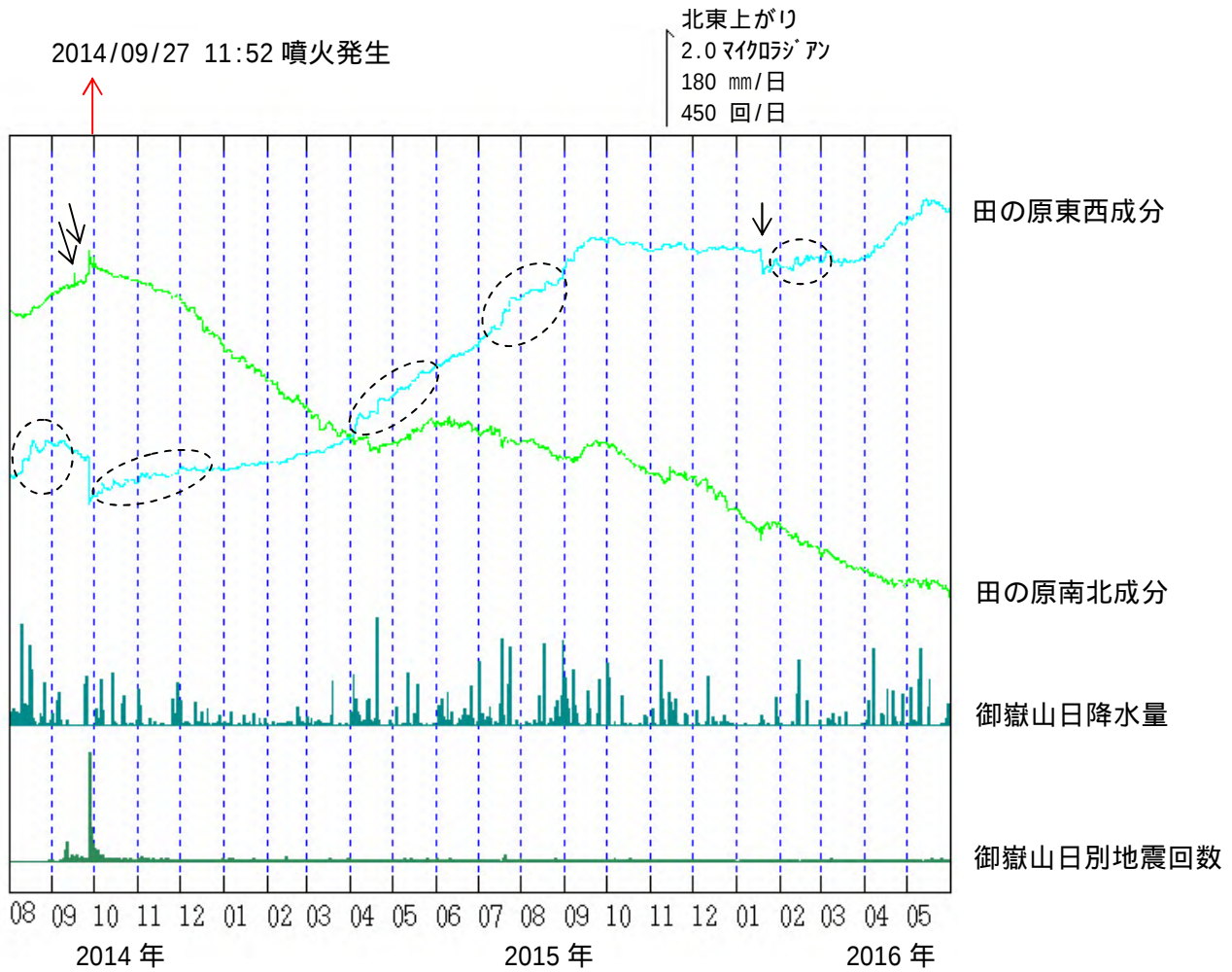
図6 御嶽山 田の原観測点（剣ヶ峰山頂の南東約3 km）の傾斜変動 （2014年8月1日～2016年5月31日）
