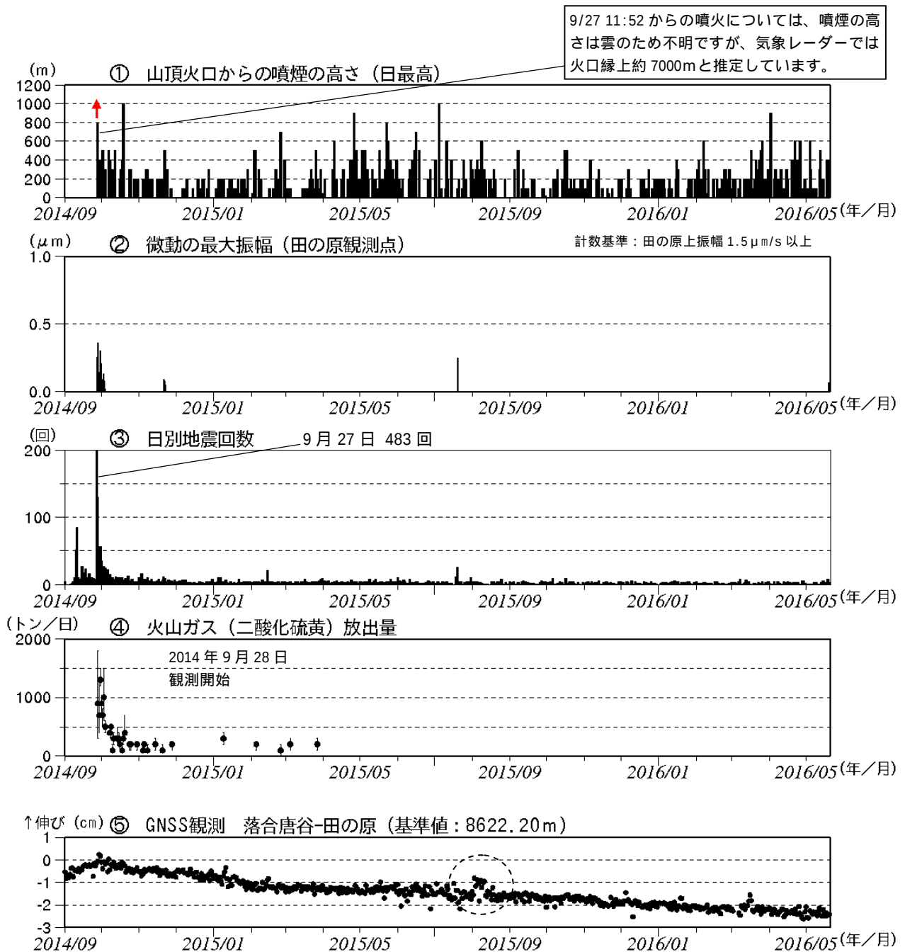
図 4 御嶽山 最近の火山活動経過図（2014 年 9 月 1 日～2016 年 5 月 31 日）
