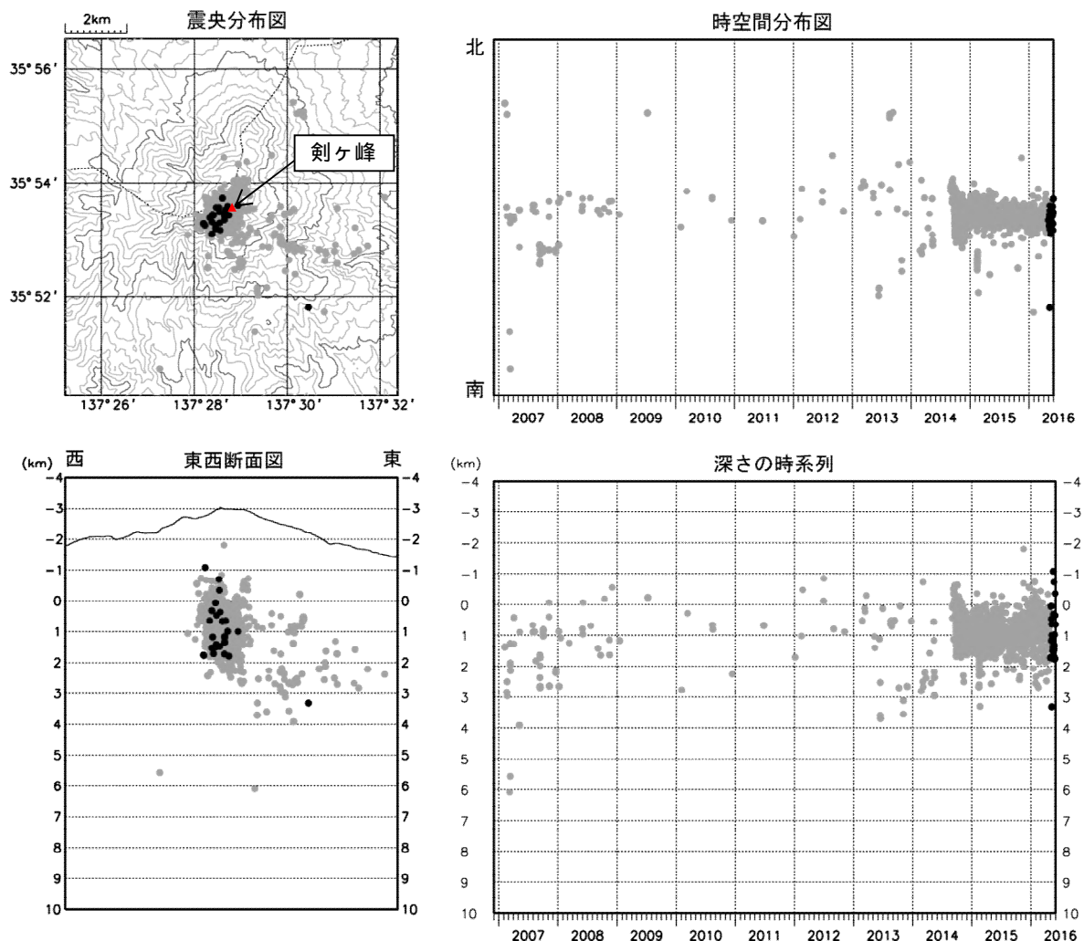
図 2 御嶽山 震源分布図（2006 年 12 月 1 日～2016 年 5 月 31 日）
