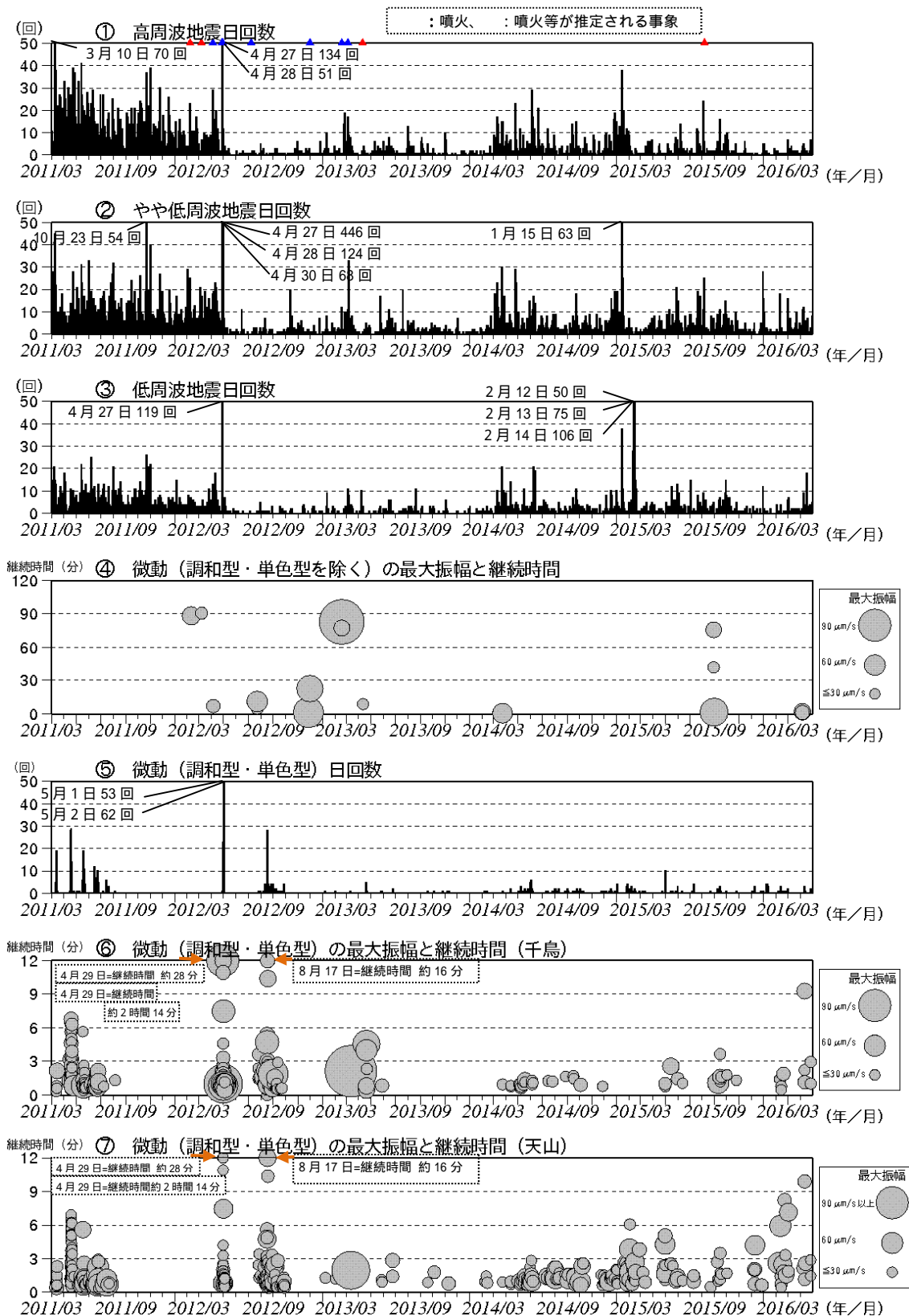
図5 硫黄島 火山活動経過図（2011年3月8日～2016年4月30日）
