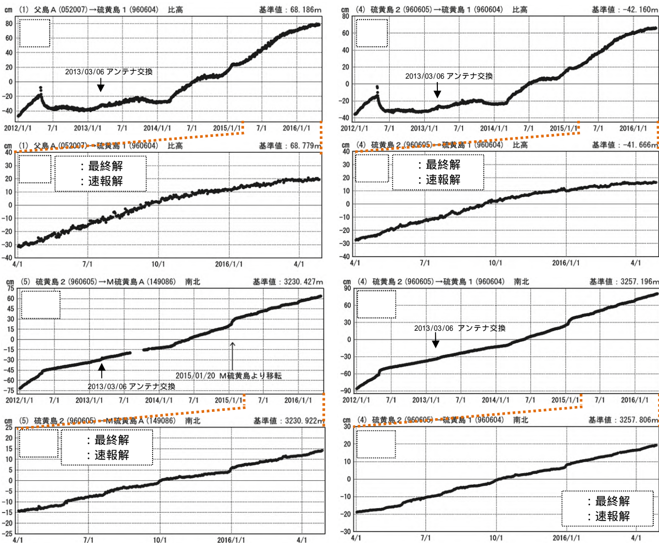
図6 硫黄島 国土地理院による地殻変動観測結果 2) ( 2012年1月1日~2016年4月26日、 2015年4月1日~2016年4月26日 ) のグラフ: 父島に対する硫黄島1の比高の変化 のグラフ: 硫黄島2(島西部の摺鉢山付近)に対する硫黄島1(島北部の元山地域)の比高の変化 のグラフ: 硫黄島2に対するM硫黄島(島西部の阿蘇台陥没孔付近)の南北の変化 のグラフ: 硫黄島2に対する硫黄島1の南北の変化
