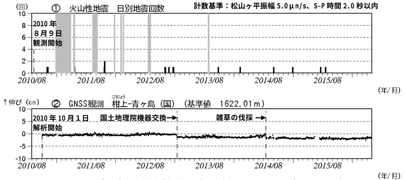
図2 青ヶ島 火山活動経過図（2010年8月9日～2016年4月30日）
