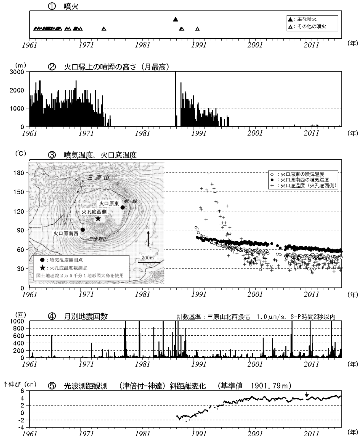
図1 伊豆大島 長期間の火山活動経過図（1961年1月～2016年4月30日）
