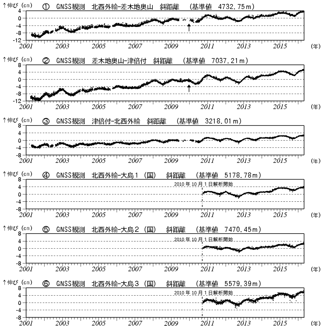
図3 伊豆大島 GNSS連続観測による基線長変化(2001年1月～2016年4月30日)(国): 国土地理院 2010年10月以降のデータについては、電離層の影響を補正する等、解析方法を改良しています。 ~ は図8のGNSS基線 ~ に対応しています。 グラフの空白部分は欠測。 の矢印は差木地奥山支柱工事を実施。 ・長期的な山体膨張に加えて約1年周期で膨張と収縮を繰り返す変動がみられています。最近では、2015年1月頃から収縮傾向でしたが、10月頃から膨張傾向になっています。
