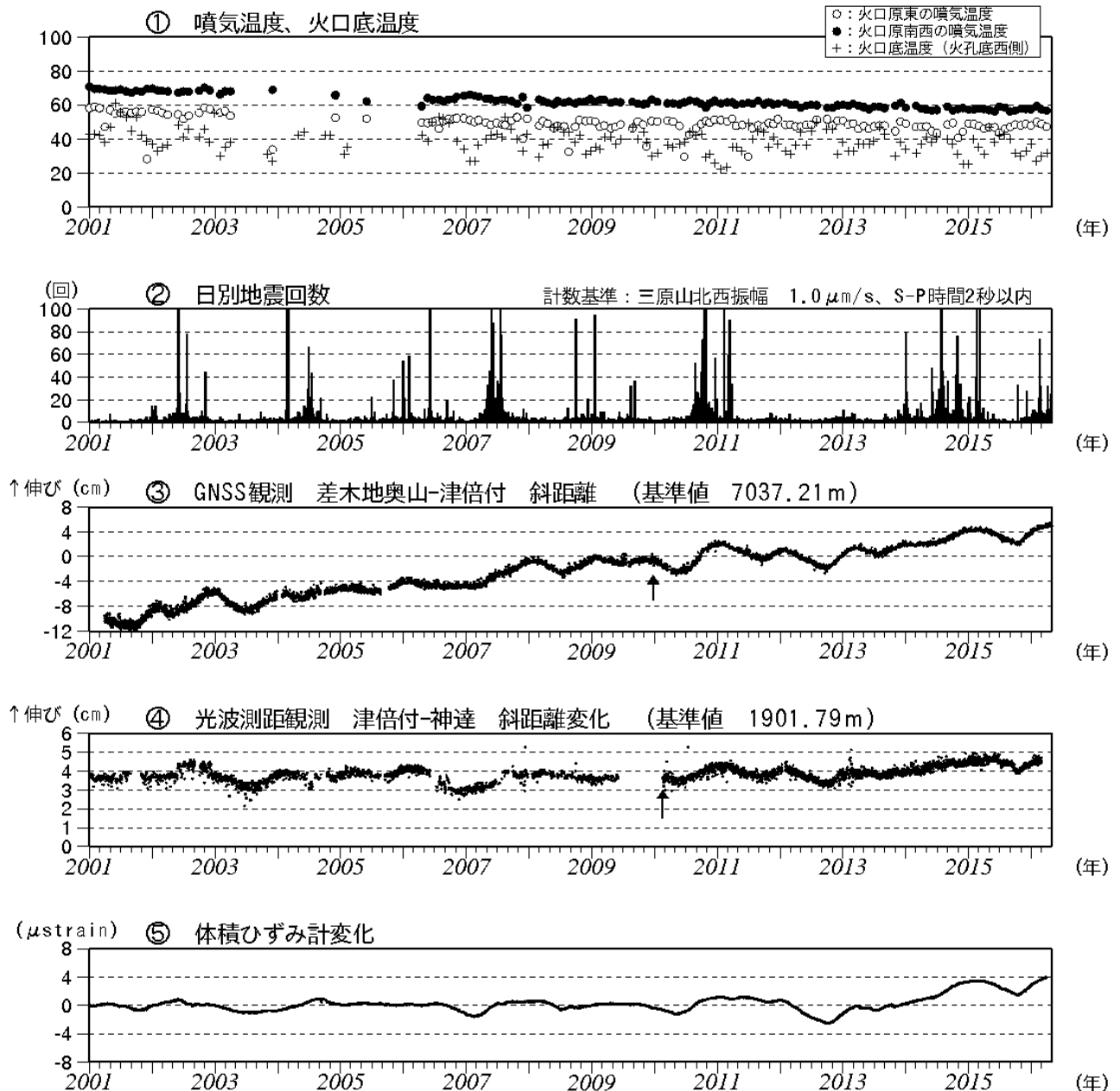
図2 伊豆大島 最近の火山活動経過図(2001年1月~2016年4月30日)
