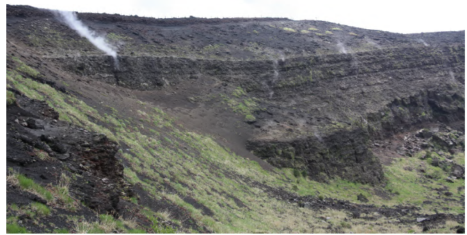
山頂部（4月20日、北西外輪遠望カメラによる） 剣ガ峰付近（4月19日、撮影方向は図7参照） 図5 伊豆大島 三原山山頂部及び山頂火口の状況
