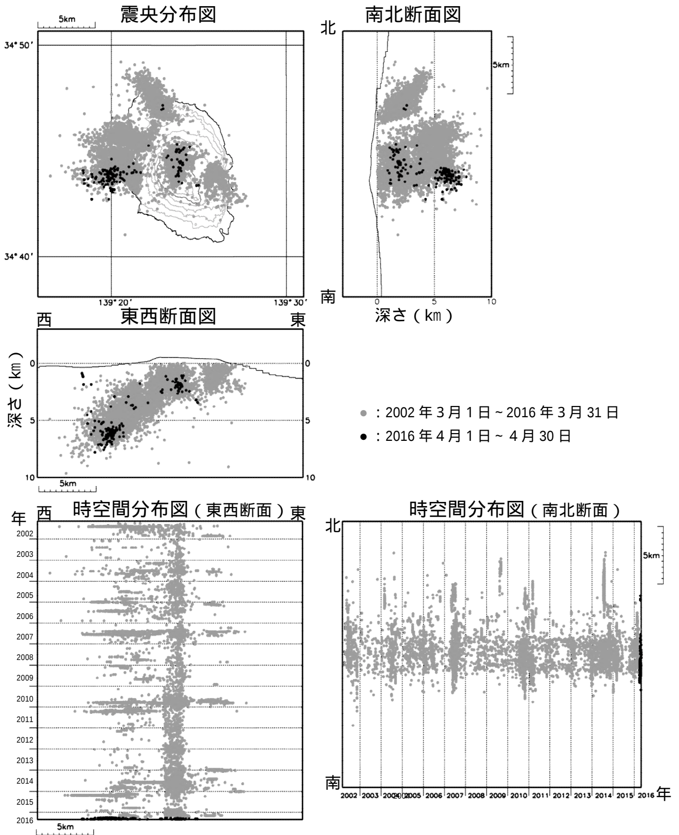
図 4 伊豆大島 震源分布図（2002 年 3 月 1 日～2016 年 4 月 30 日）
