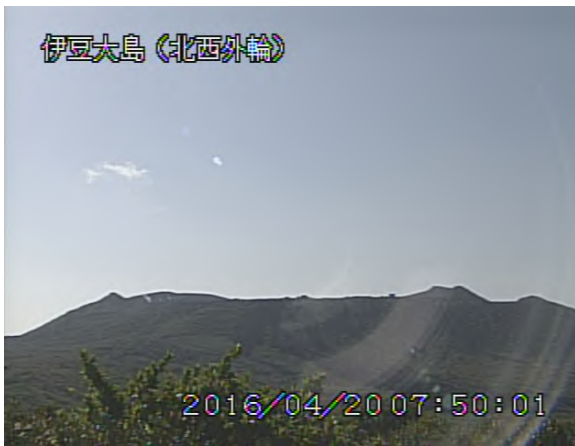
山頂部（4月20日、北西外輪遠望カメラによる） 剣ガ峰付近（4月19日、撮影方向は図7参照） 図5 伊豆大島 三原山山頂部及び山頂火口の状況
