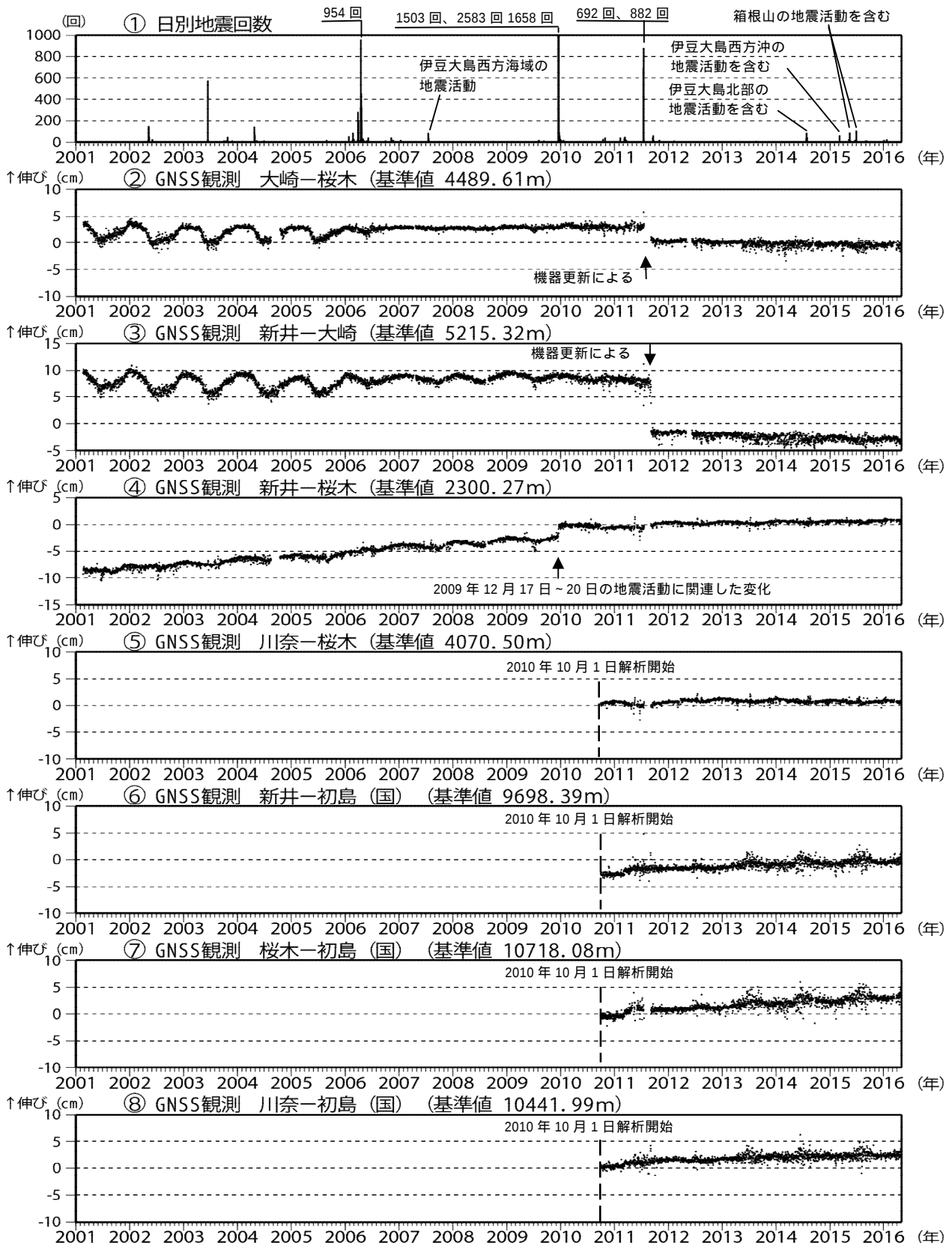
図3 伊豆東部火山群 火山活動経過図(2001年1月1日~2016年4月30日)
