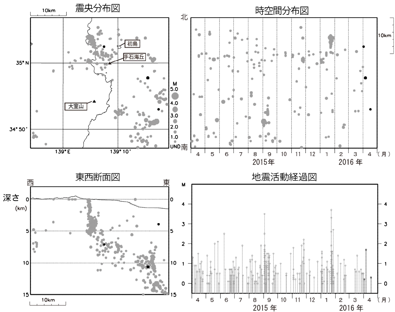
図 2 伊豆東部火山群 広域地震観測網による震源分布図（2015 年 4 月 1 日～2016 年 4 月 30 日） ・ M（マグニチュード）は地震の規模を表します。 ・ 図中の震源要素は一部暫定値が含まれており、後日変更することがあります。
