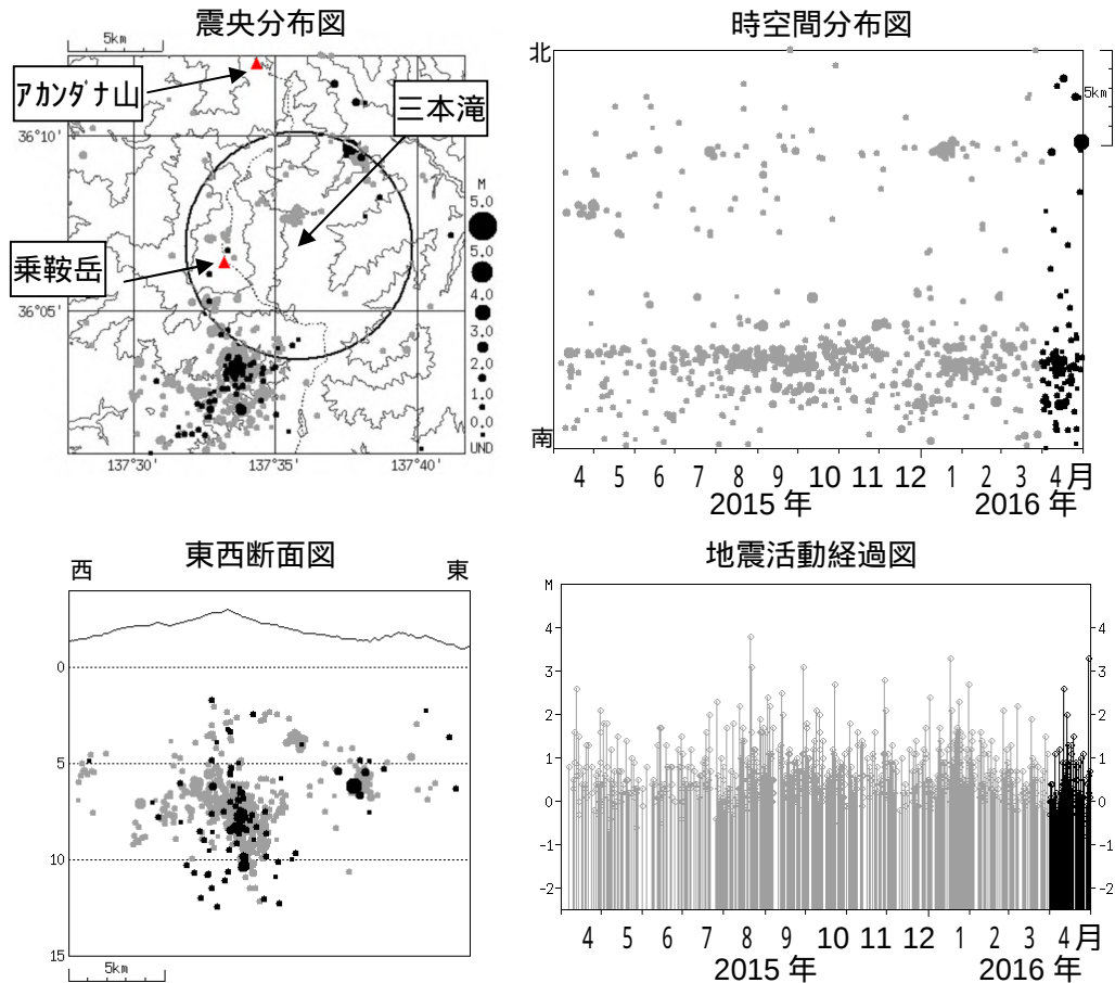
図 3 乗鞍岳 広域地震観測網による山体・周辺の地震活動(2015 年 4 月 1 日～2016 年 4 月 30 日)
