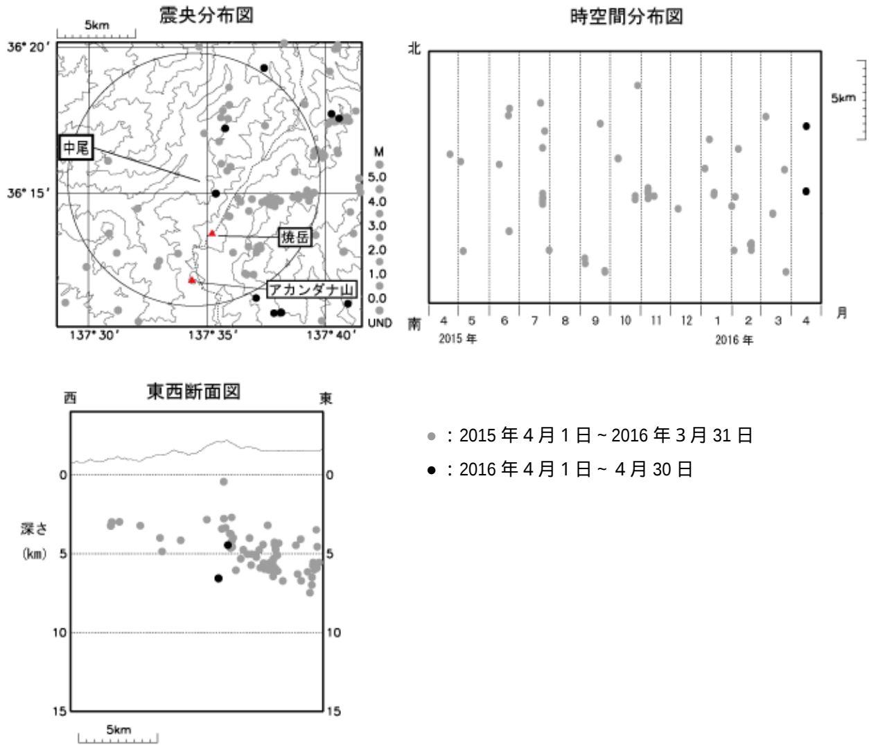
図 3 焼岳 震源分布図（2015 年 4 月 1 日 ~ 2016 年 4 月 30 日）
