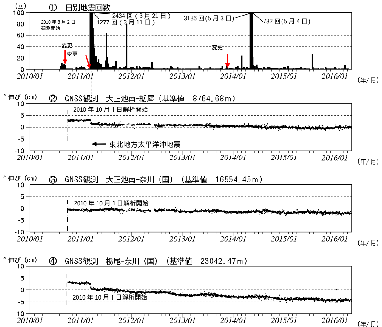
図 2 焼岳 火山活動経過図（2010年 8 月 2 日～2016年 4 月30日）
