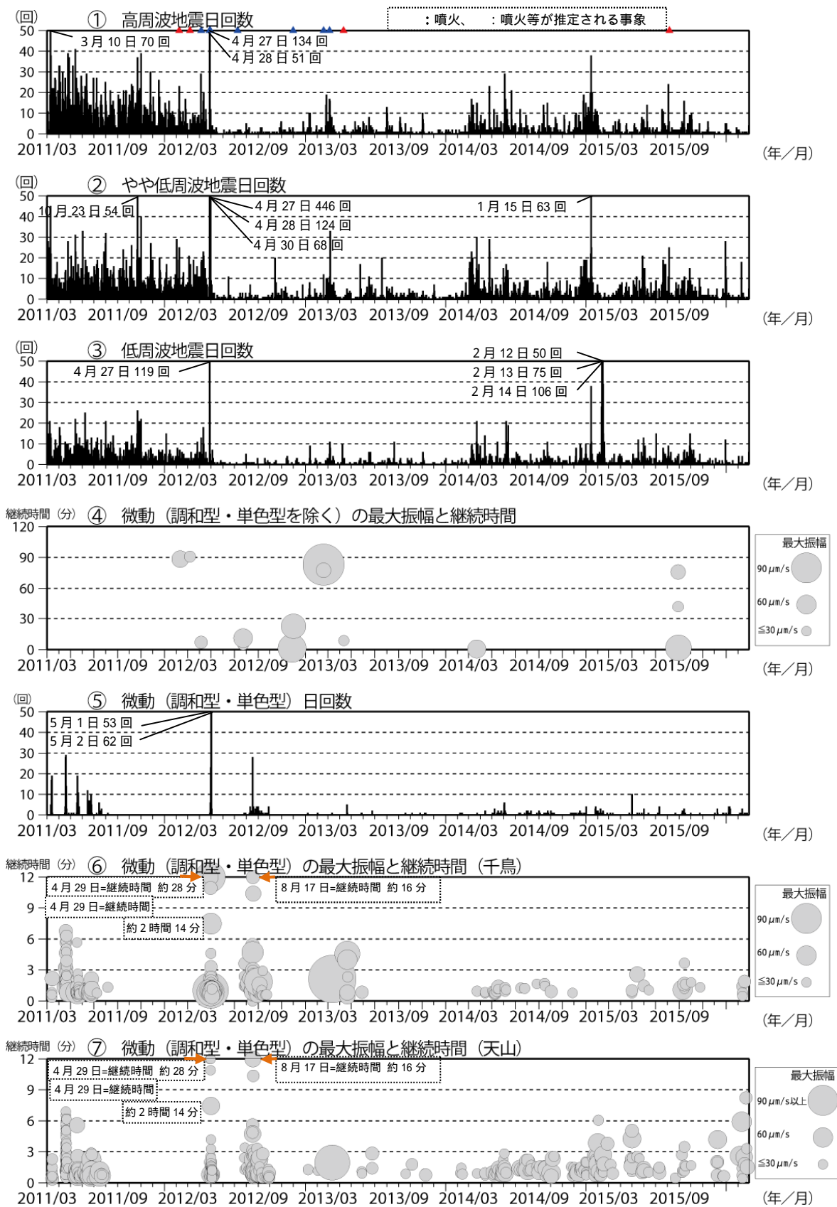
図4 硫黄島 火山活動経過図（2011年3月8日～2016年2月29日）
