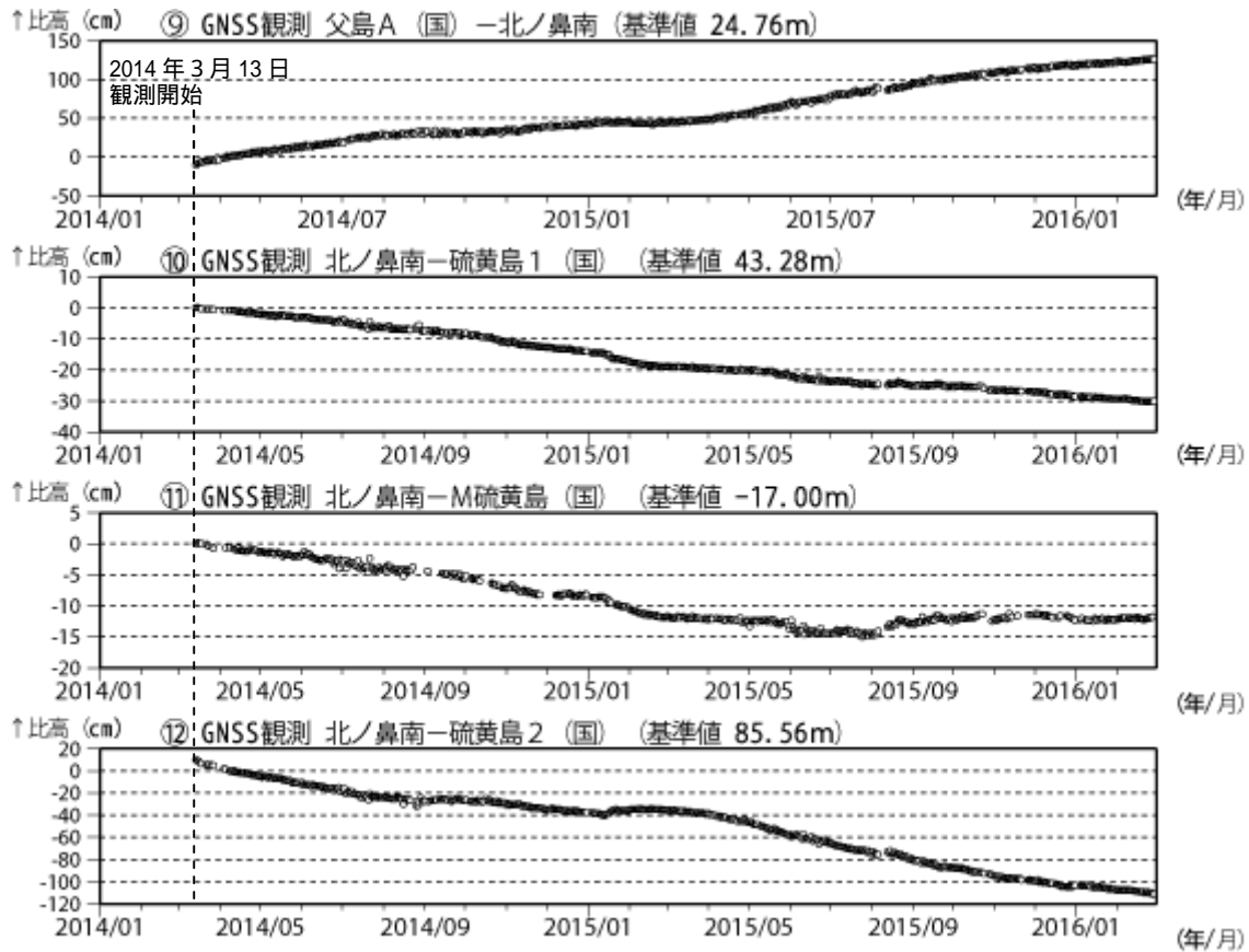
図 6 硫黄島 GNSS 観測結果（2014 年 1 月～2016 年 2 月）（国）：国土地理院
