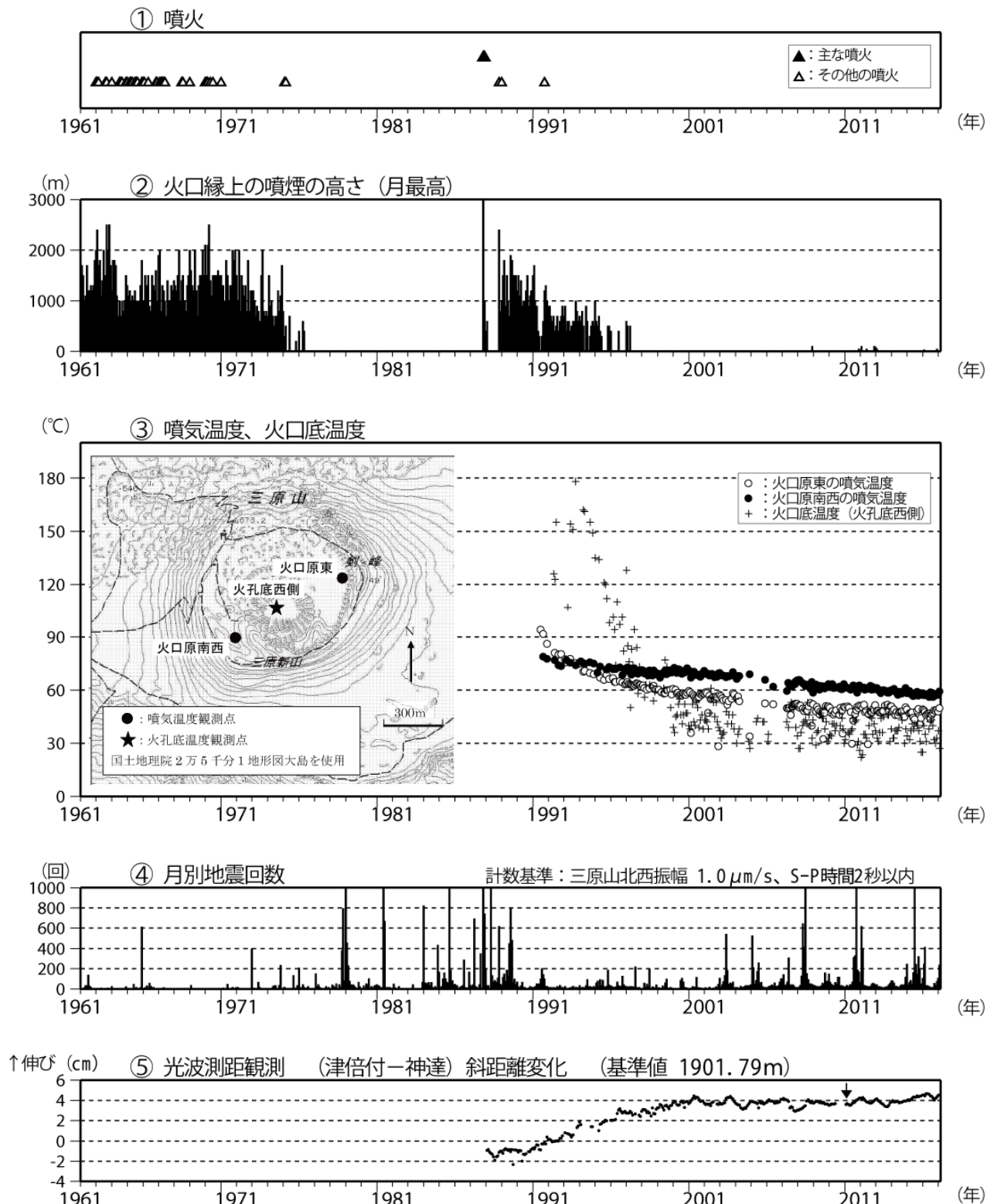
図 1 伊豆大島 長期間の火山活動経過図（1961 年 1 月～2016 年 2 月 29 日）
