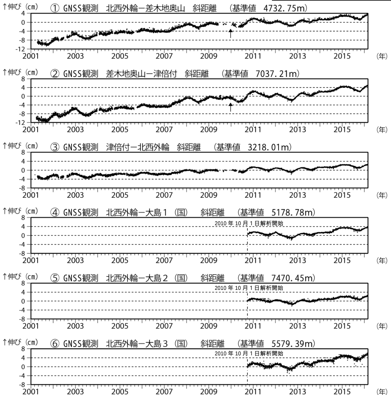
図3 伊豆大島 GNSS 連続観測による基線長変化(2001 年 1 月～2016 年 2 月 29 日)(国): 国土地理院
