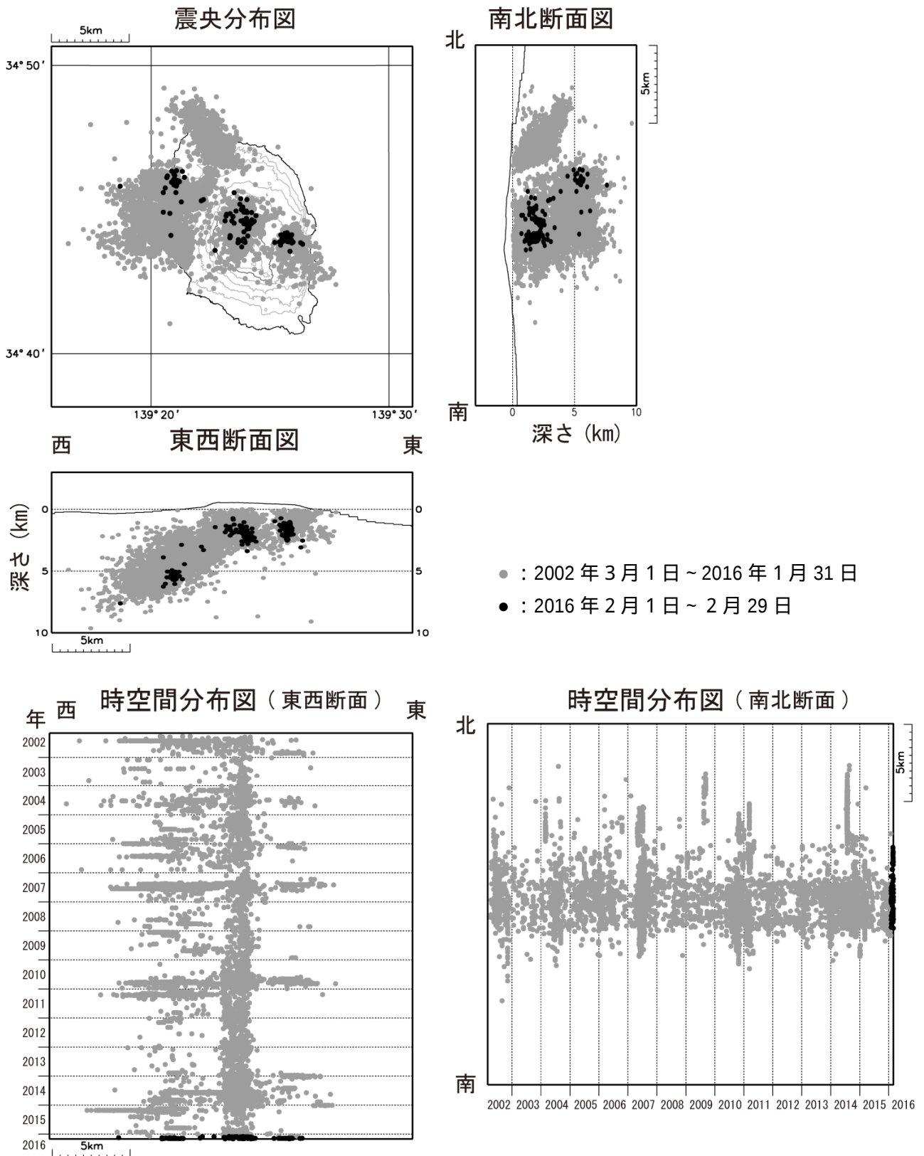
図 4 伊豆大島 震源分布図（2002 年 3 月 1 日～2016 年 2 月 29 日）
