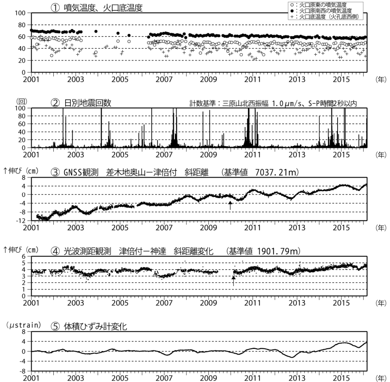
図2 伊豆大島 最近の火山活動経過図（2001年1月～2016年2月29日）
