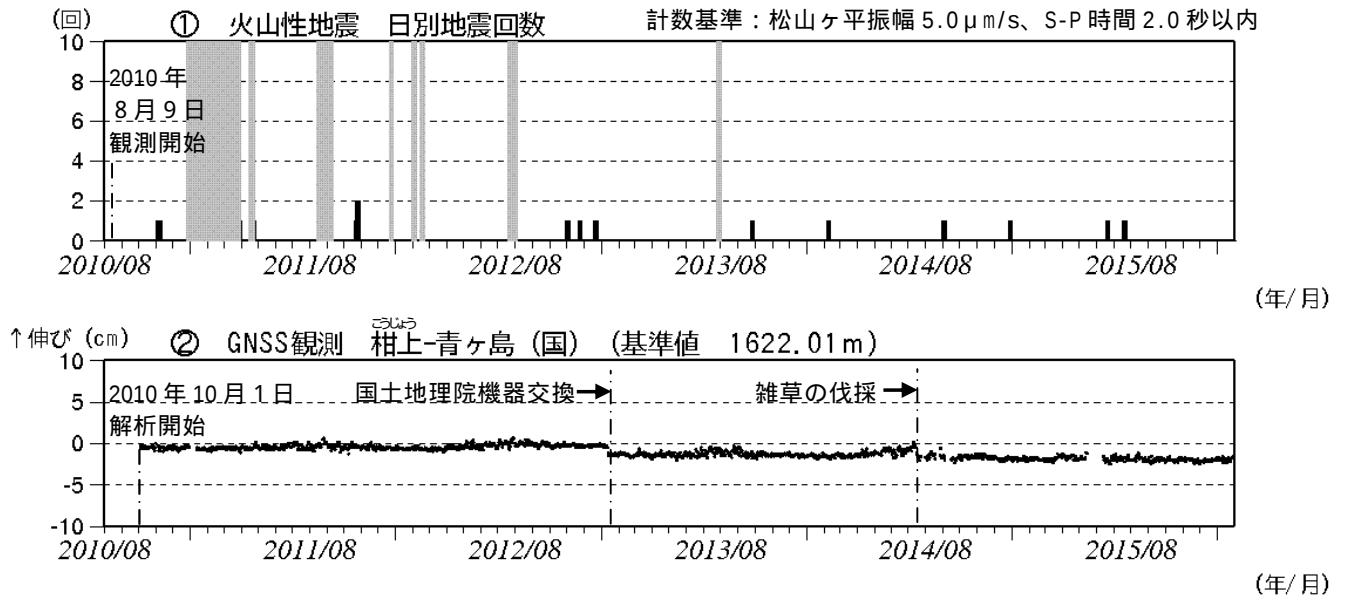
図2 青ヶ島 火山活動経過図（2010年8月9日～2016年1月31日） 青ヶ島周辺の日別地震回数 グラフの灰色部分は機器障害による欠測。 GNSS 連続観測による基線長変化（国）：国土地理院 は図3のGNSS基線に対応。グラフの空白部分は欠測。 ・2014年7月15日に実施した雑草の伐採の影響により、ステップ状の変化がみられます。
