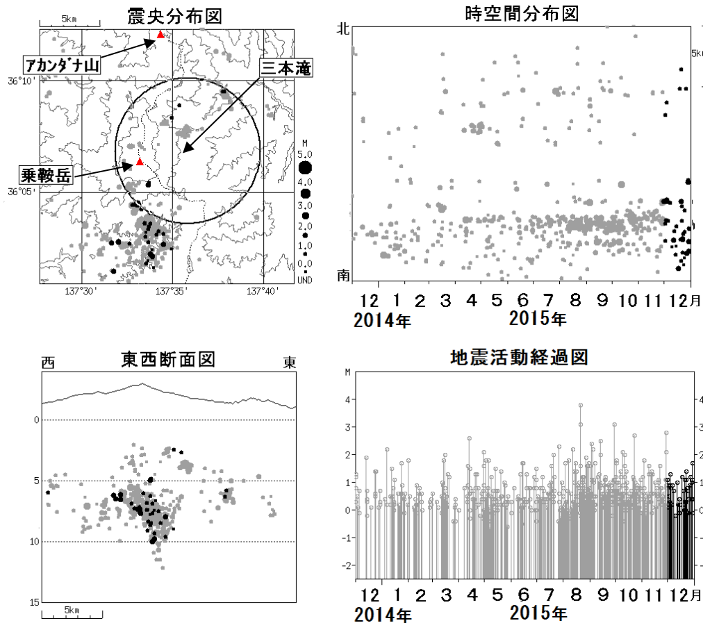
図 3 乗鞍岳 広域地震観測網による山体・周辺の地震活動(2014 年 12 月 1 日～2015 年 12 月 31 日)
