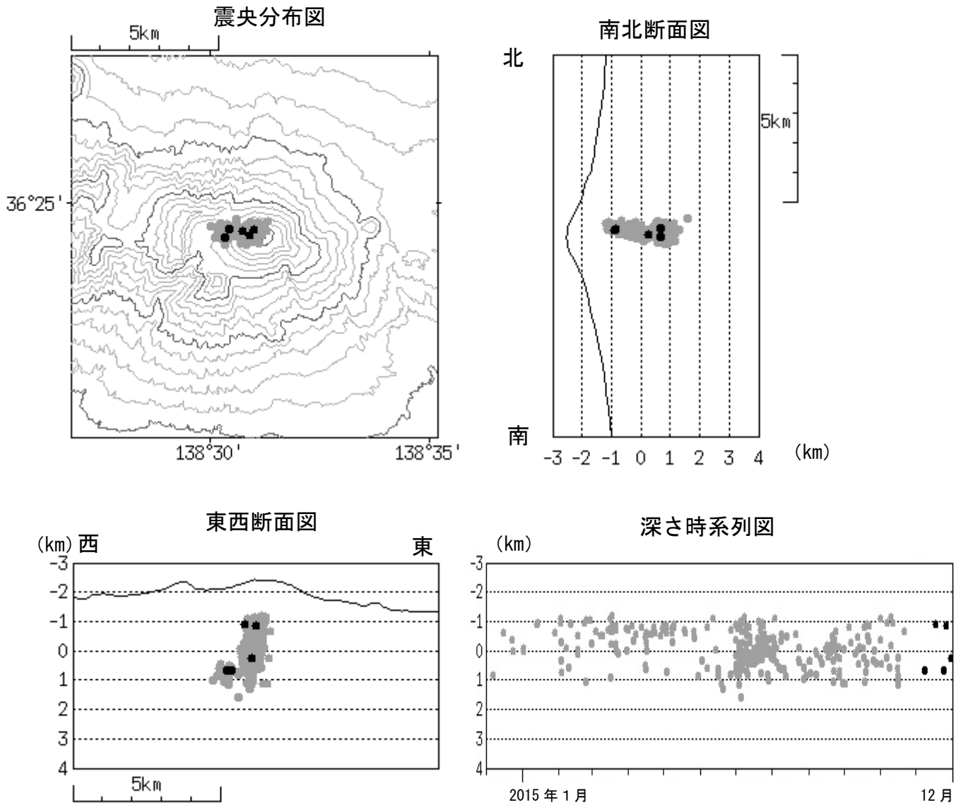
図5 浅間山 震源分布図（2014 年 12 月 1 日～2015 年 12 月 31 日）
