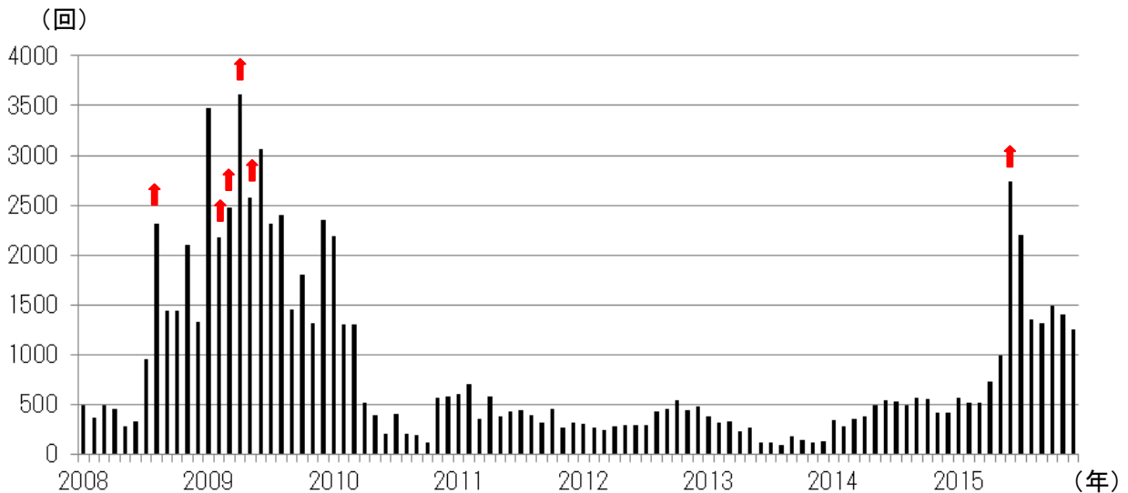
図 7 浅間山 火山性地震の月別回数（2008 年 1 月～2015 年 12 月）
