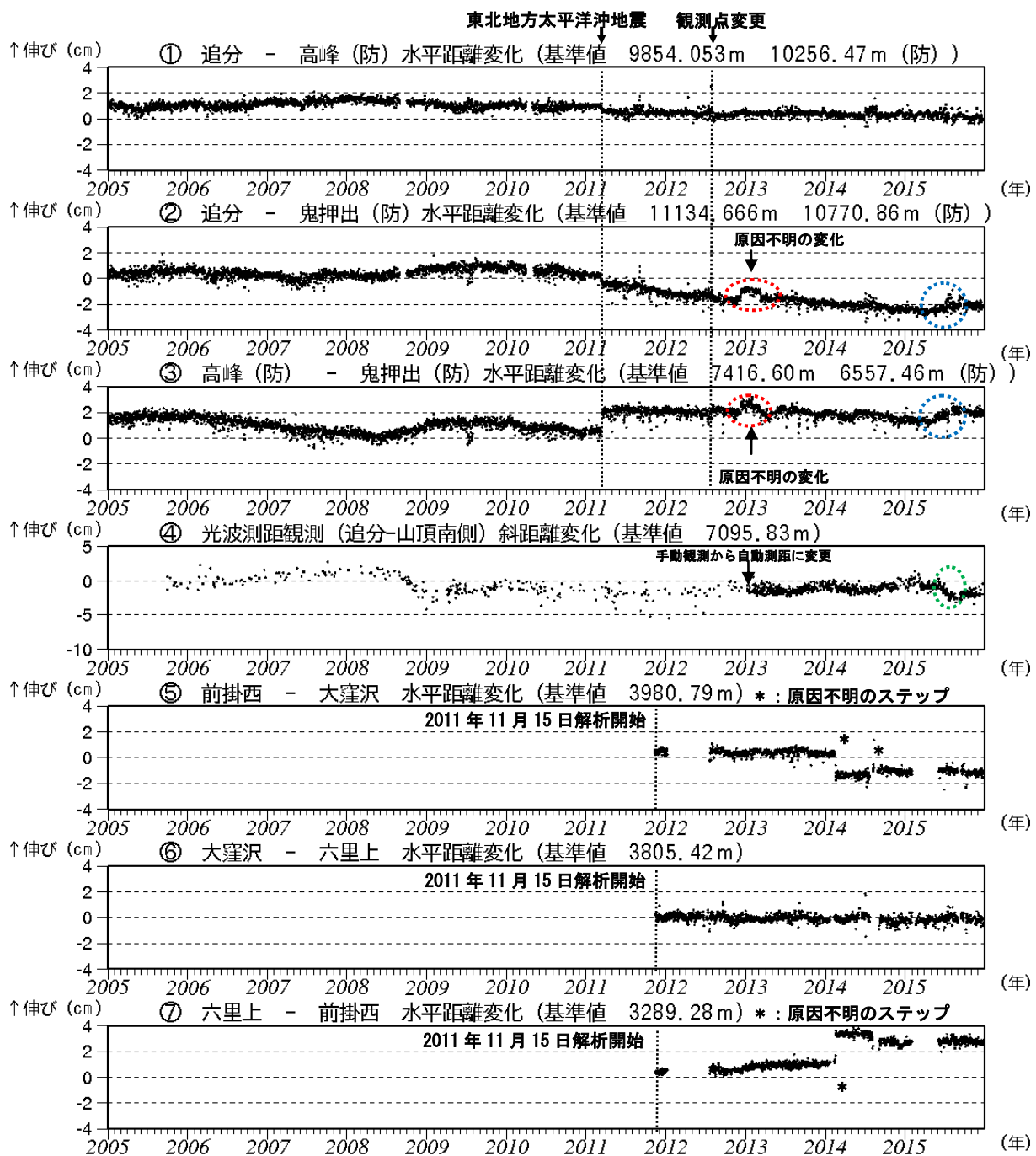
図 8 浅間山 GNSS 連続観測及び光波測距観測の結果 (2005 年 1 月 1 日～2015 年 12 月 31 日)
