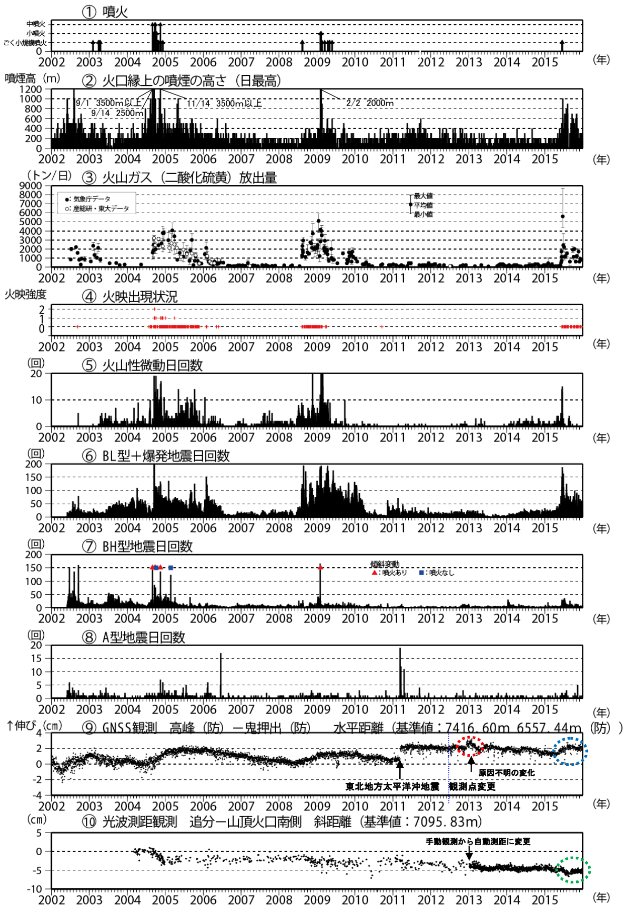
図3 浅間山 火山活動経過図 (2002 年 1 月 1 日～2015 年 12 月 31 日)
