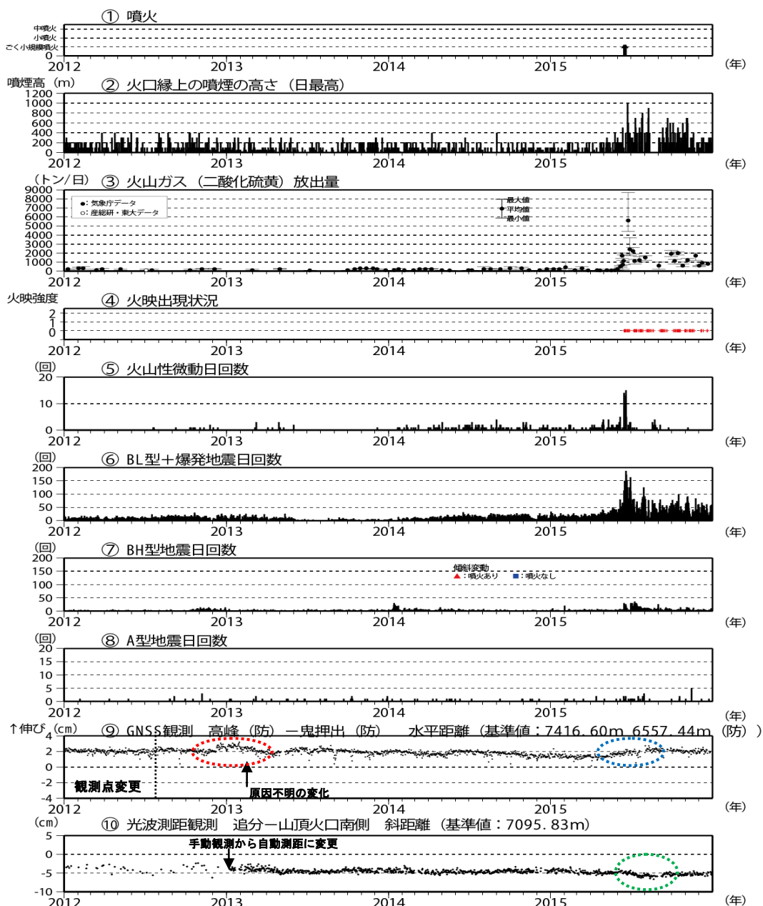
図 4 浅間山 最近の火山活動経過図 (2012 年 1 月 1 日~2015 年 12 月 31 日)
