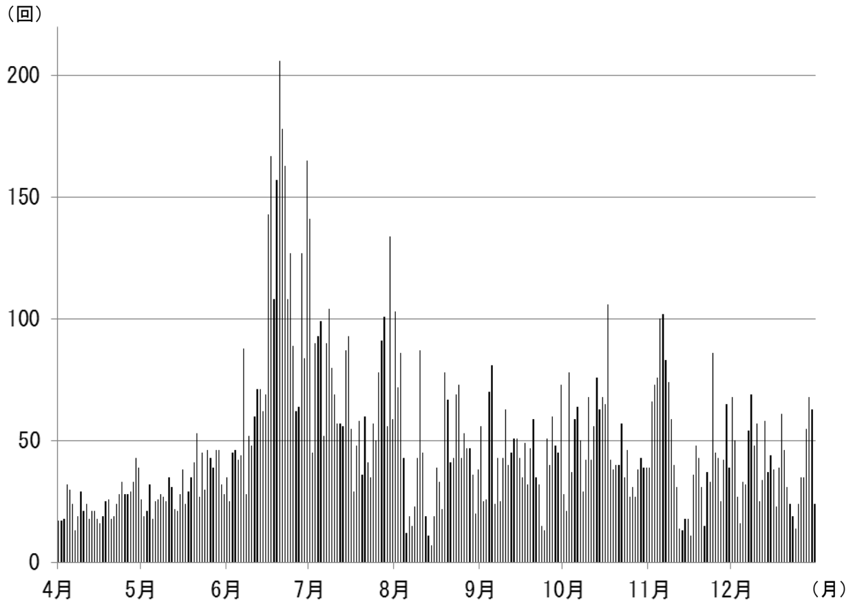
図 6 浅間山 火山性地震の日別回数（2015 年 4 月 1 日～12 月 31 日）
