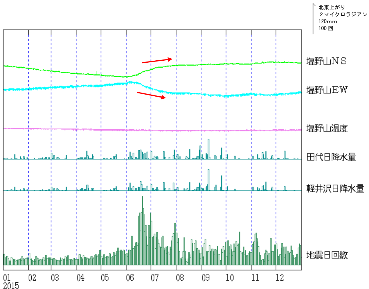
図 10 浅間山 塩野山観測点における傾斜データ（2015 年 1 月 1 日～2015 年 12 月 31 日）
