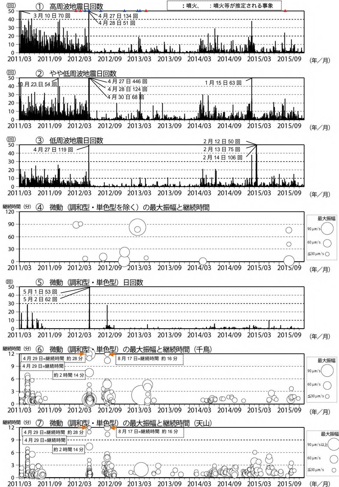
図5 硫黄島 火山活動経過図(2011年3月8日~2015年11月30日)
