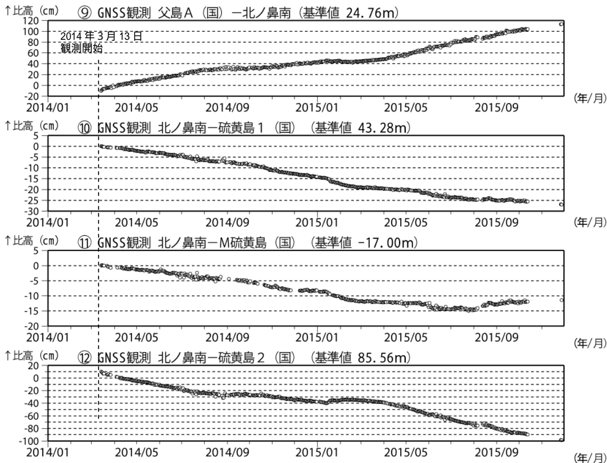
図7 硫黄島 GNSS 観測結果(2014年1月~2015年11月) (国): 国土地理院
