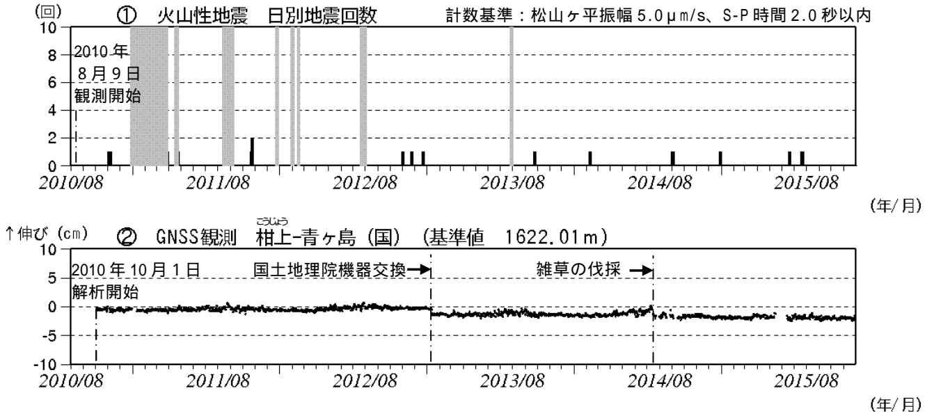
図2 青ヶ島 火山活動経過図（2010年8月9日～2015年11月30日）
