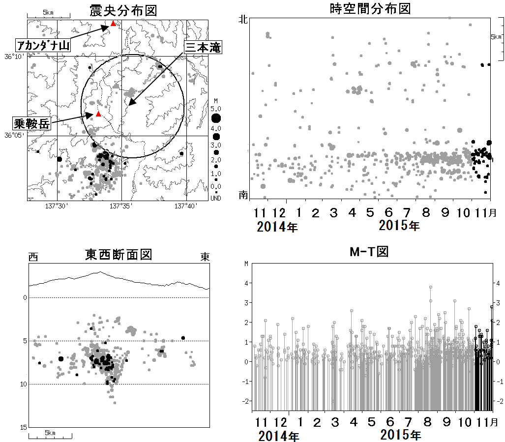
図 3 乗鞍岳 広域地震観測網による山体・周辺の地震活動(2014 年 11 月 1 日～2015 年 11 月 30 日)
