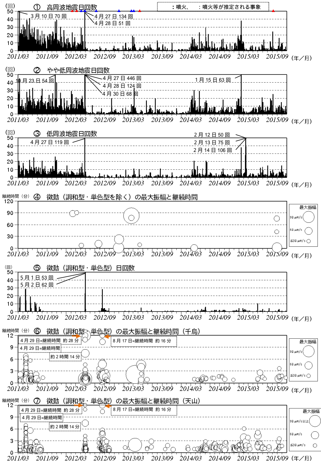
図5 硫黄島 火山活動経過図(2011年3月8日~2015年10月31日)
