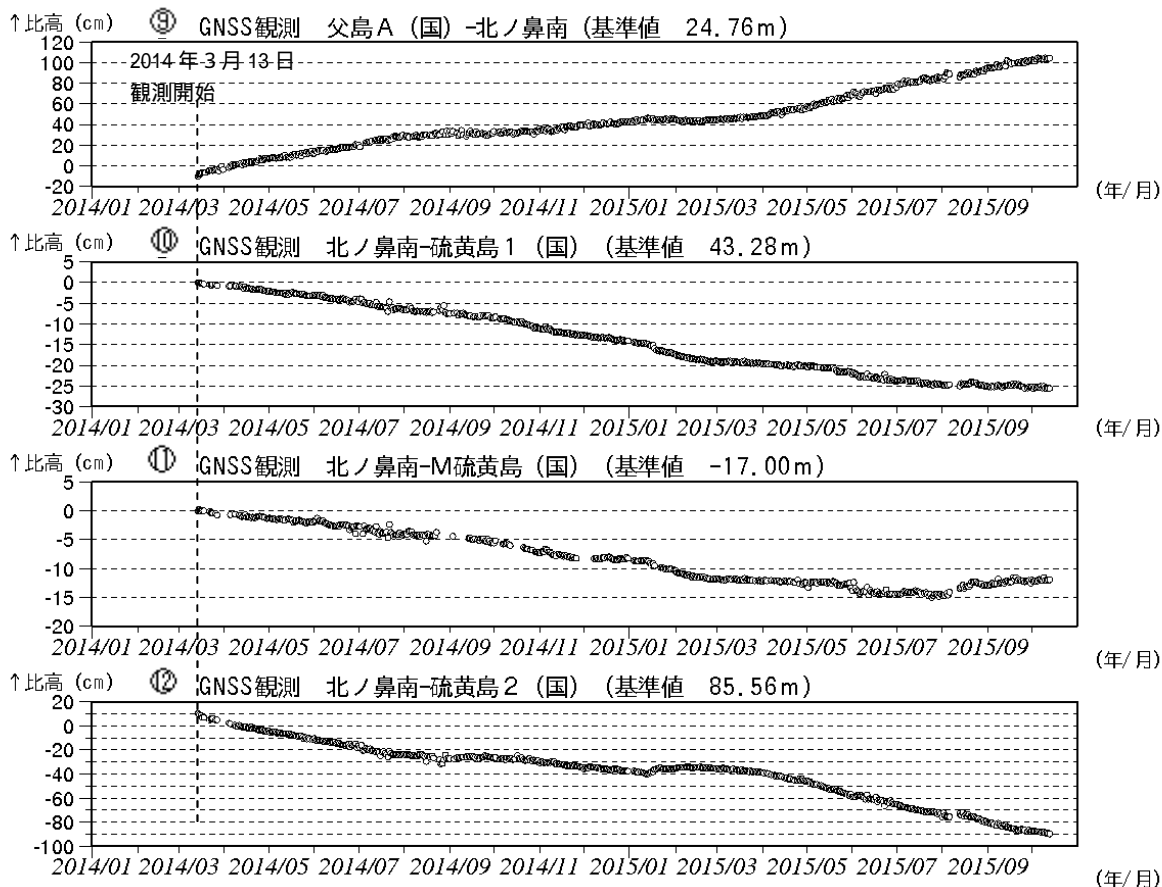
図7 硫黄島 GNSS 観測結果(2014年1月~2015年10月) (国): 国土地理院
