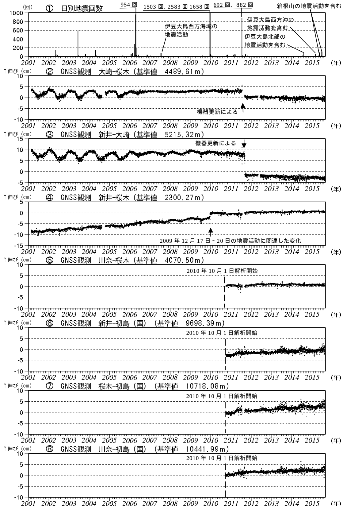
図3 伊豆東部火山群 火山活動経過図（2001年1月1日～2015年8月31日）
