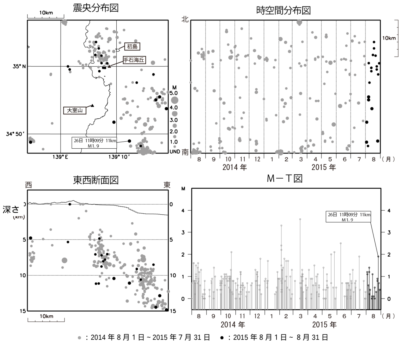
図 2 伊豆東部火山群 広域地震観測網による震源分布図（2014 年 8 月 1 日～2015 年 8 月 31 日）
