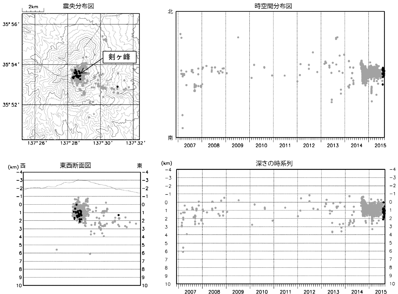
図2 御嶽山 震源分布図（2006 年 12 月 1 日～2015 年 8 月 31 日）
