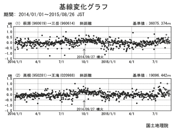
図 6 御嶽山 国土地理院による GNSS 基線変化グラフ 4)
