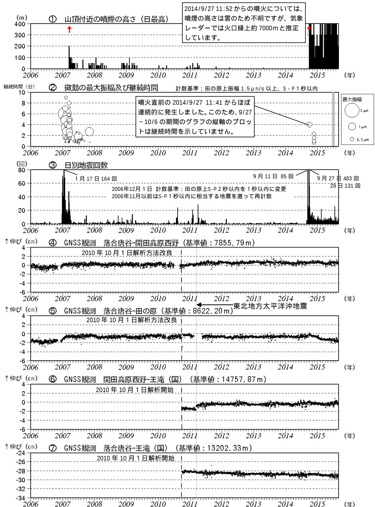
図 4 御嶽山 長期間の火山活動経過図（2006 年 1 月 1 日～2015 年 8 月 31 日）
