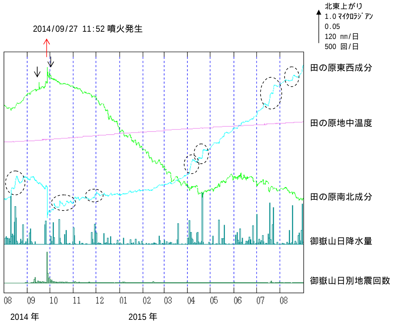
図5 御嶽山 田の原観測点（剣ヶ峰山頂の南東約3 km）の傾斜変動 （2014年8月1日～2015年8月31日）
