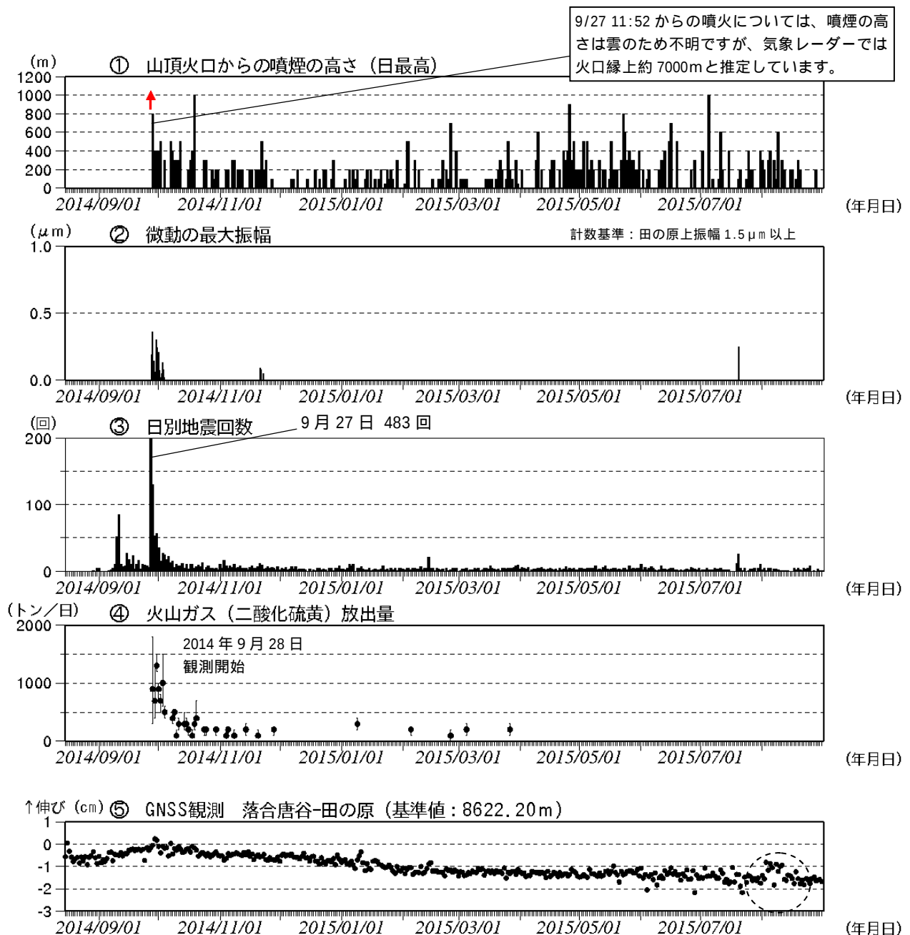
図 3 御嶽山 最近の火山活動経過図（2014 年 8 月 15 日～2015 年 8 月 31 日）
