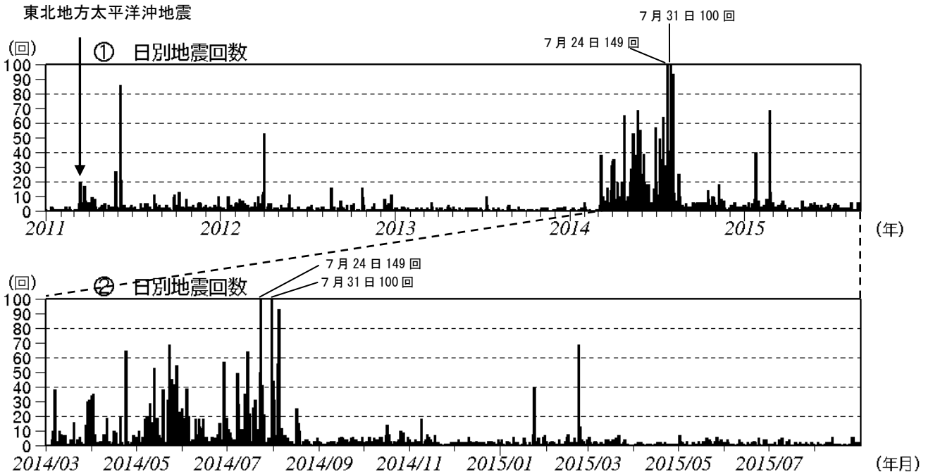
図2 草津白根山 日別地震回数 (2011年1月1日～2015年8月31日)
