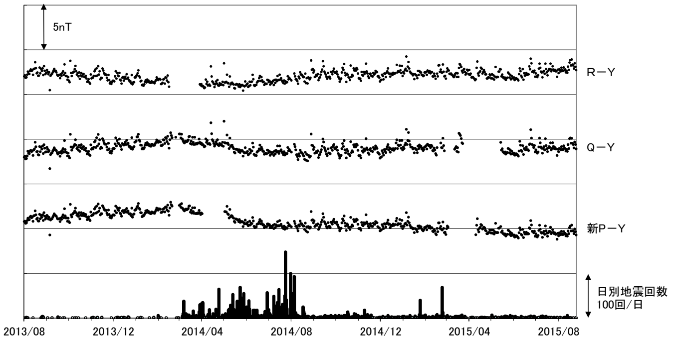
図7 草津白根山 全磁力連続観測による全磁力値の変化及び日別地震回数（2013年8月～2015年8月25日） 連続観測点P、Q、Rおよび新Pにおける八ヶ岳地球電磁気観測所（東京大学）（Y）との全磁力の夜間日平均 値差。最下段は草津白根山で観測された日別地震回数を示しています。 全磁力連続観測で、2014年5月頃からみられていた湯釜近傍地下の温度上昇を示すと考えられる変化は、 2014年7月以降停滞しています。グラフの空白部分は欠測を示します。
