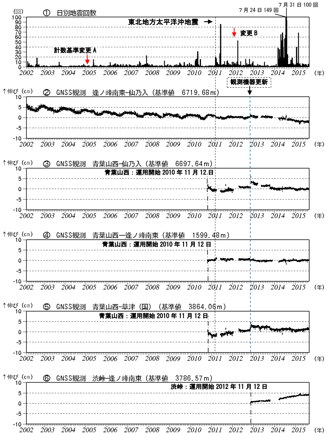
図3 草津白根山 火山活動経過図（2002年1月1日～2015年8月31日）
