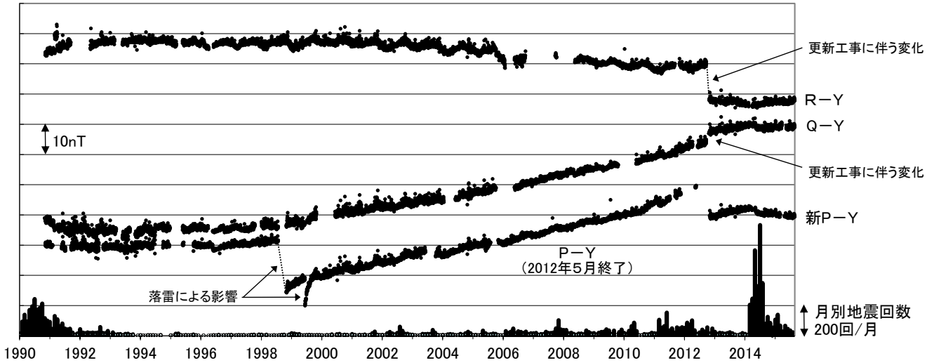
図6 草津白根山 全磁力連続観測による全磁力値の変化及び月別地震回数（1990年～2015年8月25日） 連続観測点P、Q、Rおよび新Pにおける八ヶ岳地球電磁気観測所（東京大学）（Y）との全磁力の夜間日 平均値差。最下段は草津白根山で観測された月別地震回数を示しています。全磁力連続観測で、2014 年5月頃からみられていた湯釜近傍地下の温度上昇を示すと考えられる変化は、2014年7月以降停 滞しています。グラフの空白部分は欠測を示します。
