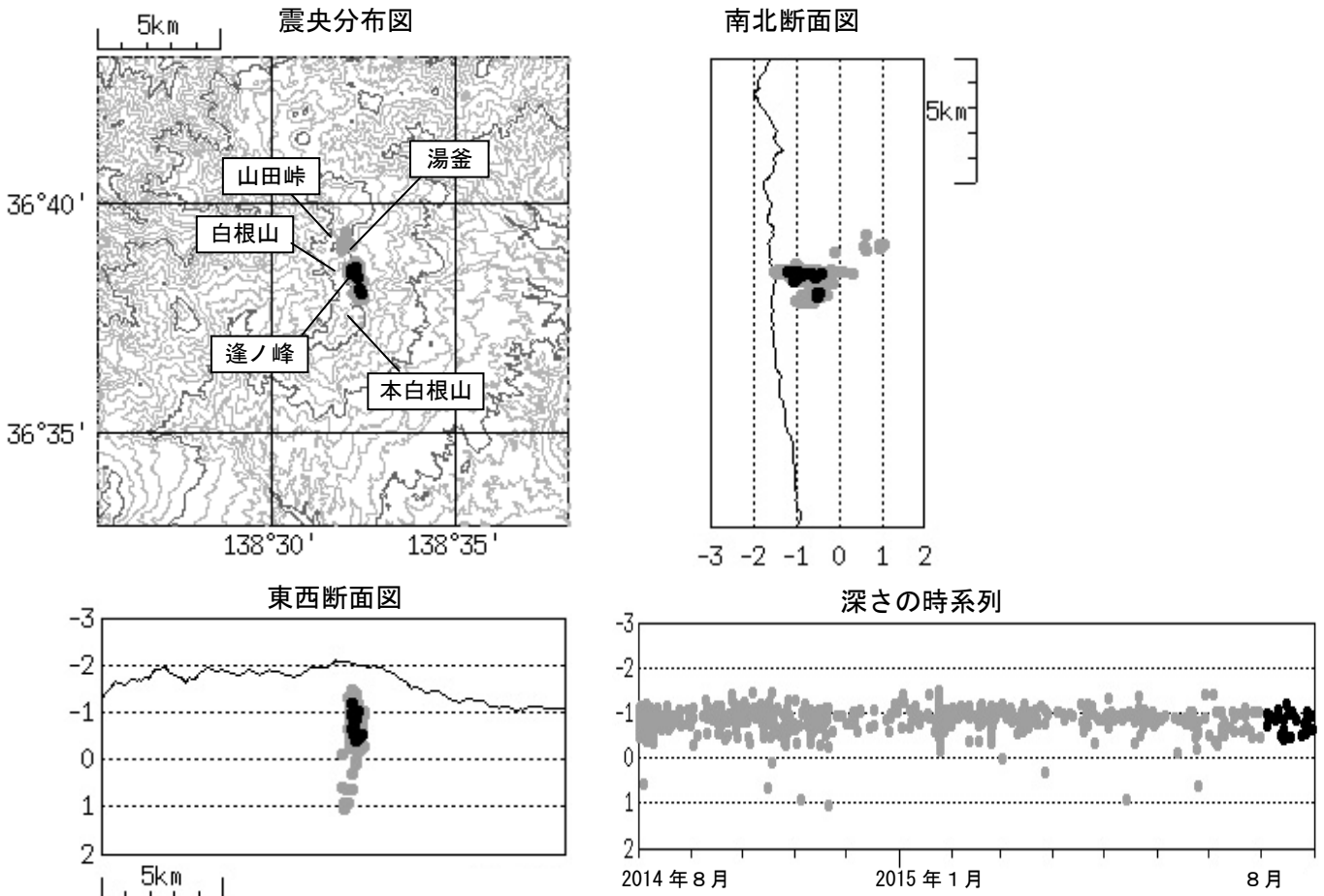
図1 草津白根山 震源分布図 (2014年8月1日～2015年8月31日) ● : 2014年8月1日～2015年7月31日 ● : 2015年8月1日～8月31日
