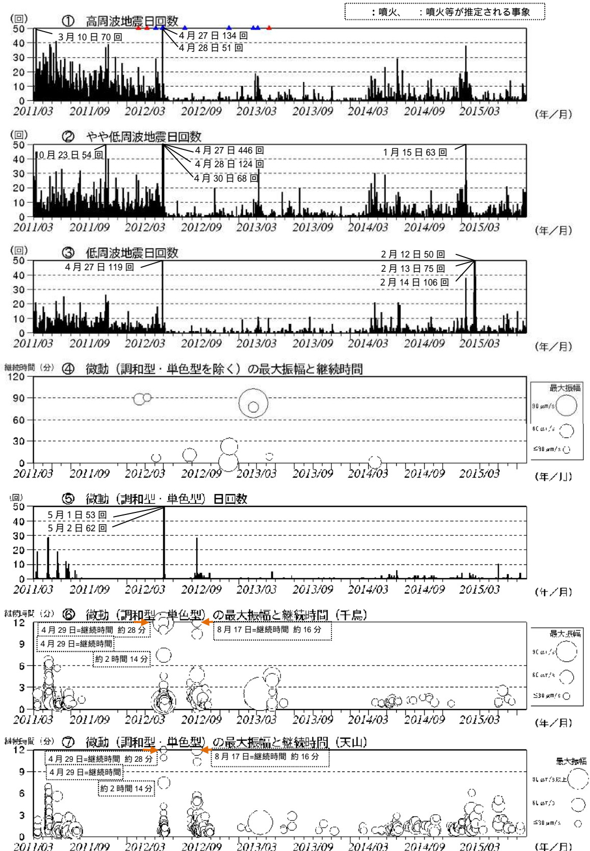
図5 硫黄島 火山活動経過図(2011年3月8日~2015年7月31日)
