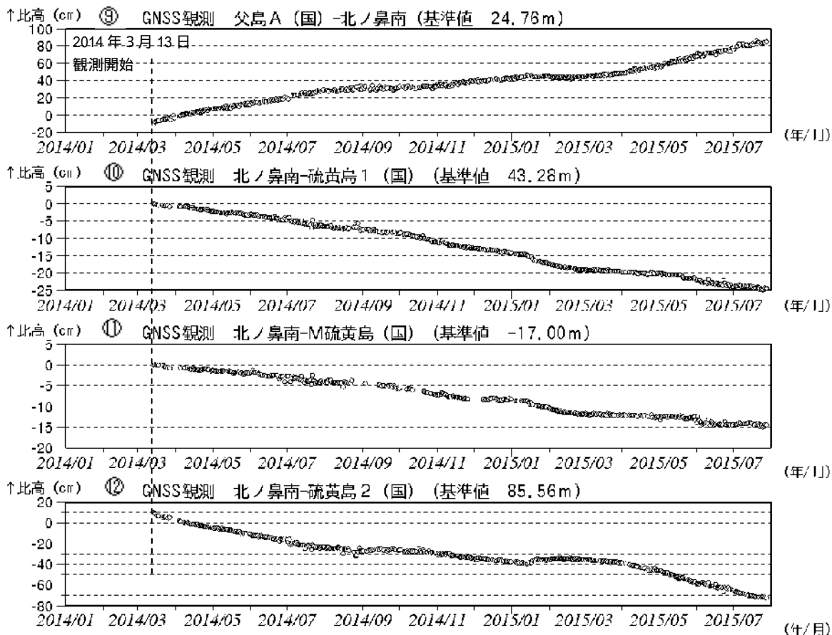
図7 硫黄島 GNSS 1) 観測結果(2014年1月~2015年7月) (国): 国土地理院
