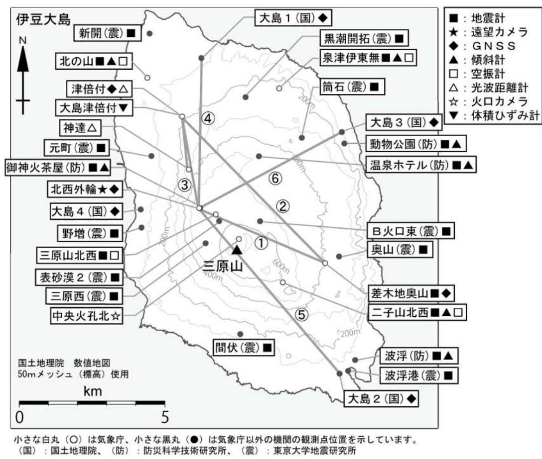
図 8 伊豆大島 観測点配置図
