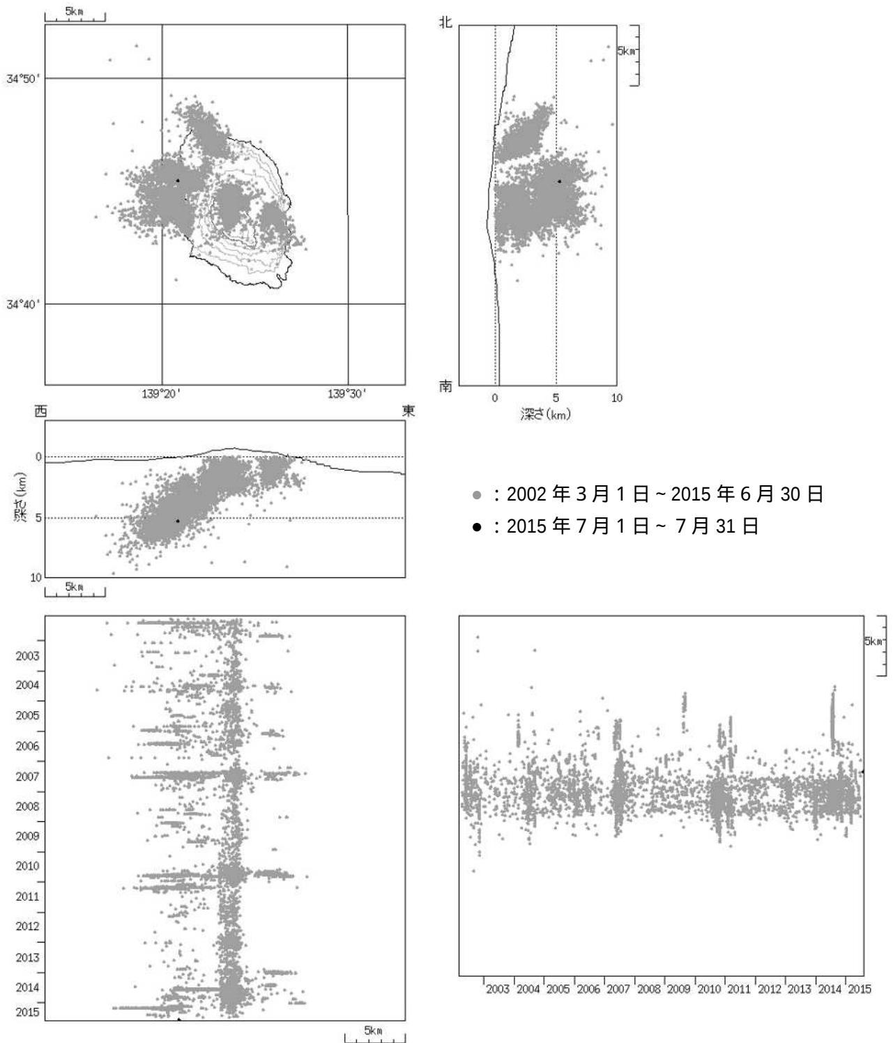
図4 伊豆大島 震源分布図（2002 年 3 月 1 日～2015 年 7 月 31 日）
