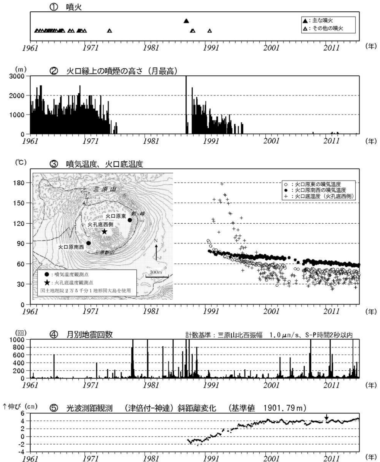
図 1 伊豆大島 長期間の火山活動経過図（1961 年 1 月～2015 年 7 月 31 日）
