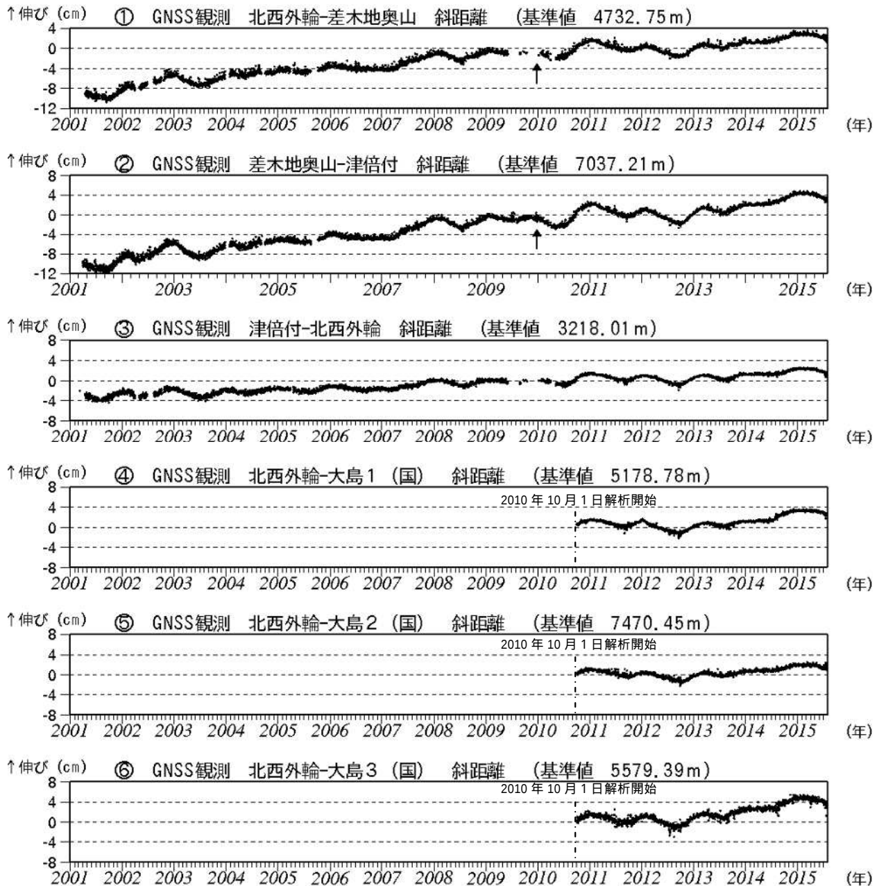
図3 伊豆大島 GNSS連続観測による基線長変化(2001年1月～2015年7月31日)(国): 国土地理院 2010年10月以降のデータについては、電離層の影響を補正する等、解析方法を改良しています。 ～ は図8のGNSS基線 ～ に対応しています。 グラフの空白部分は欠測。 の矢印は差木地奥山支柱工事を実施。
