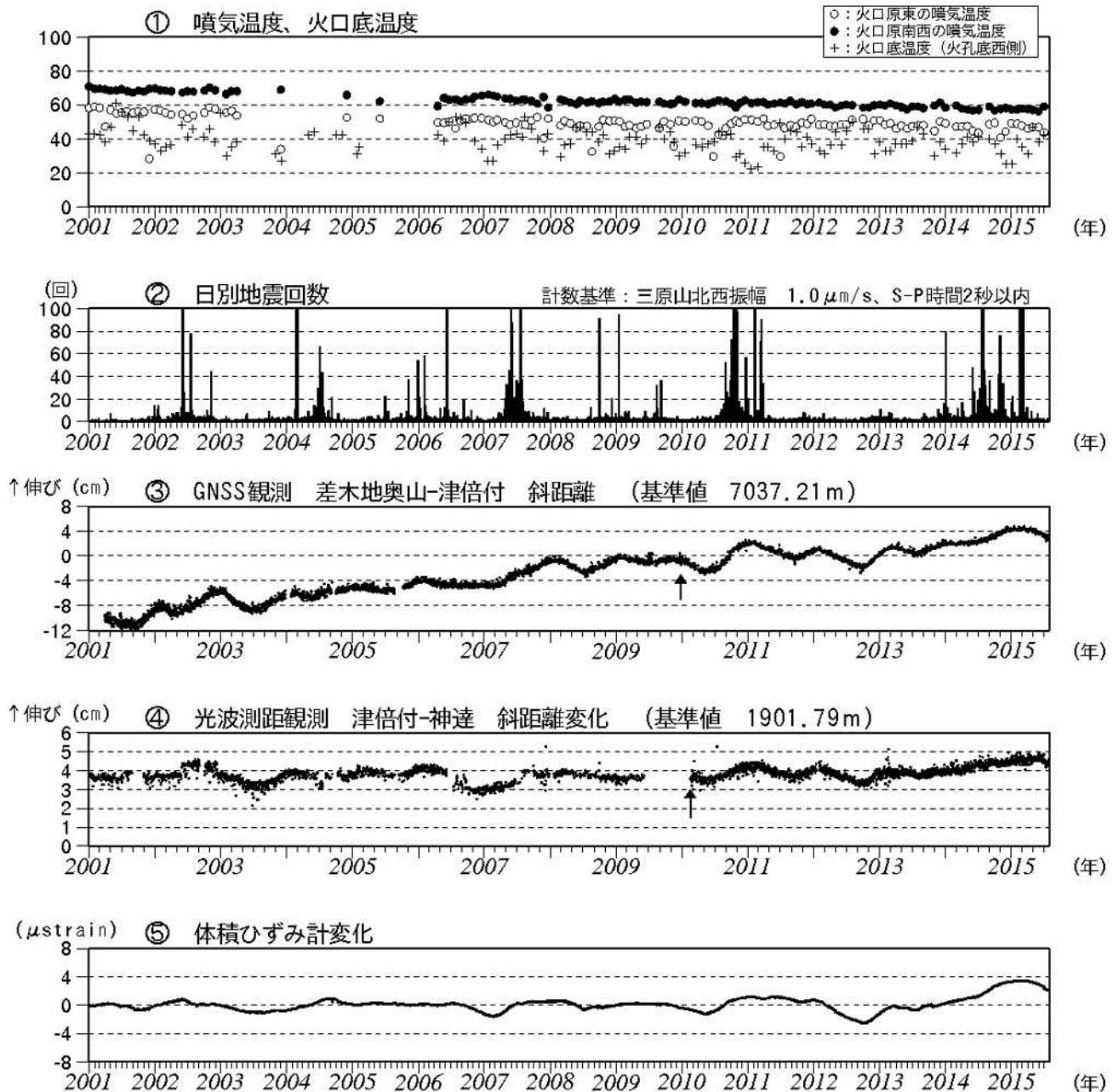
図2 伊豆大島 最近の火山活動経過図（2001年1月～2015年7月31日）
