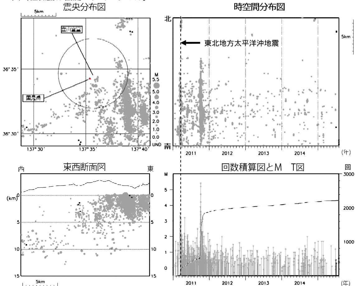
図 1 弥陀ヶ原 広域地震観測網による山体・周辺の地震活動（2011 年 1 月 1 日～2015 年 7 月 31 日）
