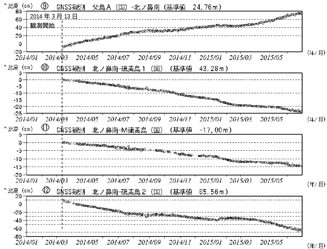
図7 硫黄島 GNSS 1) 観測結果(2014年1月~2015年6月) (国): 国土地理院
