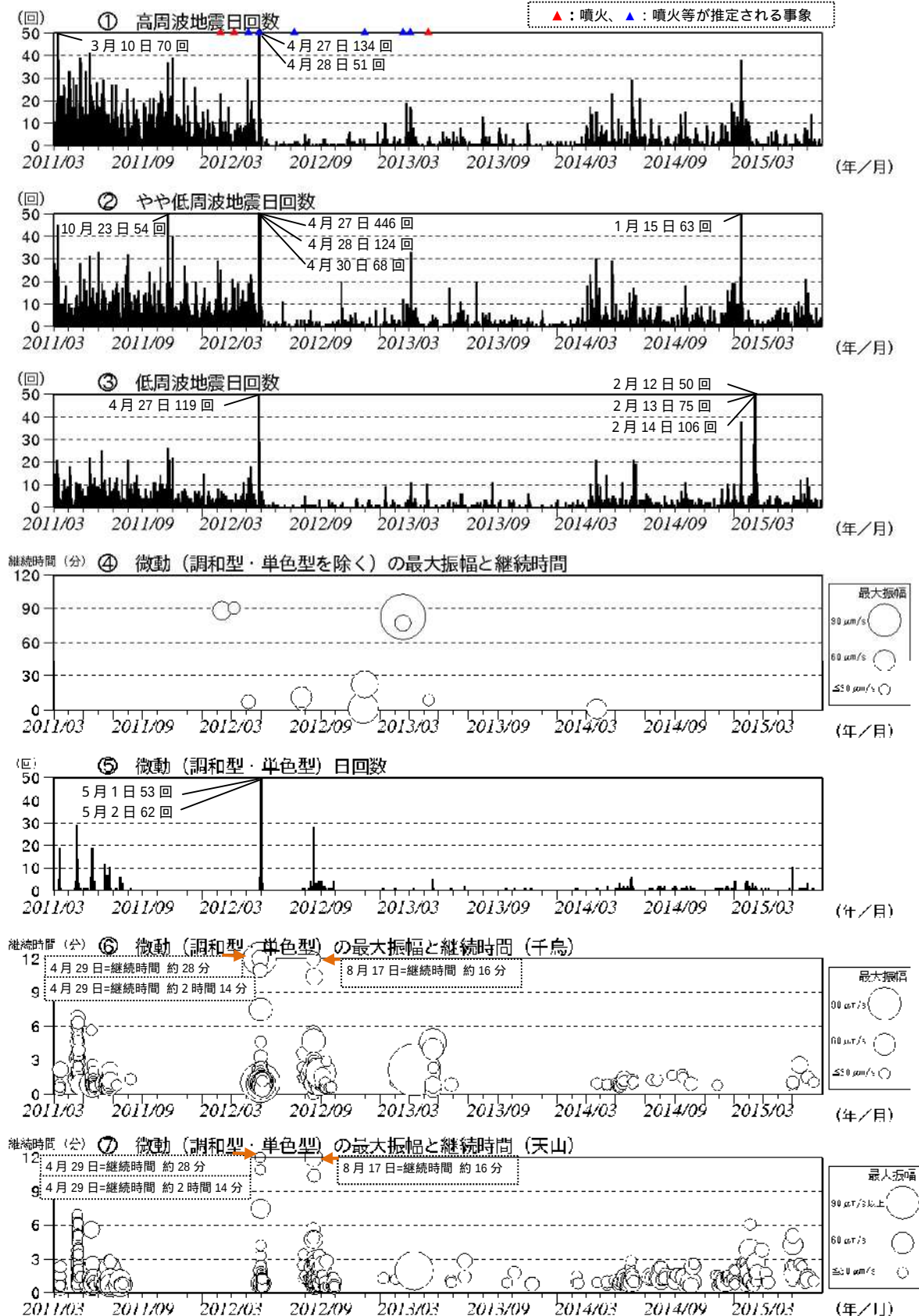
図5 硫黄島 火山活動経過図（2011年3月8日～2015年6月30日）
