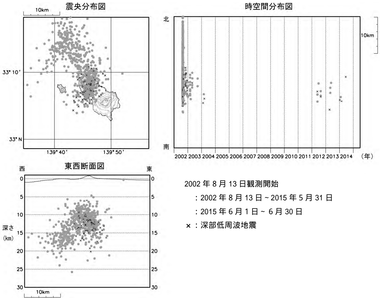
図3 八丈島 震源分布図(2002年8月13日~2015年6月30日) 今期間、八丈島付近に震源が決定された高周波地震及び深部低周波地震はありませんでした。
