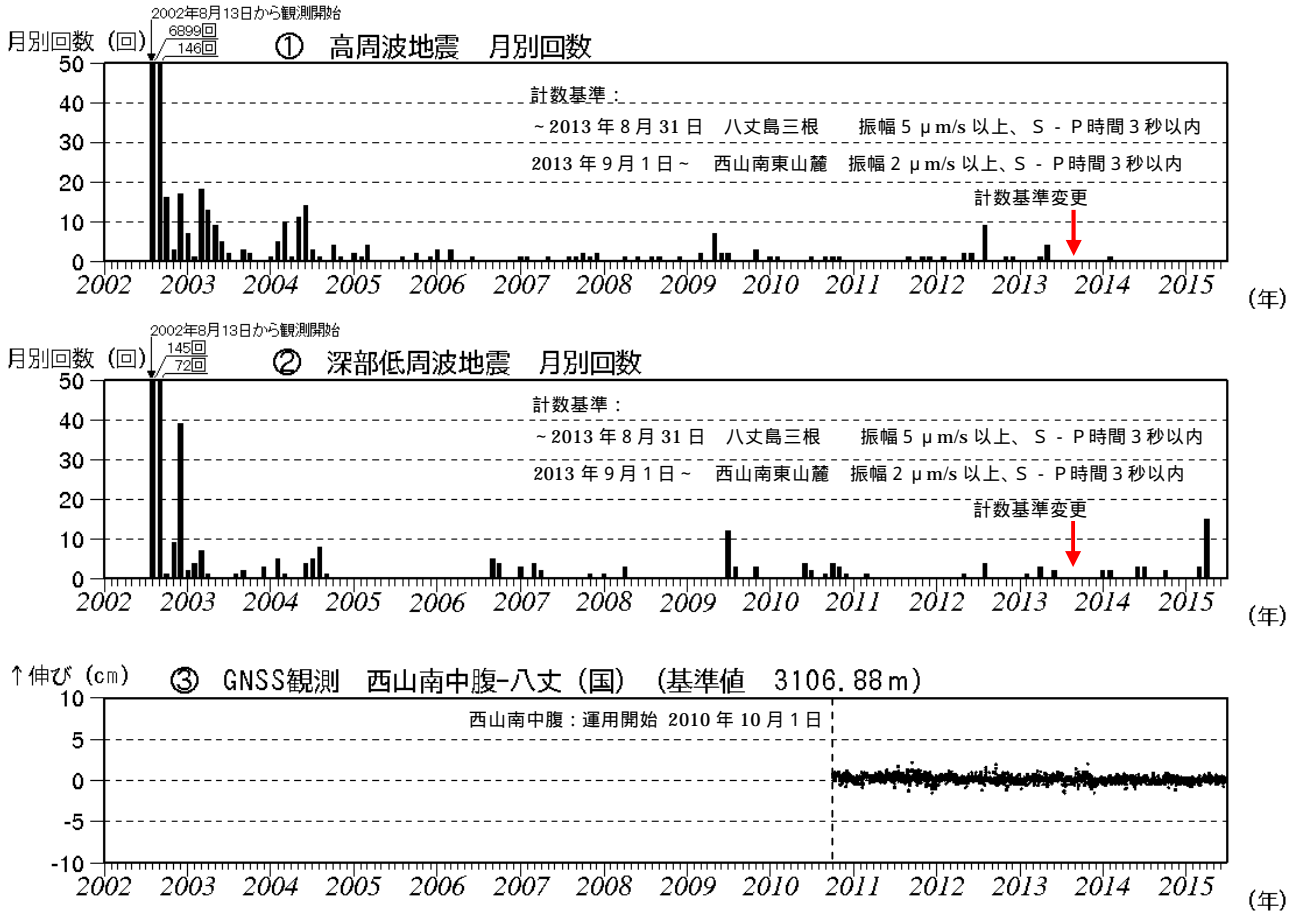
図2 八丈島 火山活動経過図(2002年8月13日~2015年6月30日)
