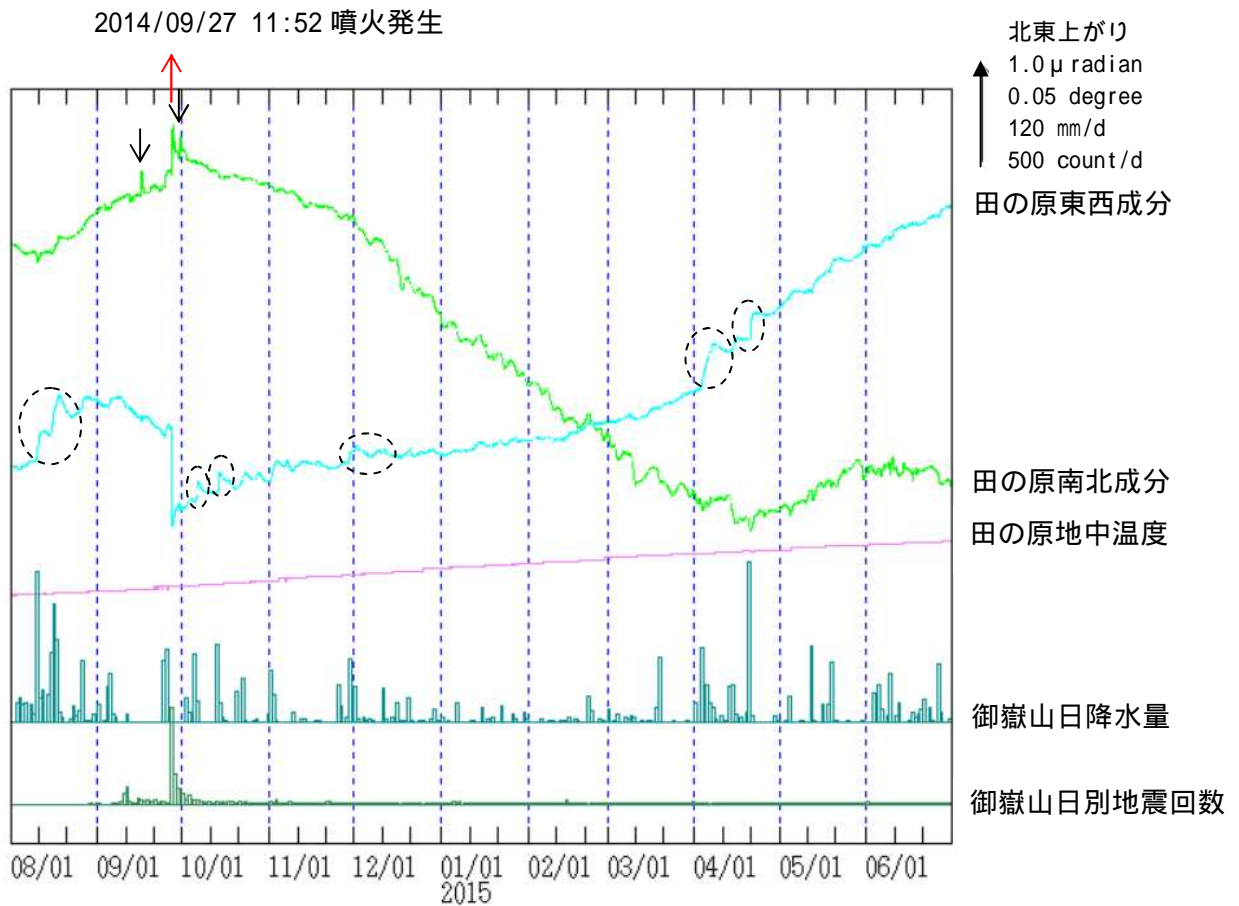
図6 御嶽山 田の原観測点(剣ヶ峰山頂の南東約3 km)の傾斜変動 (2014年8月1日~2015年6月30日)
