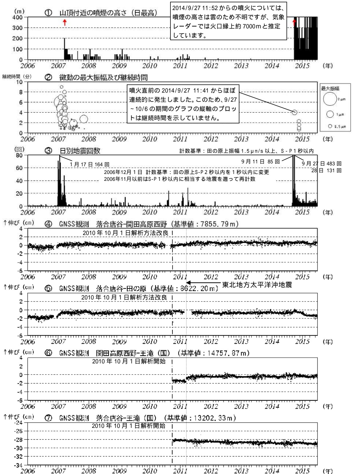
図5 御嶽山 長期間の火山活動経過図(2006年1月1日~2015年6月30日)
