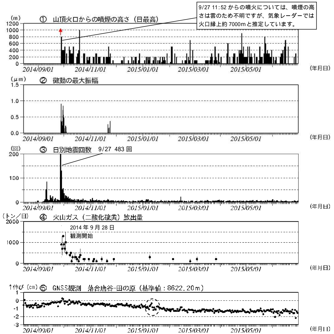
図4 御嶽山 最近の火山活動経過図(2014年8月15日~2015年5月31日)
