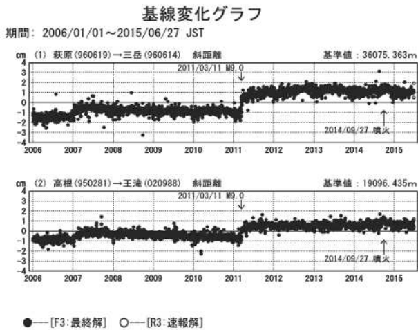
図7 御嶽山 国土地理院によるGNSS基線変化グラフ 5)
