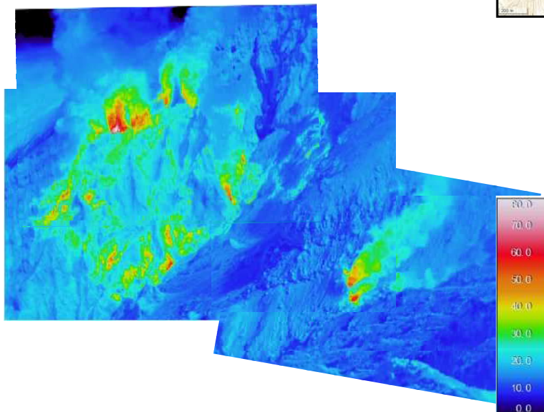
図 2 御嶽山 山頂付近の状況及び地表面温度分布（2015 年 6 月 10 日 10 時 50 分奥の院から撮影） 上図：可視画像、下図：温度分布 2)
