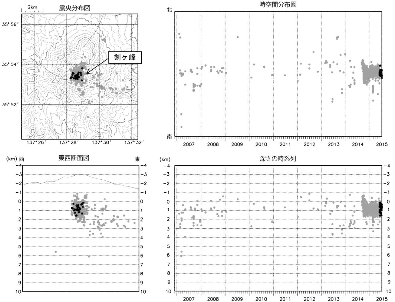
図3 御嶽山 震源分布図(2006年12月1日~2015年6月30日)
