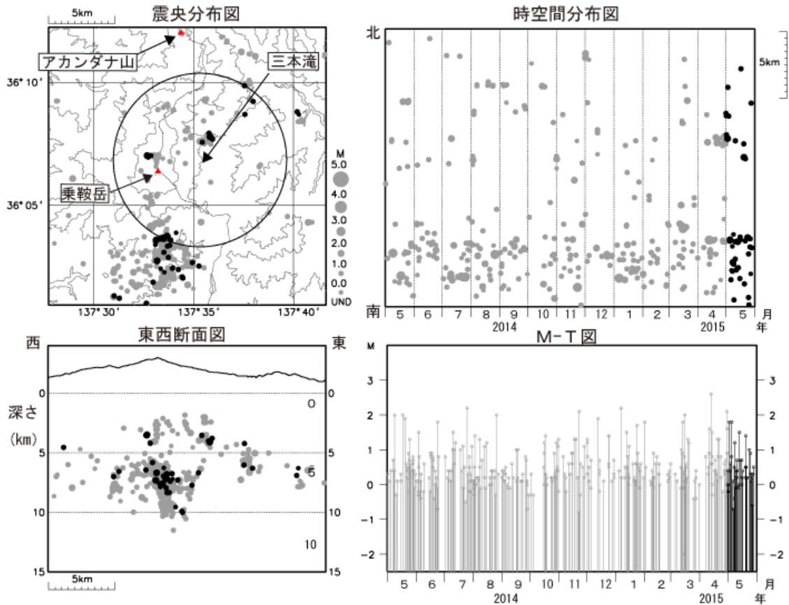
図3 乗鞍岳 広域地震観測網による山体・周辺の地震活動(2014年5月1日～2015年5月31日)
