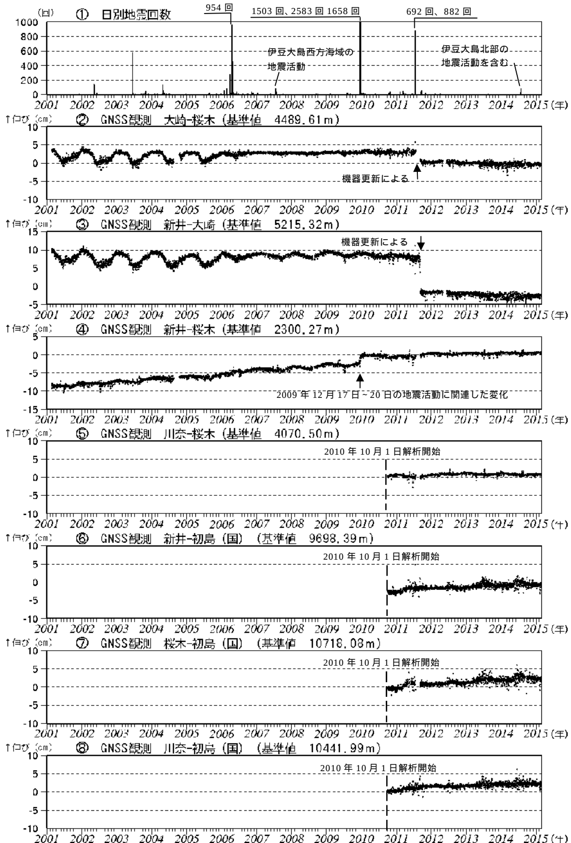
図3 伊豆東部火山群 火山活動経過図（2001年1月1日～2015年2月28日）
