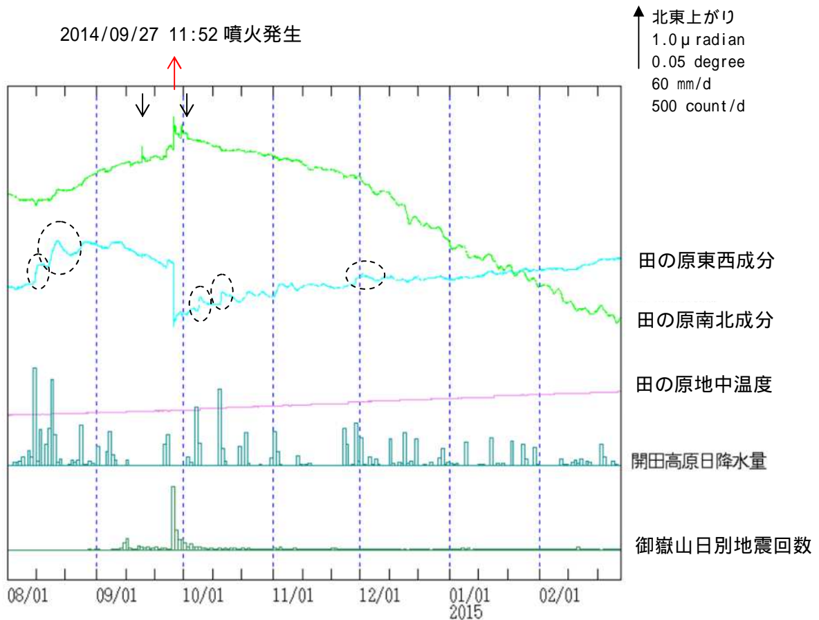
図5 御嶽山 田の原観測点(剣ヶ峰山頂の南東約3 km)の傾斜変動 (2014年8月1日~2015年2月28日)
