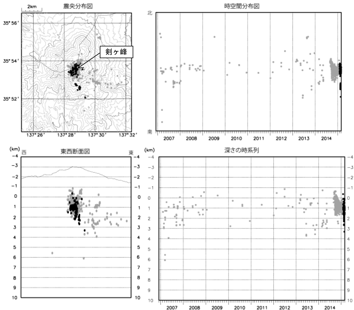
図 2 御嶽山 震源分布図（2006 年 12 月 1 日～2015 年 2 月 28 日）
