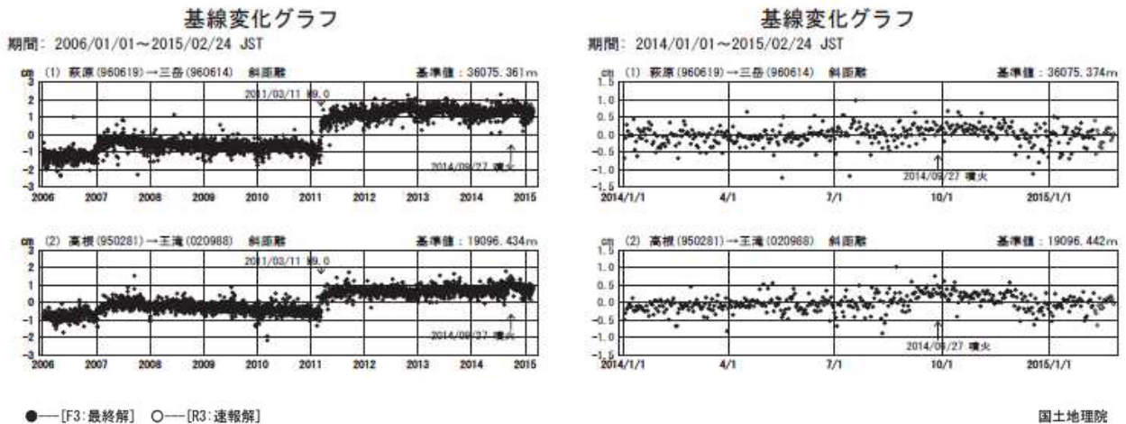
図 6 御嶽山 国土地理院による GNSS 基線変化グラフ 3)
