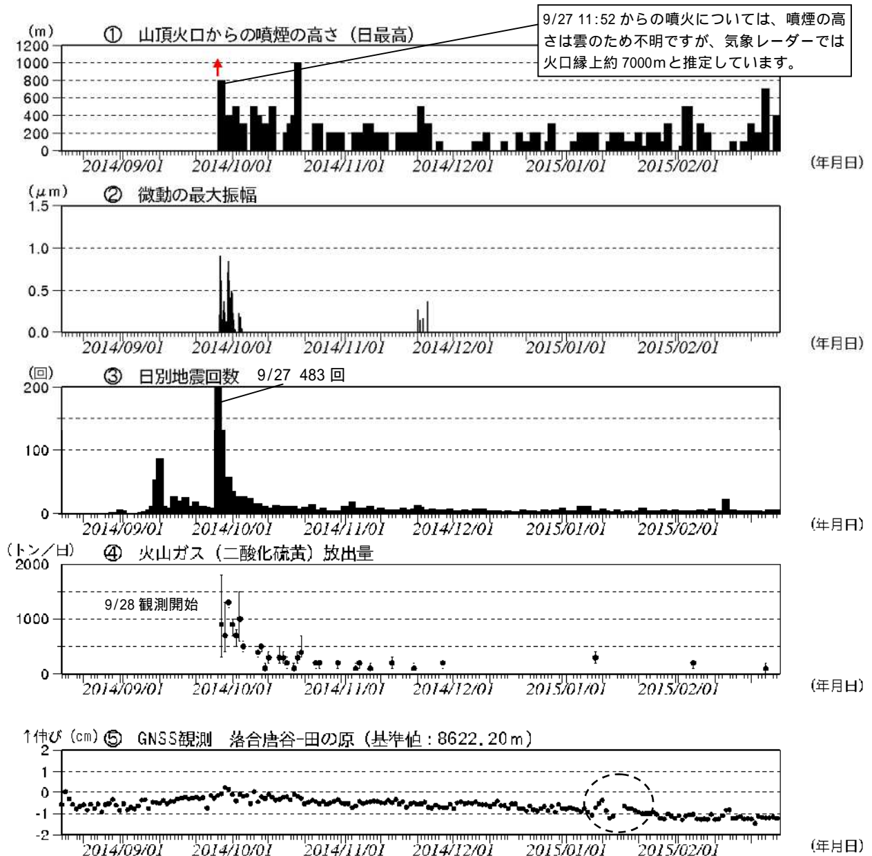
図3 御嶽山 最近の火山活動経過図(2014年8月15日~2015年2月28日)
