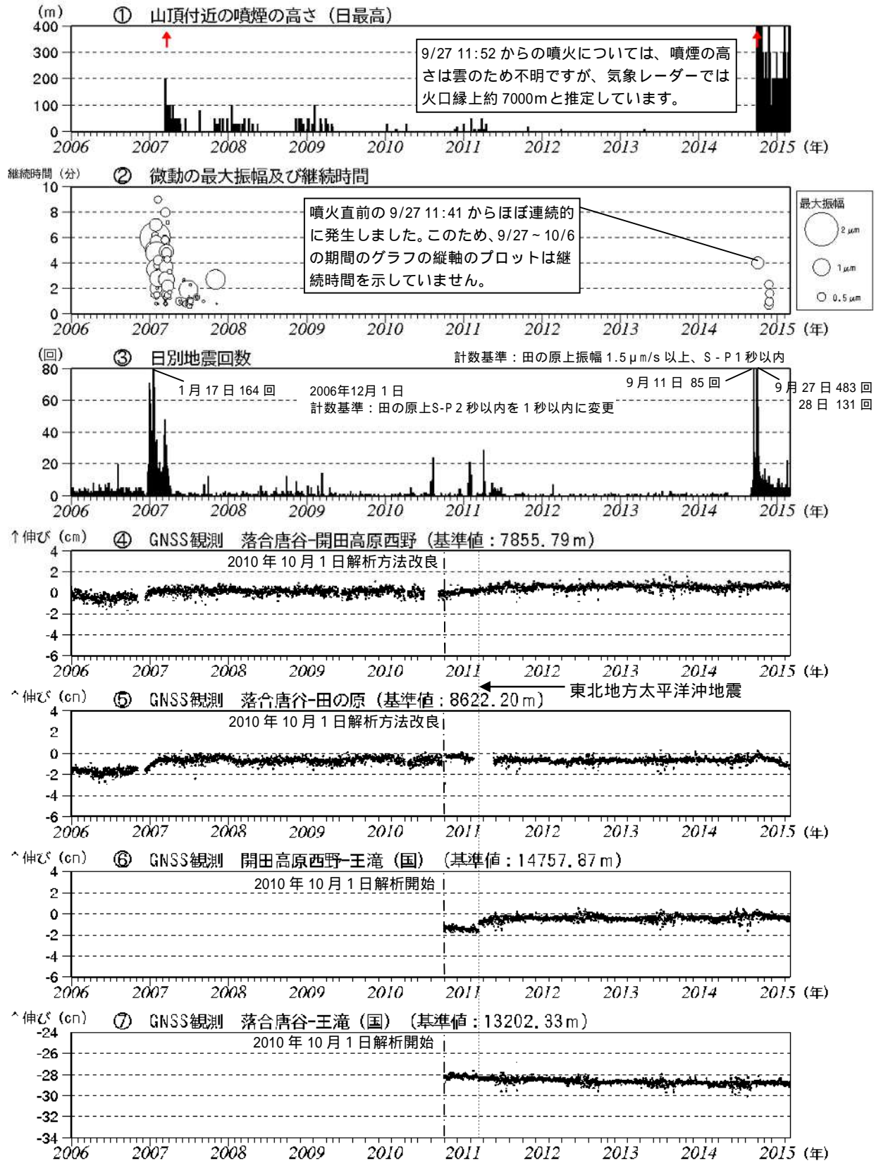
図4 御嶽山 長期間の火山活動経過図(2006年1月1日~2015年2月28日) 遠望カメラによる噴煙の高さ 噴煙の高さは日最大値(噴火時以外は定時観測(09時・15時)の値)。矢印は噴火開始を示します。 ~ GNSS連続観測による基線長変化(国):国土地理院 には東北地方太平洋沖地震(2011年3月11日)に伴うステップ状の変化がみられます。2010年10月以降のデータについては、電離層の影響を補正する等、解析方法を改良しています。図中 ~ は図8のGNSS基線 ~ に対応します。グラフの空白部分は欠測を示します。
